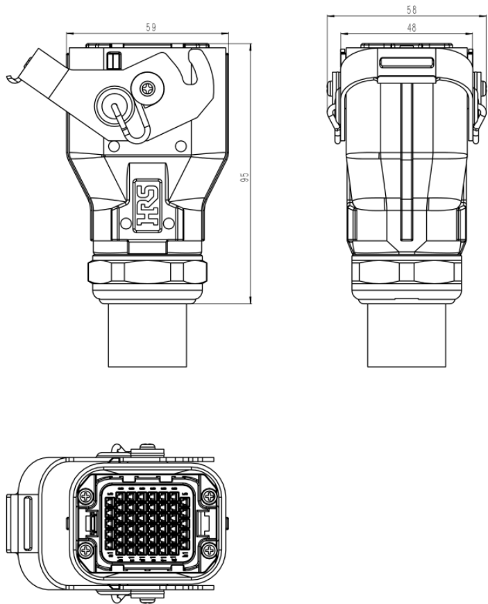
图 9-2 inCube20/inCube2S/inCube20-HP/ARC5-12 重载接头尺寸
