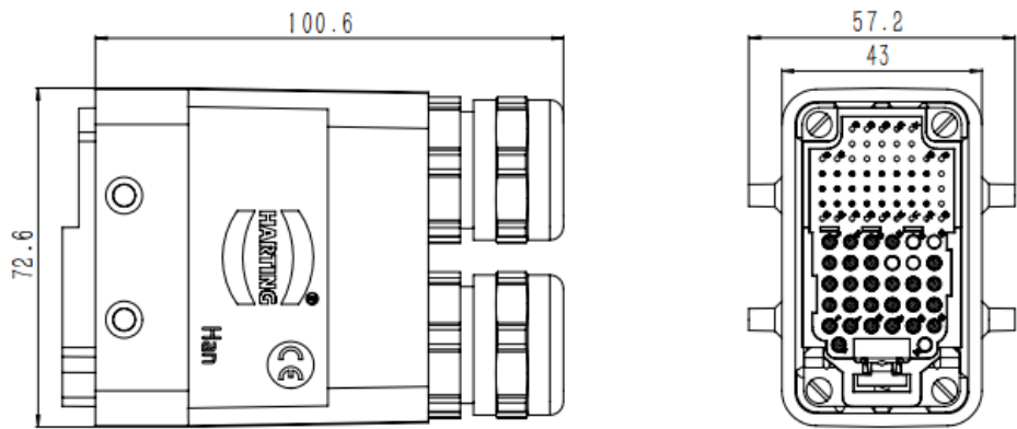
图 9-4 inCube20T/inCube20T-HP/ARC5-12T 重载插头尺寸图
