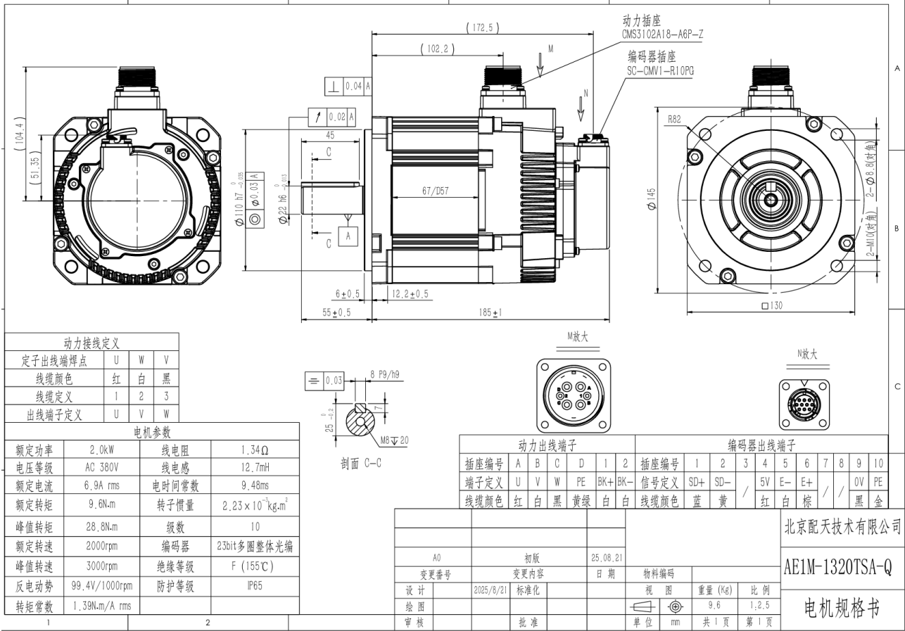
图 28-15 AE1M-1320TSA-Q 电机图纸
