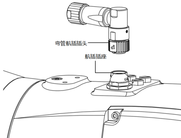
图 1-4 步骤 2 图示
