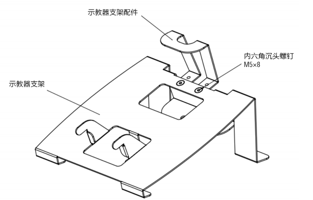
图 26-4 示教器固定装置示意图
