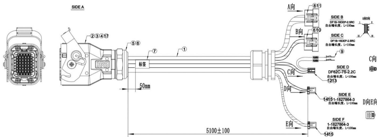
图 9-29 inCube2S-20 拖链重载线示意图
