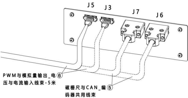
图 21-8 MCBS-IEB 正面示意图
