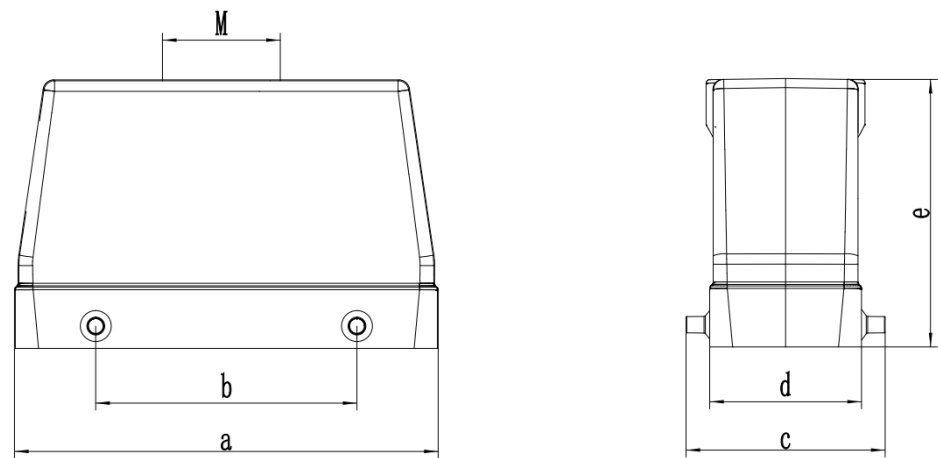
图 9-13 动力线重载接头尺寸
