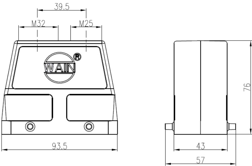
图 9-24 inCube22 重载接头尺寸
