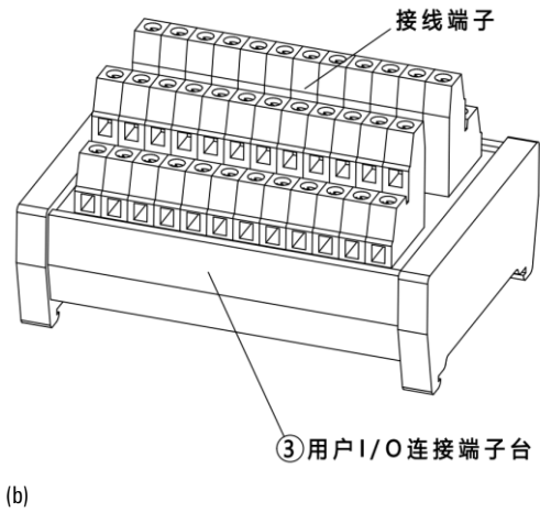
图 5-1 基座上 I/O 线束连接示意图
