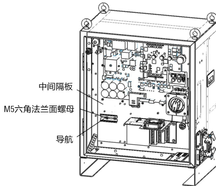
图 16-6 安装导轨
