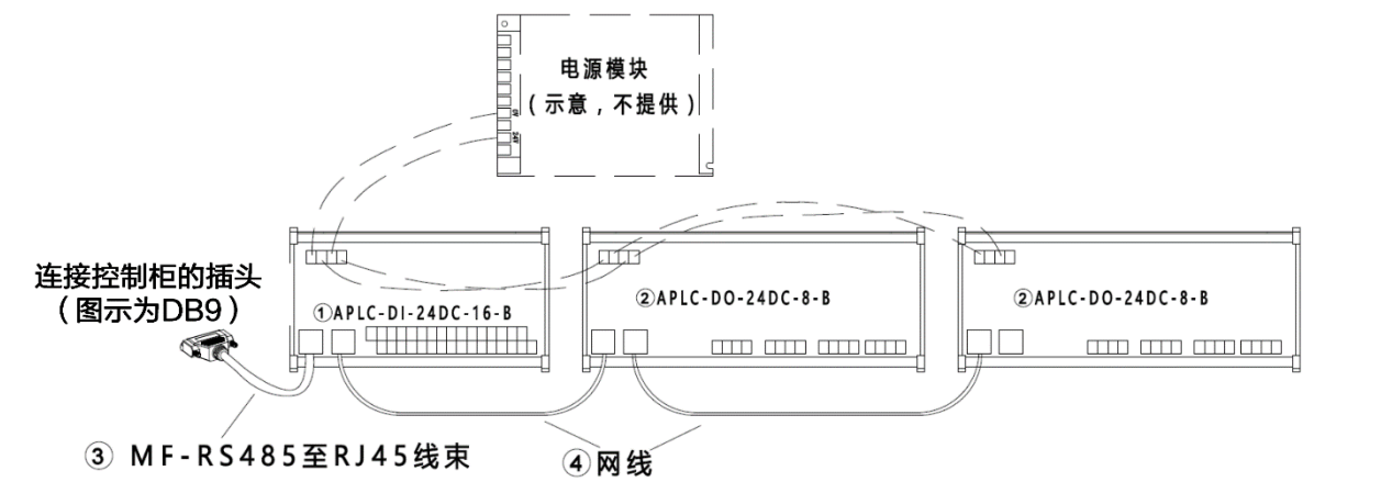
图 20-14 “16 路 DI+16 路 DO” 的连接示意图
