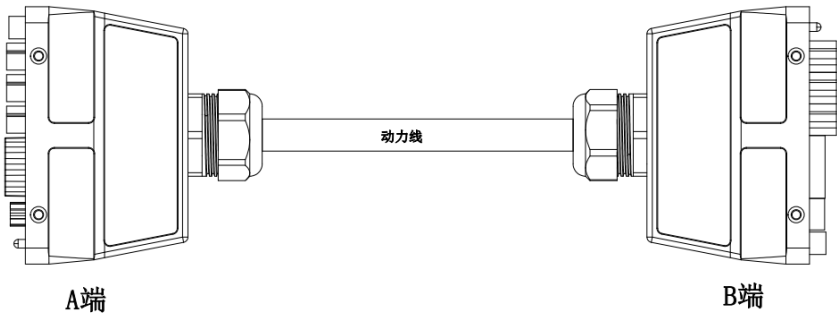
图 9-15 AIR280-2700 柜外重载动力线束示意图
