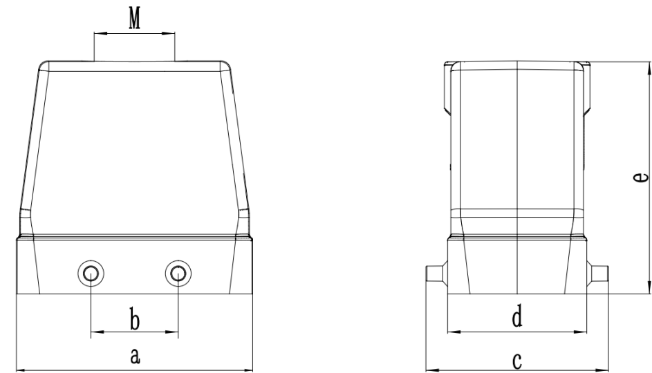
图 9-33 编码器线重载接头尺寸
