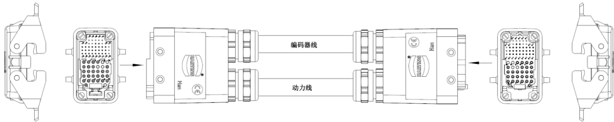
图 9-31 inCube30 拖链重载线示意图
