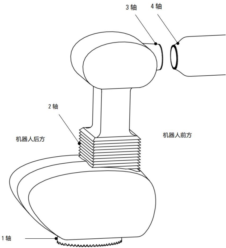
图 2-3 步骤 3 示意图
