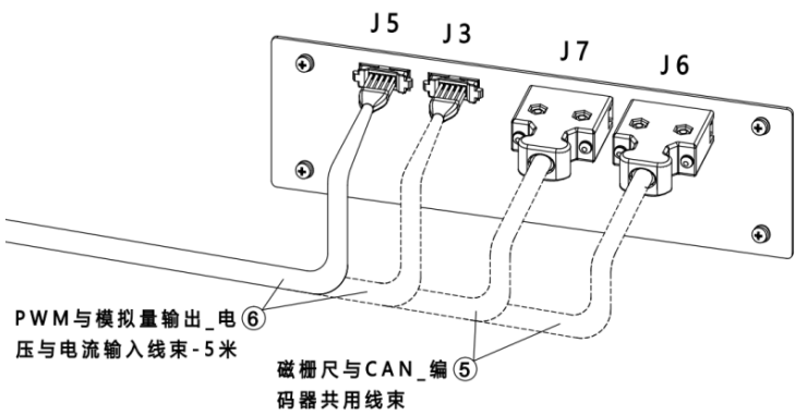
图 21-20 MCBS-IEB 正面示意图
