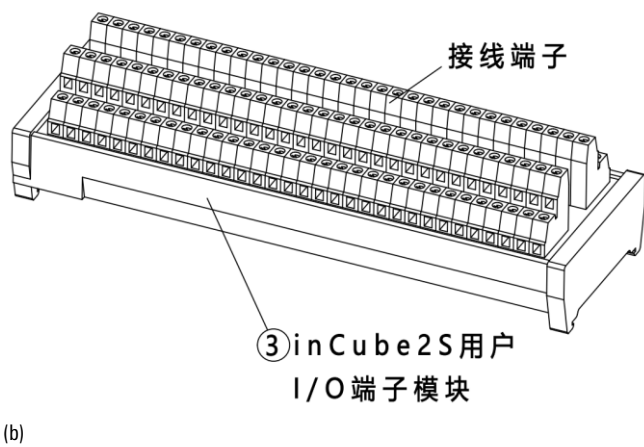
图 19-3 inCube2S 控制柜用户 D0 模块接线示意图
