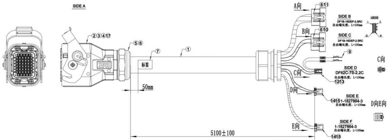
图 9-8 inCube2S-20 标准重载线（AIR12SC/AIR20SC 机型）示意图
