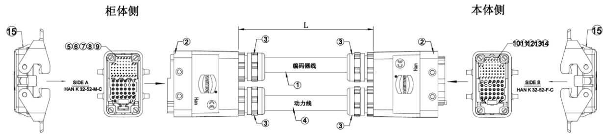
图 9-9 inCube30 标准重载线（适配 AIR4-560C/AIR4-560C-HW 等机型）示意图
