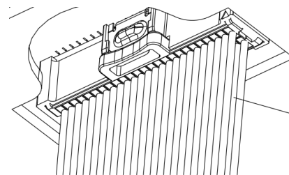
图 21-29 安装 ARC5-MCBS 和扣板连接线
