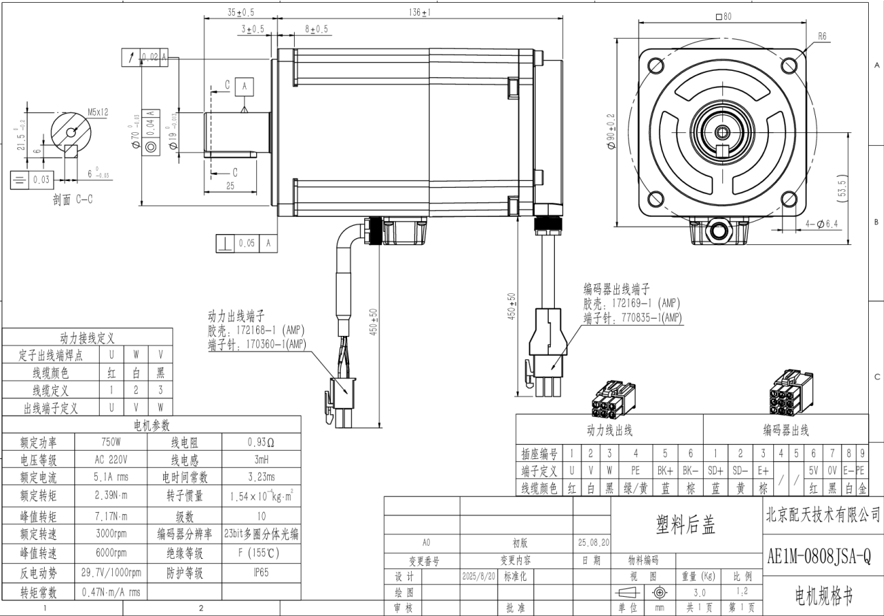
图 28-7 AE1M-0808JSA-Q 电机图纸
