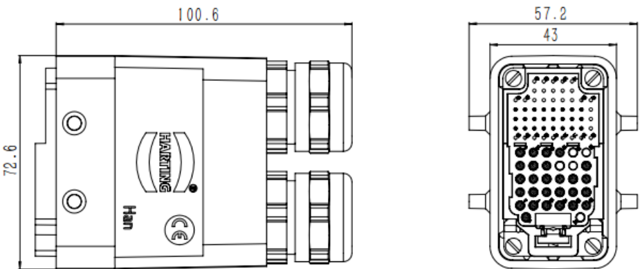
图 9-30 inCube30 重载接头尺寸
