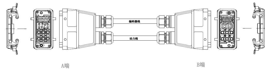
图 9-6 inCube22 标准重载线示意图
