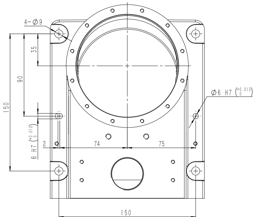
图 3-2 AIR6SC-600A 型操作机基座接口尺寸
