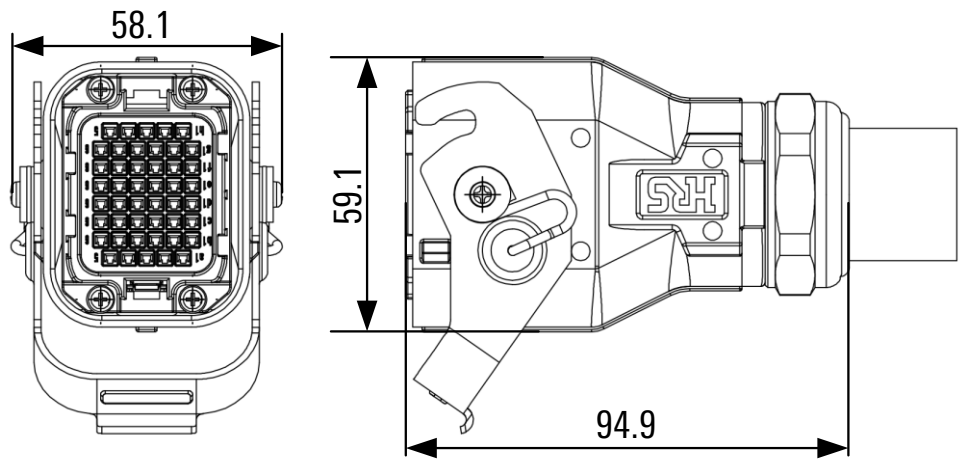
图 4-6 柜侧重载插头尺寸
