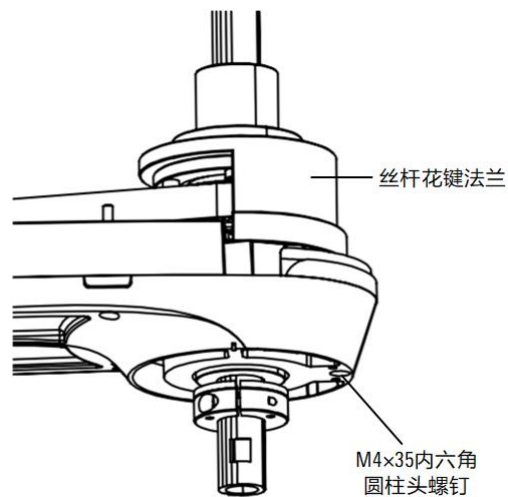
图 8-14 拆卸丝杆花键法兰示意图
