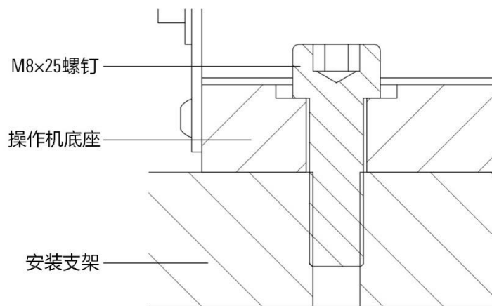
(b) 剖面图
