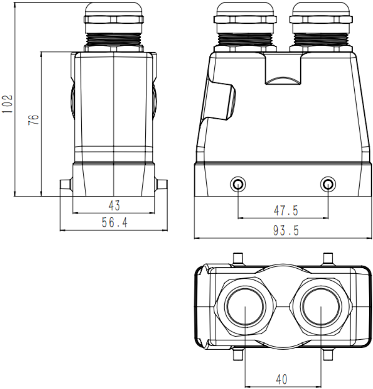
图 9-22 AIR8-710A/AIR10-1420A 机型本体端重载插头尺寸
