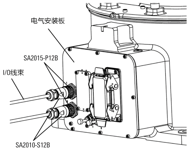
图 5-3 基座上 I/O 线束连接示意图
