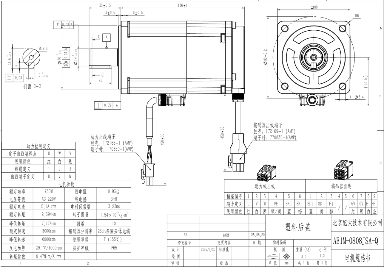
图 28-7 AE1M-0808JSA-Q 电机图纸
