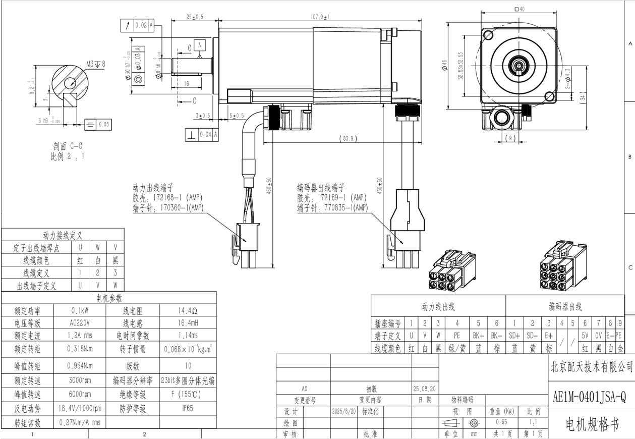
图 28-1 AE1M-0401JSA-Q 电机图纸
