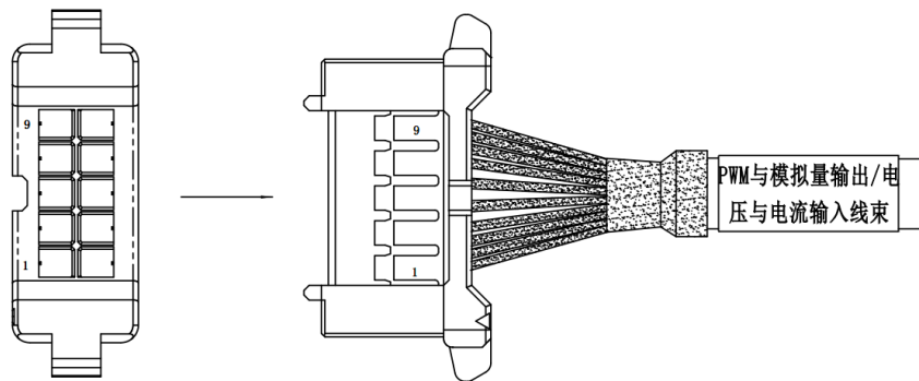
图 21-27 PWM 与模拟量输出_电压与电流输入线束(5m)示意图
