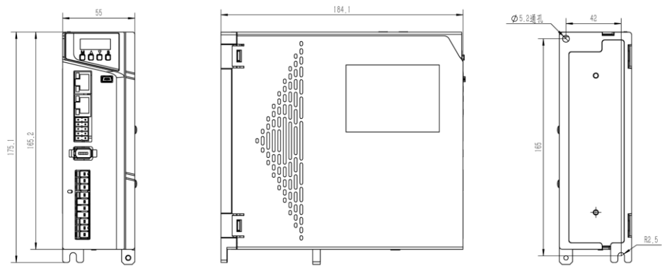
图 28-12 A2E-8R0AI-Q 驱动图纸
