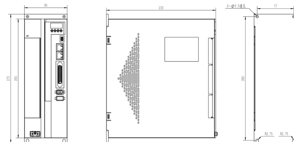
图 28-26 A2E-260TI-Q 驱动图纸
