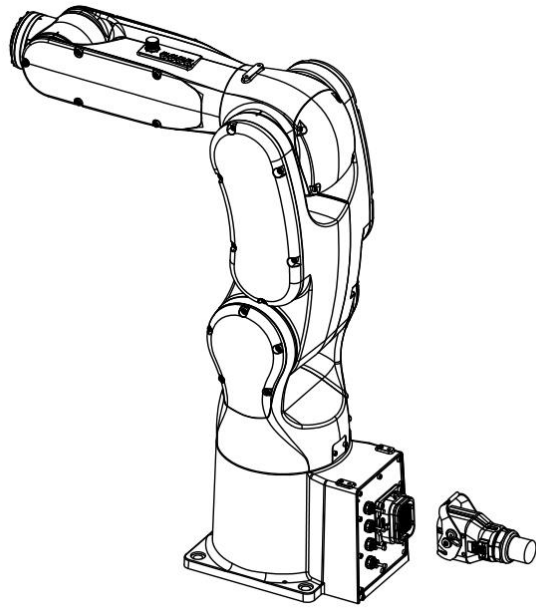
图 3-2 AIR4-560A 本体后出线（标配）示意图
