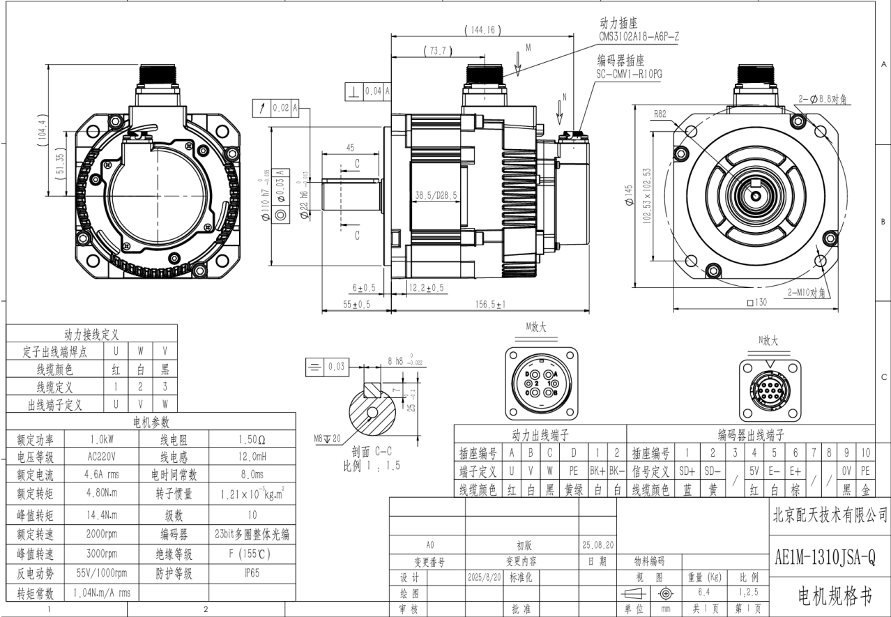
图 28-9 AE1M-1310JSA-Q 电机图纸
