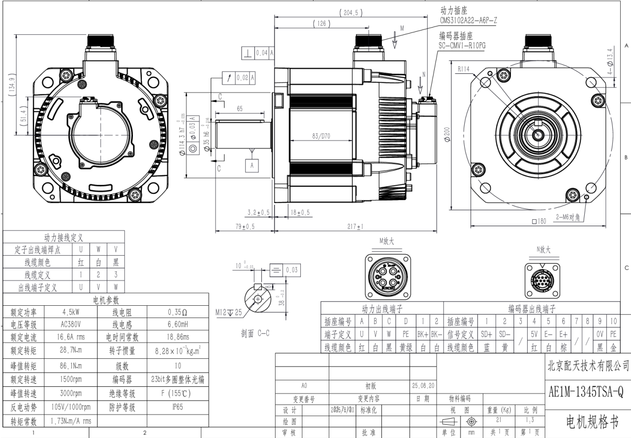
图 28-21 AE1M-1345TSA-Q 电机图纸
