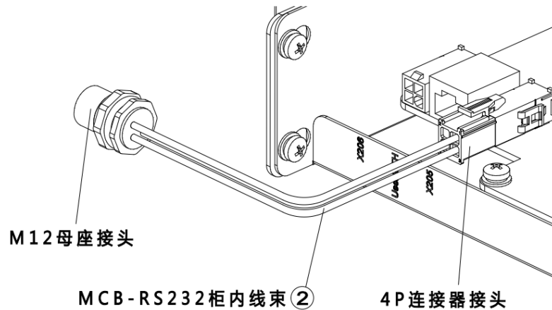
图 13-6 连接 MCB 的 X205 串口示意图
