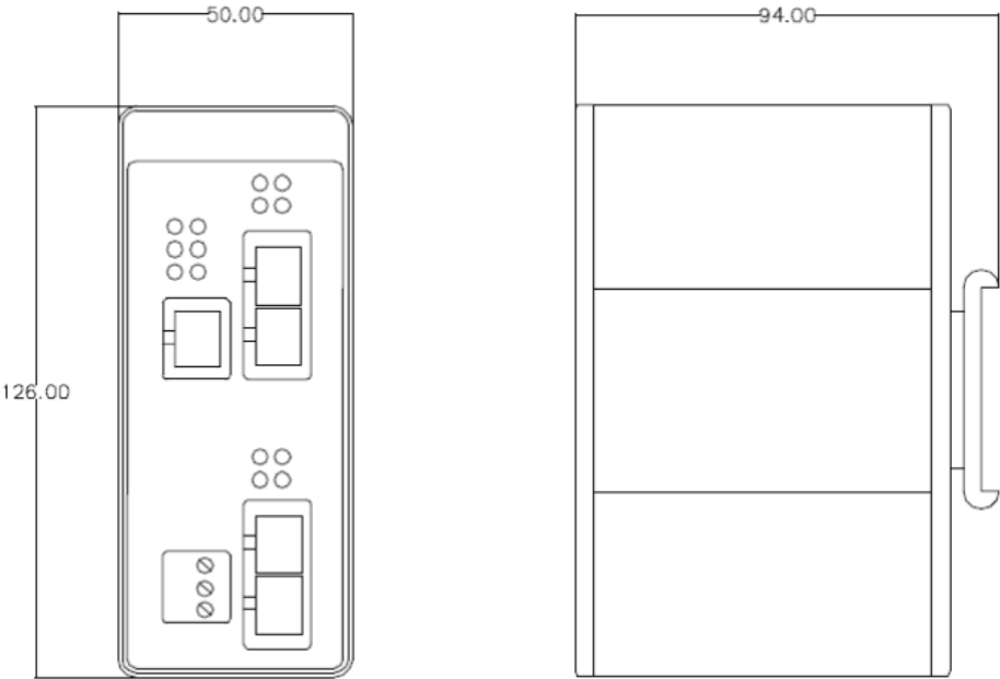
图 18-1 EtherNet/IP 模块的外型尺寸
