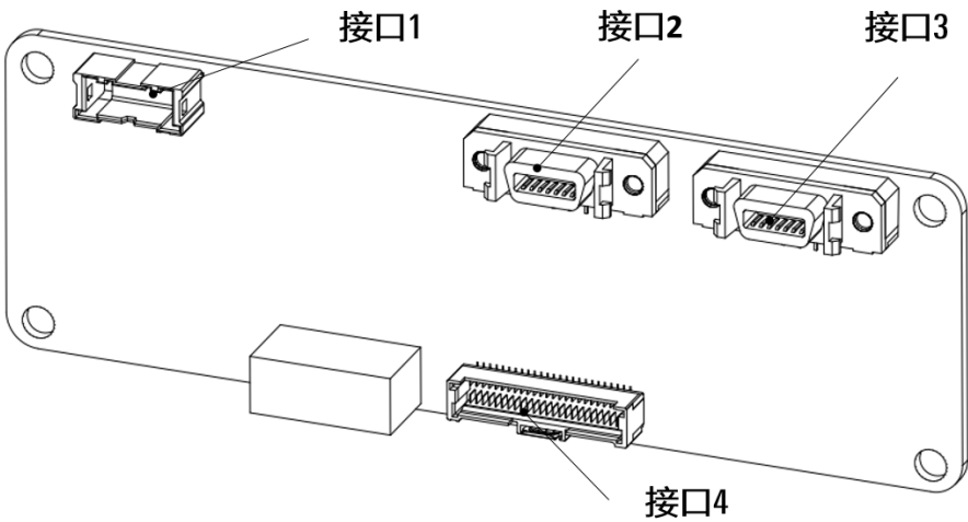
图 21-36 MCB-IEB 接口示意图
