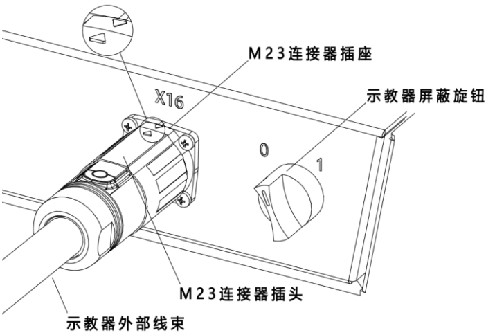
图 10-2 示教器连接接口
