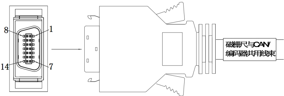
图 21-14 磁栅尺与 CAN_编码器共用线束及 SCSI 引脚示意图
