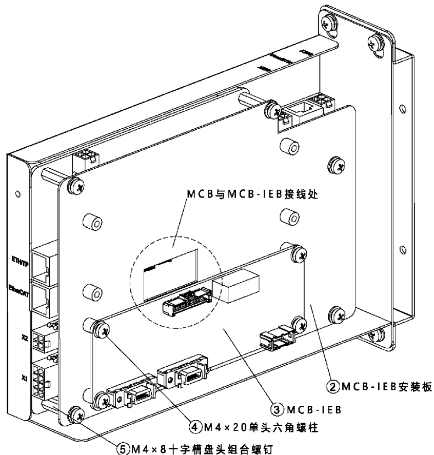
图 21-40 安装 MCB-IEB
