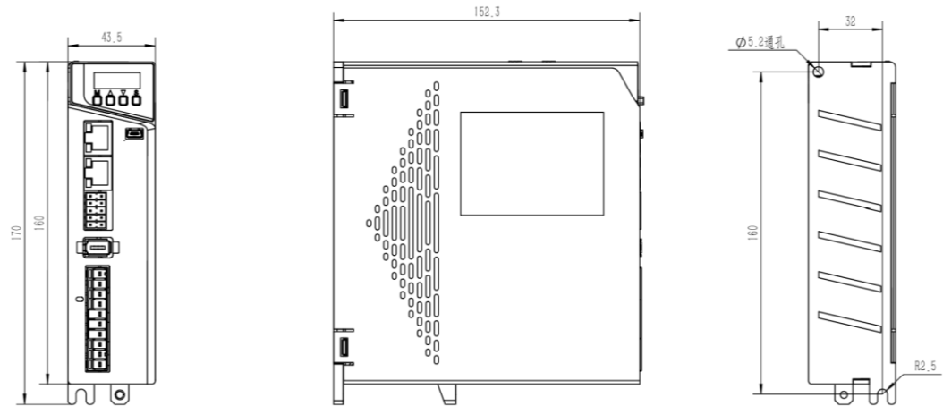
图 28-8 A2E-5R5AI-Q 驱动图纸
