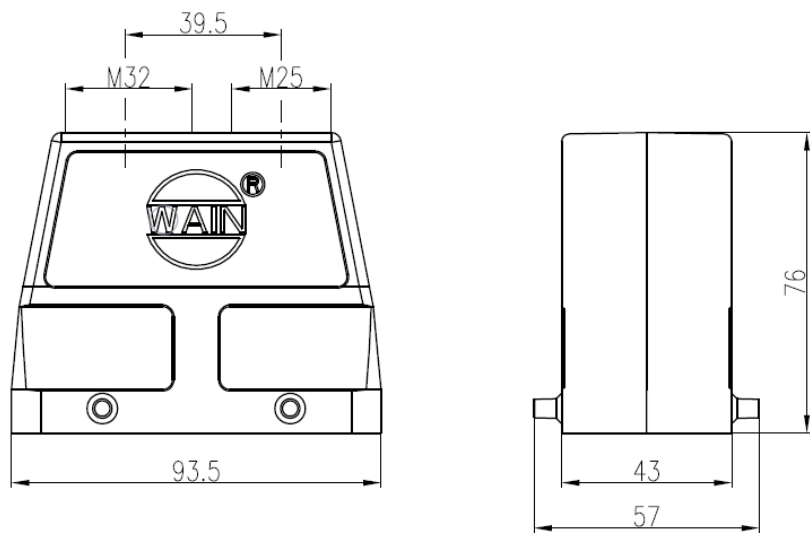
图 9-25 inCube22 重载接头尺寸
