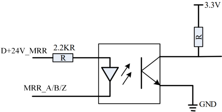
图 21-32 磁栅尺输入电路示意图
