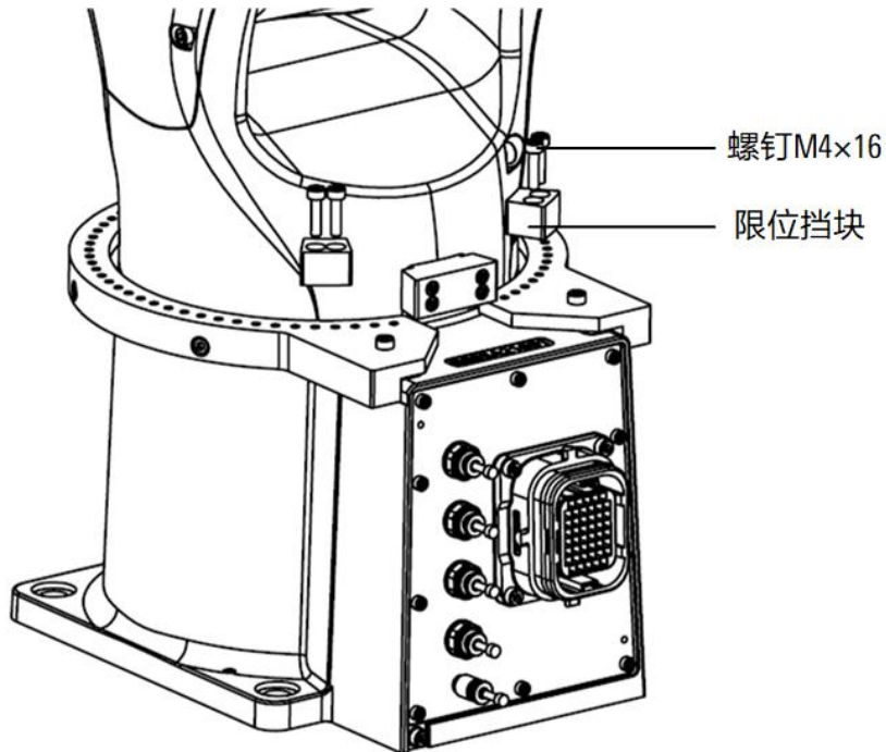
图 6-2 限位块安装示意图
