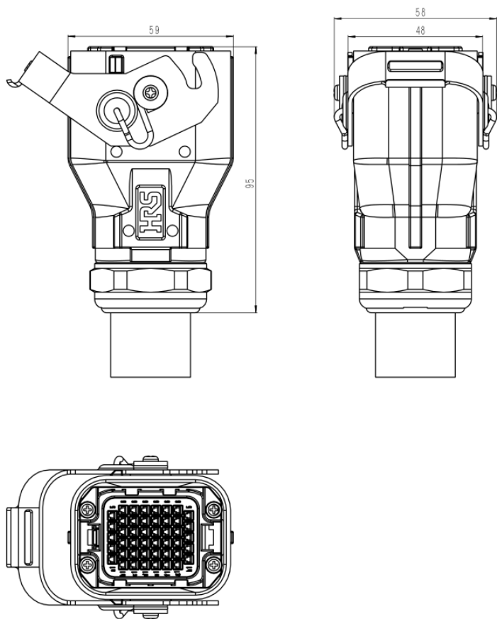
图 9-3 inCube20/2S 重载接头尺寸
