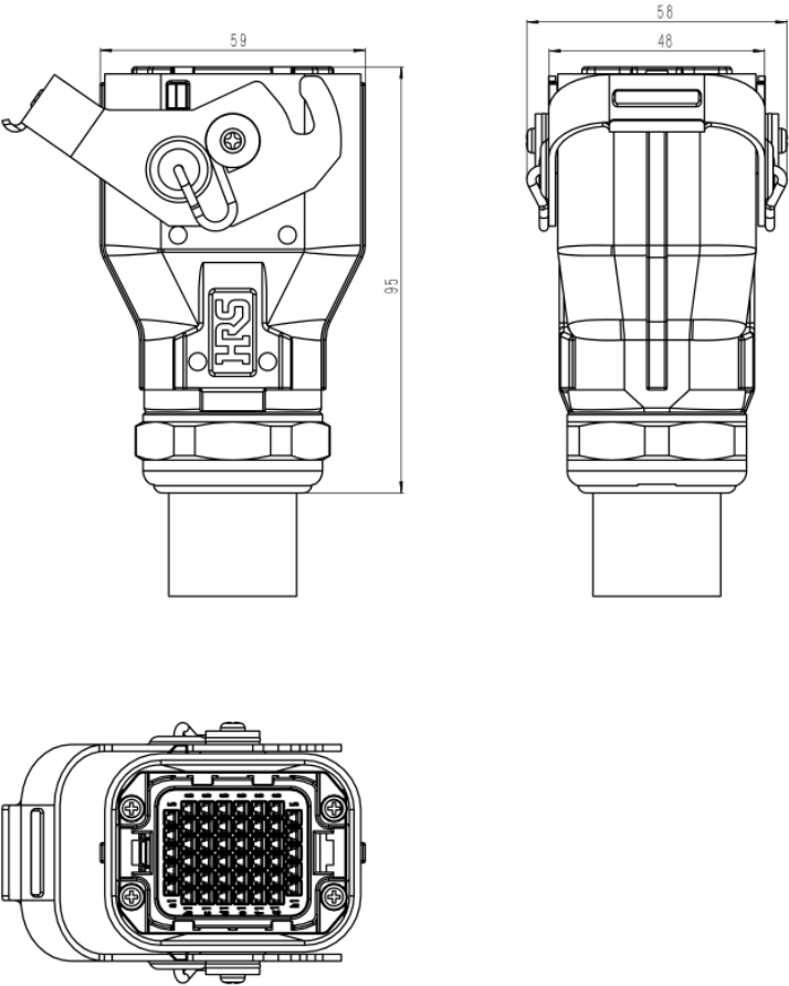
图 3-1 AIR4-560A 本体基座底部出线重载插头尺寸
