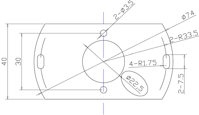
图 29-1 安装支架尺寸图
