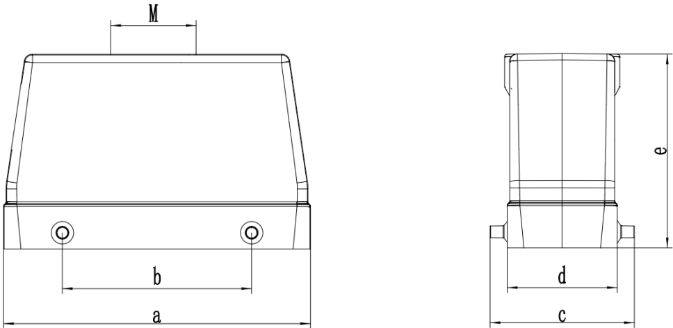
图 9-17 动力线重载插头尺寸示意图
