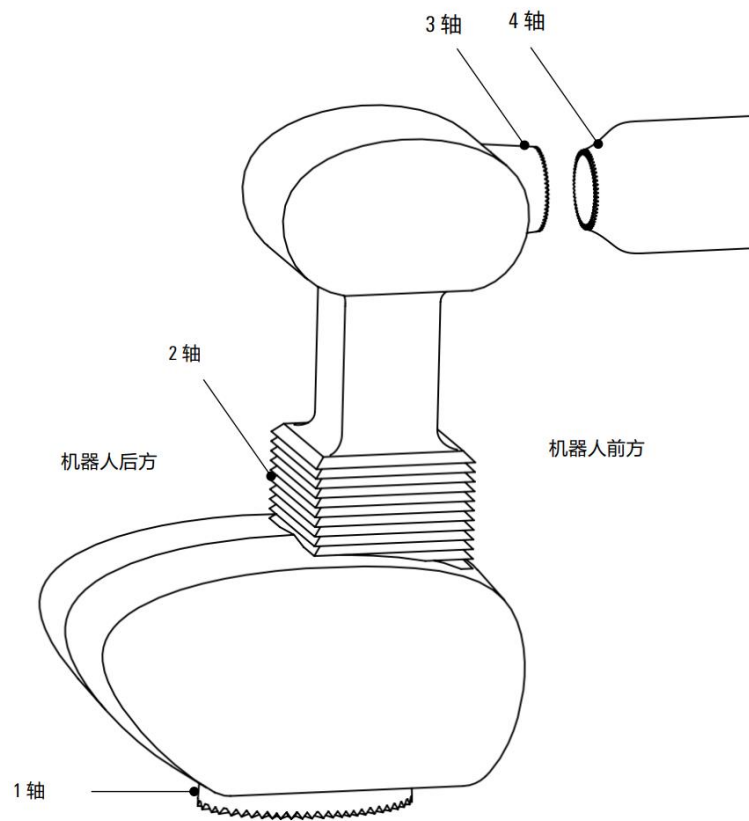
图 2-3 步骤 3 示意图
