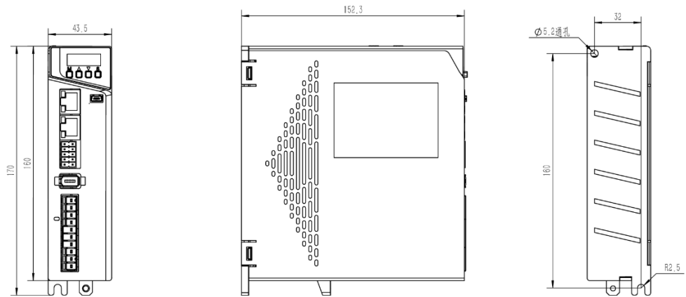
图 28-4 A2E-2R8AI-Q 驱动图纸
