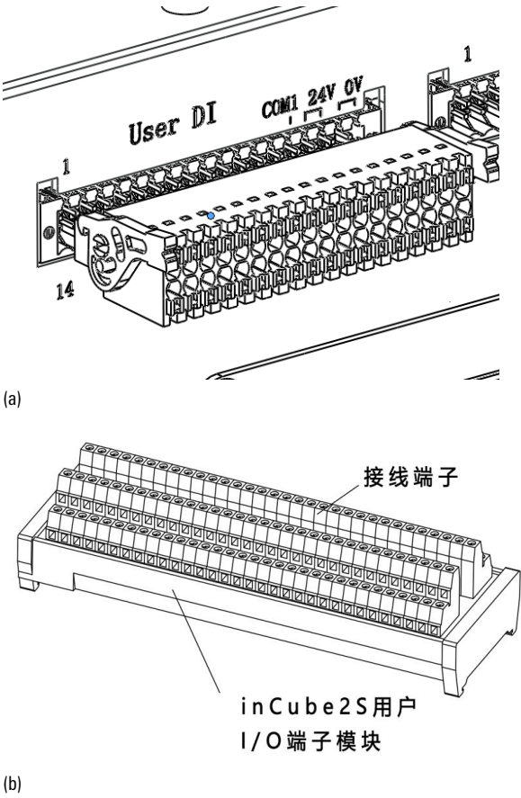
图 19-5 inCube20/22 控制柜用户 DI 模块接线示意图
