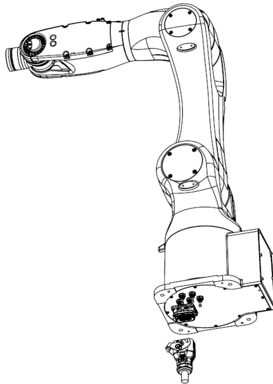
图 3-5 AIR7-920B 本体基座底部出线（选配）示意图
