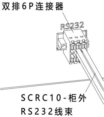
图 13-1 SCRC10-柜外 RS232 线束接线示意图
