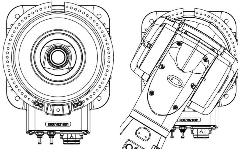
图 6-7 最大限位角度姿态示意图
