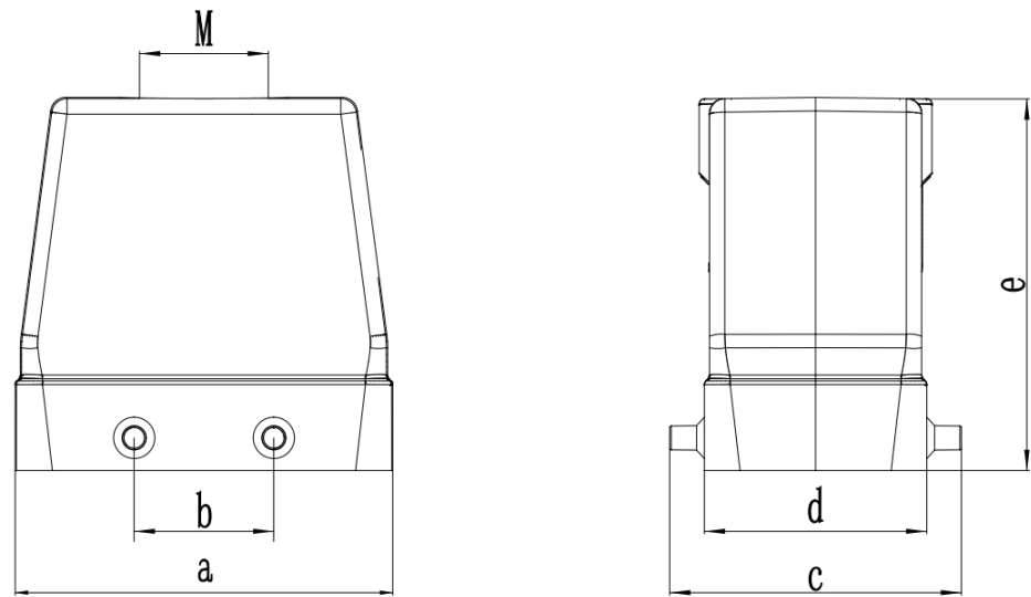
图 9-19 编码器线重载插头示意图
