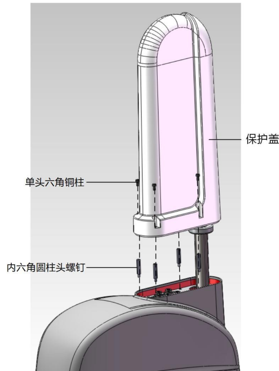
图 4-3 保护盖安装示意图
