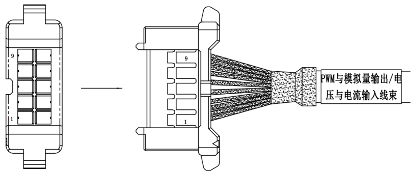
图 21-15 PWM 与模拟量输出_电压与电流输入线束(5m)示意图
