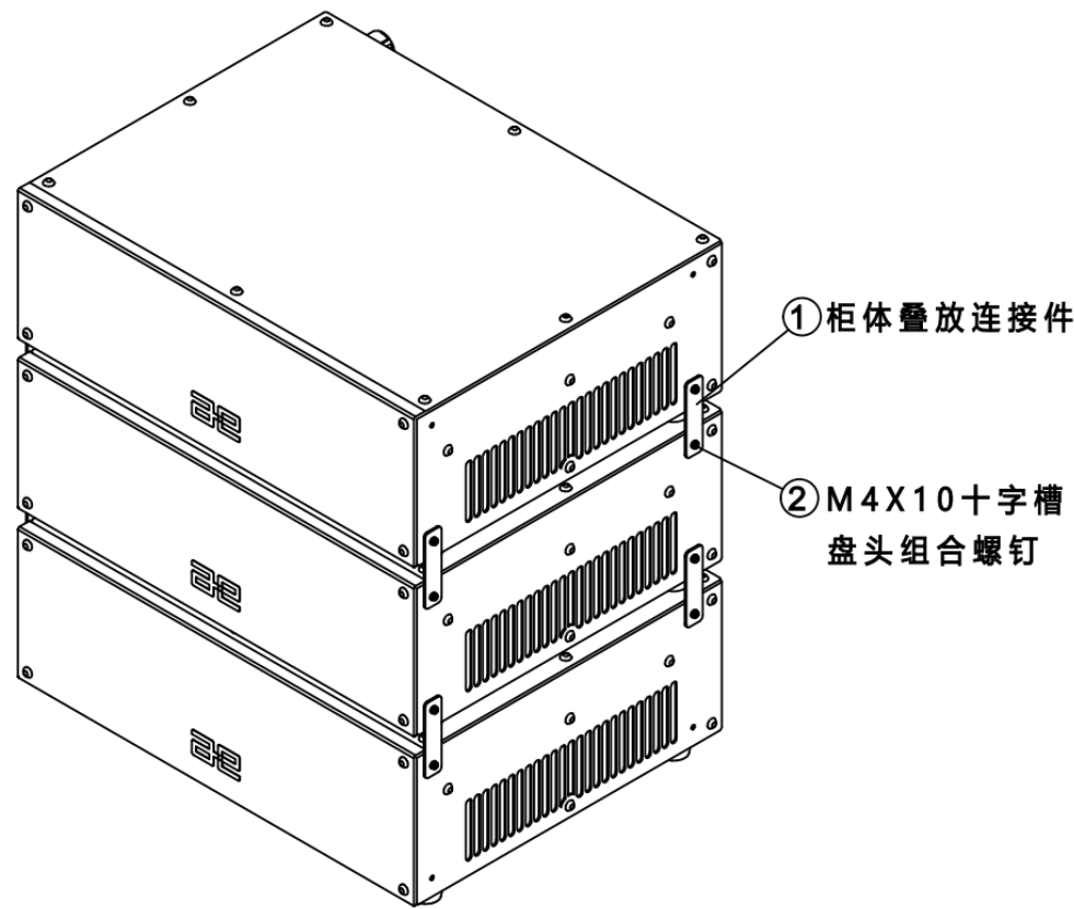
图 25-1 inCube2S 控制柜叠放效果
