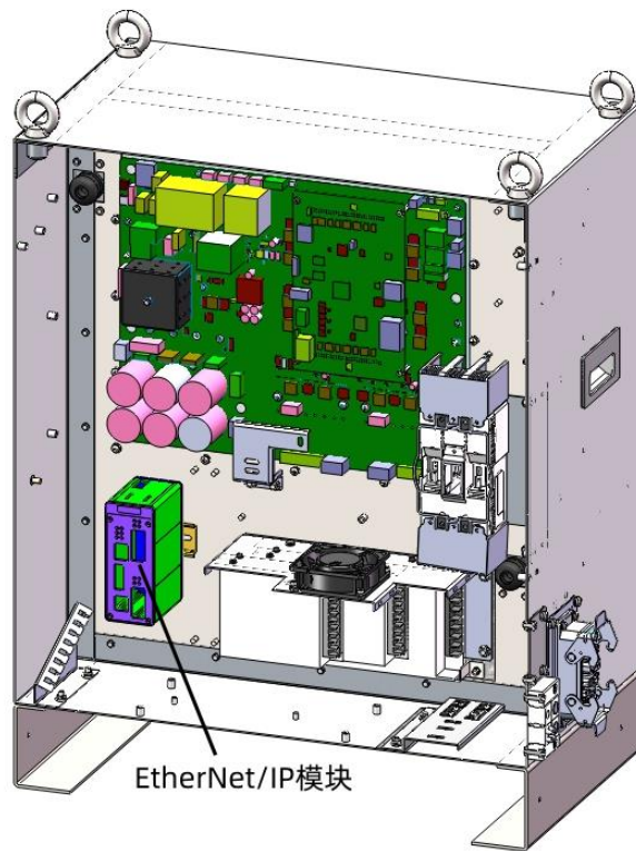
图 18-8 ARC5-12/25 控制柜安装 EtherNet/IP 模块
