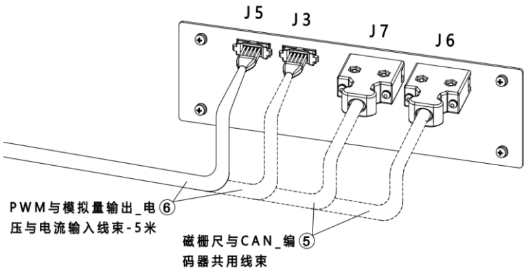
图 21-8 MCBS-IEB 正面示意图
