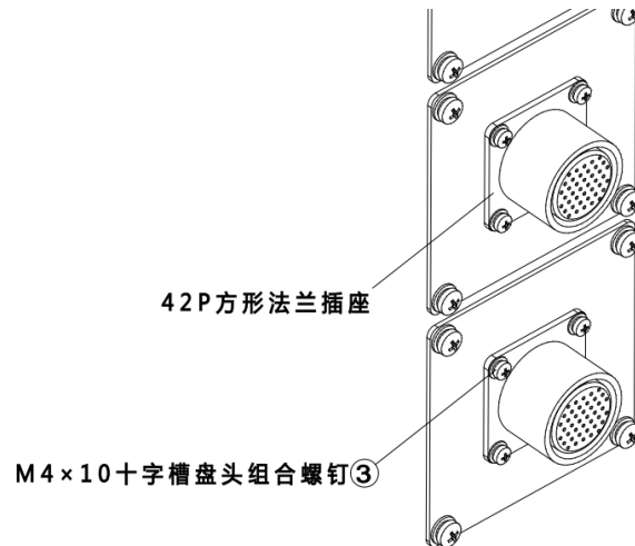
图 19-12 42P 方形法兰插座
