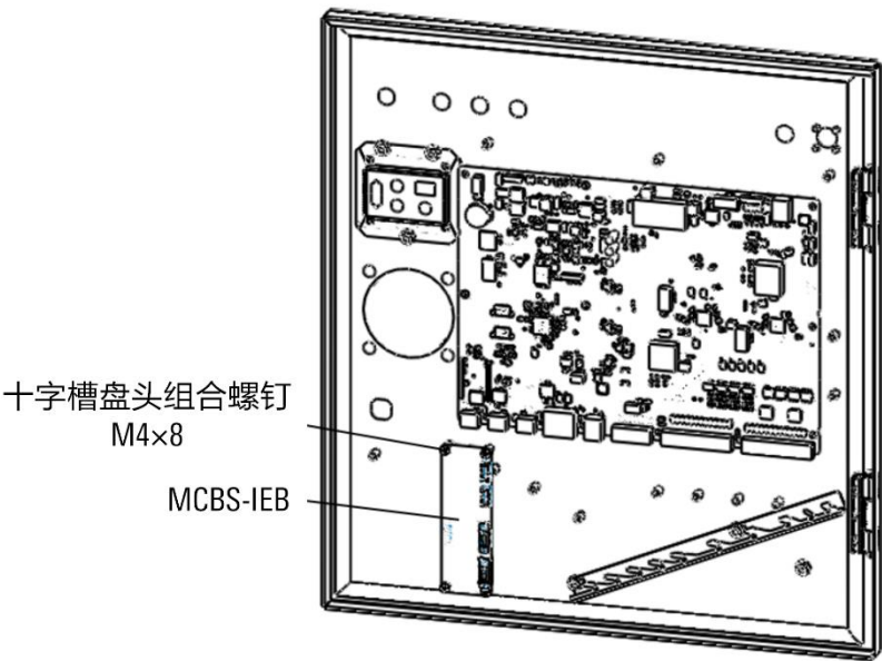
图 21-30 MCBS-IEB 安装示意图
