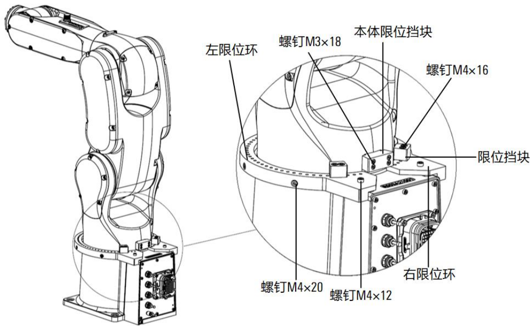
图 6-1 AIR4-560A 安装限位环总览图
