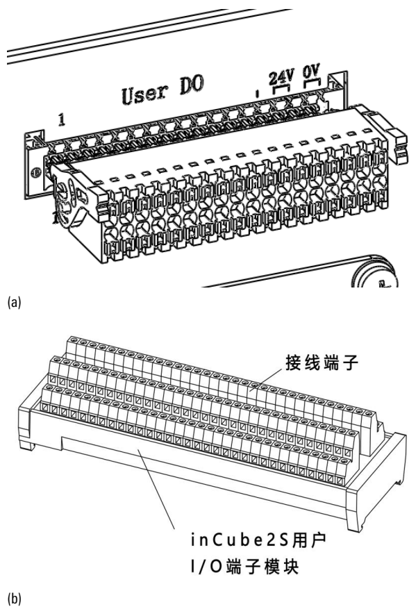
图 19-6 inCube20/22 控制柜用户 DO 模块接线示意图
