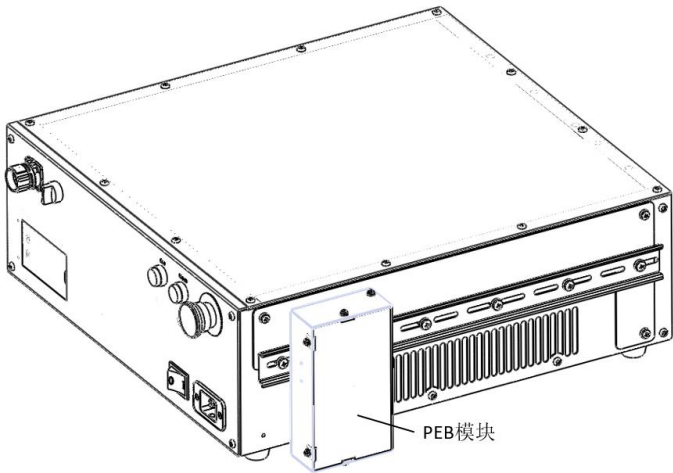
图 16-4 将 PEB 模块安装在导轨上
