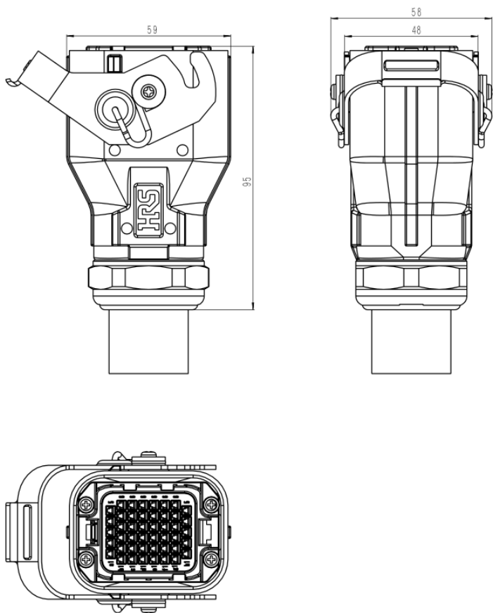
图 9-24 inCube20/2S 重载接头尺寸
