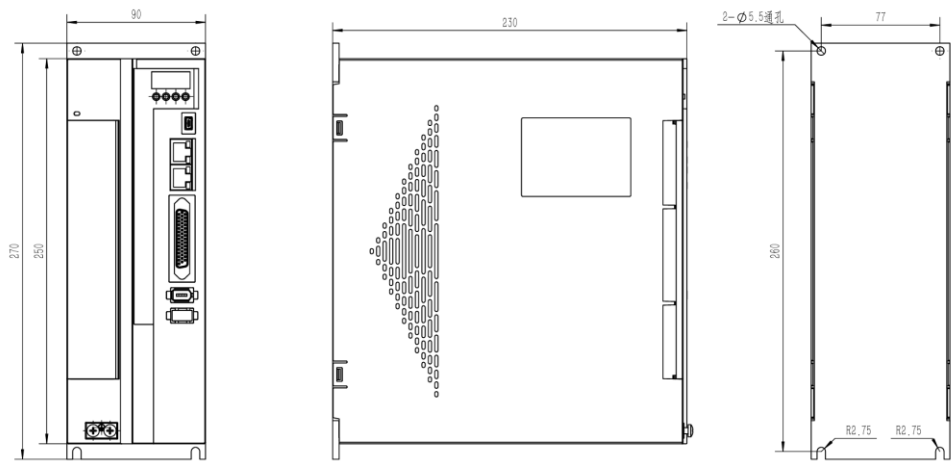
图 28-22 A2E-170TI-Q 驱动图纸
