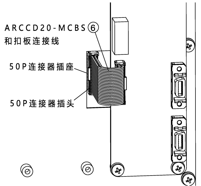
图 21-41 MCB 和 MCB-IEB 连接
