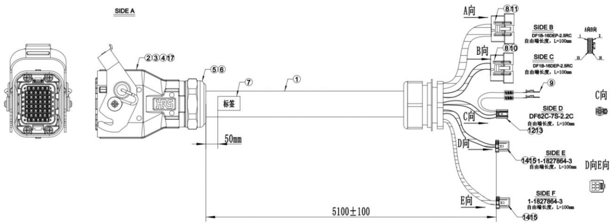
图 9-9 inCube2S-20 标准重载线（AIR12SC/AIR20SC 机型）示意图
