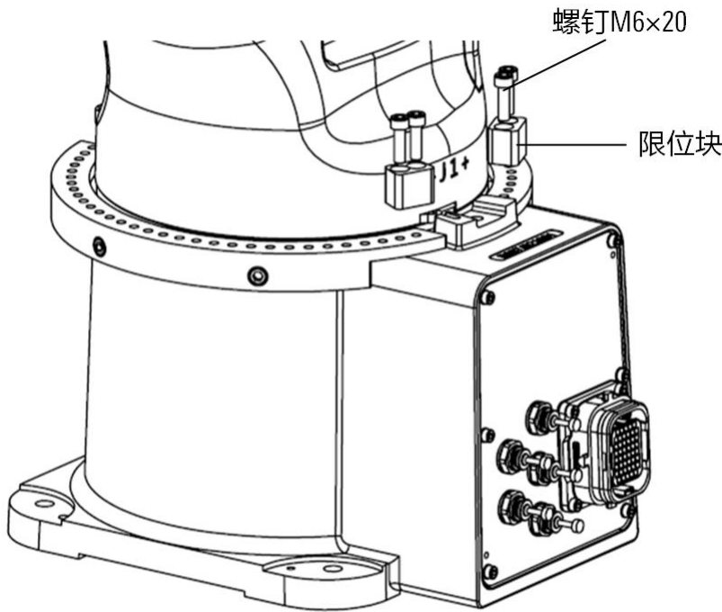
图 6-6 限位块安装示意图
