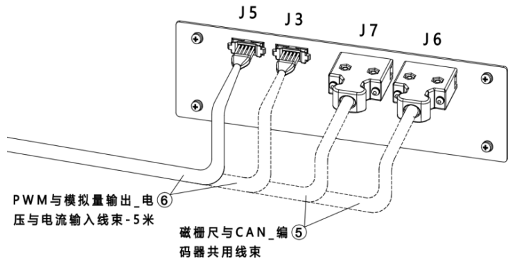
图 21-20 MCBS-IEB 正面示意图
