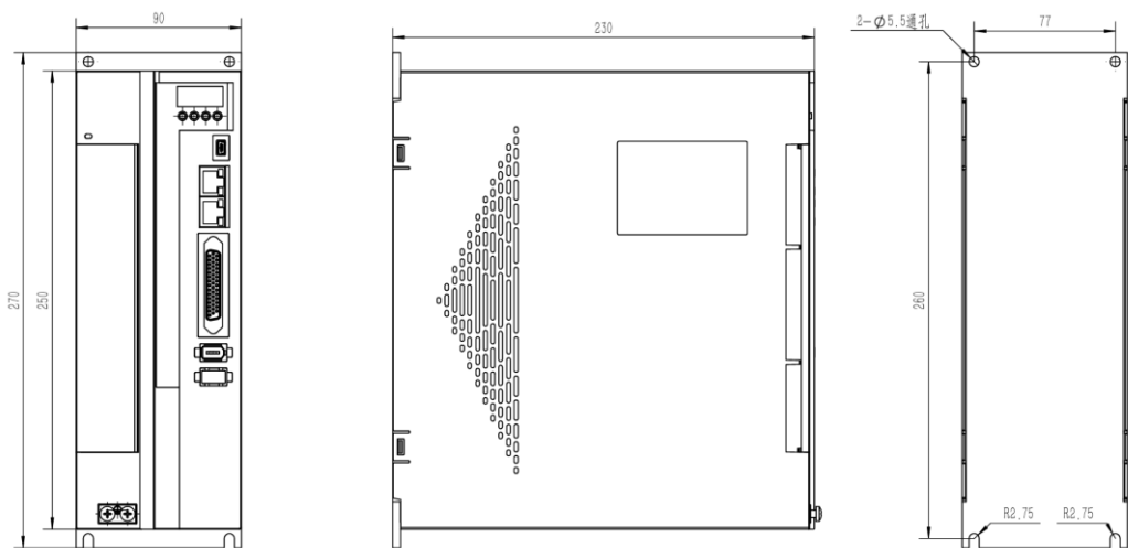
图 28-24 A2E-210TI-Q 驱动图纸
