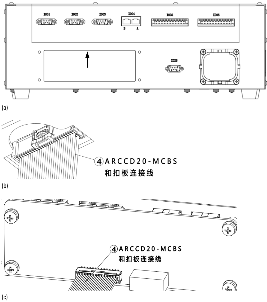
图 21-6 安装 ARCCD20-MCBS 和扣板连接线
