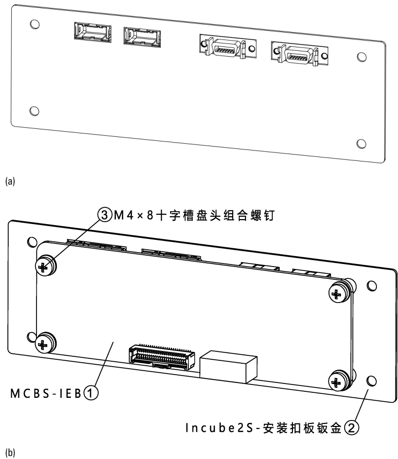
图 21-17 安装 MCBS-IEB
