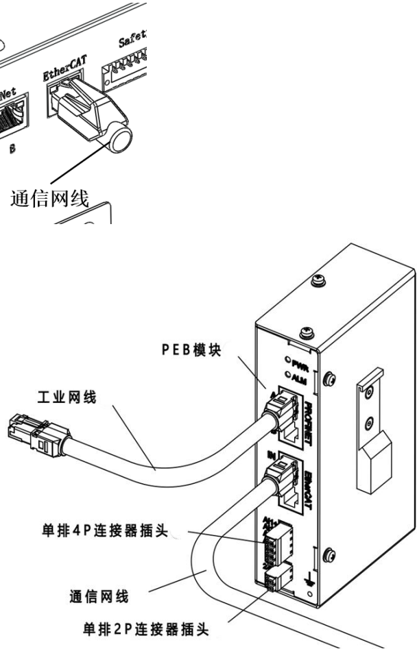
图 16-5 PEB 模块接线
