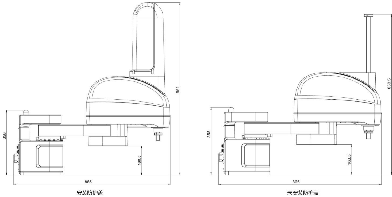
图 4-1 AIR12SC 的 400mm 行程的丝杆防护盖尺寸对比示意图
