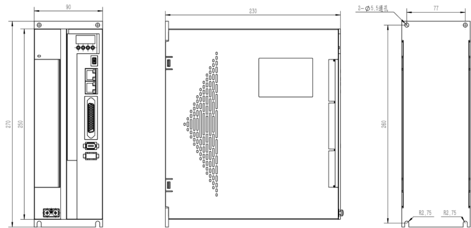
图 28-20 A2E-100TI-Q 驱动图纸
