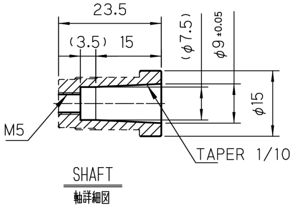
(b) 编码器对外连接孔剖面图
