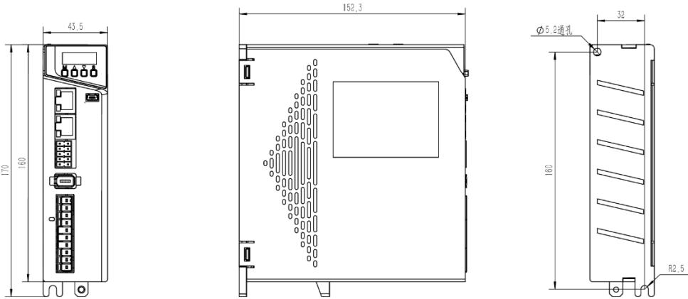
图 28-2 A2E-2R8AI-Q 驱动图纸
