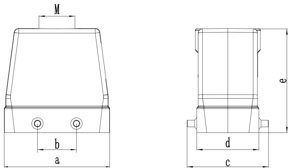
图 9-32 编码器线重载接头尺寸
