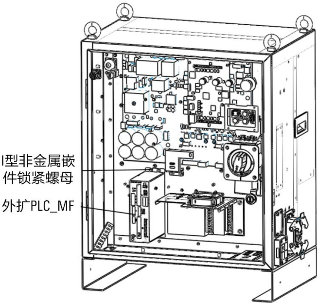
图 20-3 在 ARC5 柜内安装外扩 PLC_MF
