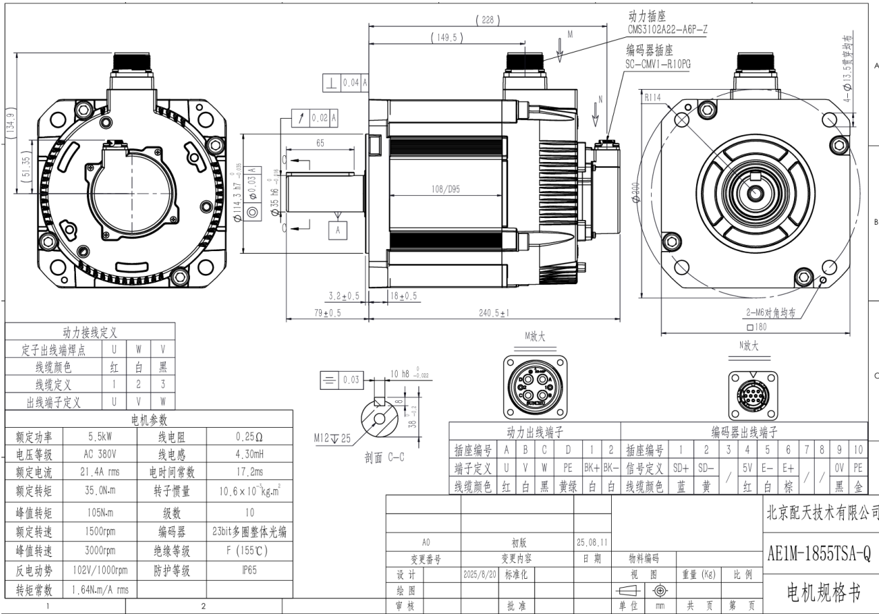
图 28-23 AE1M-1855TSA-Q 电机图纸
