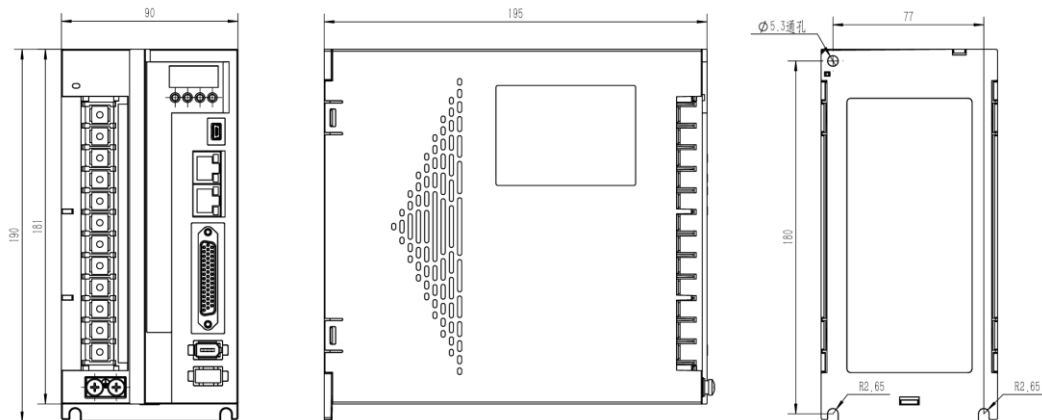
图 28-16 A2E-8R5AI-Q 驱动图纸
