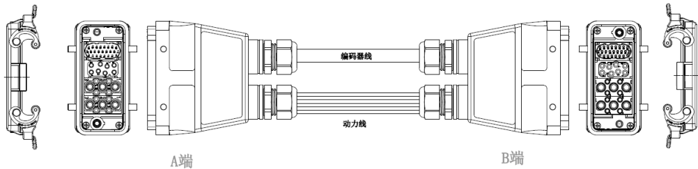
图 9-27 inCube22 重载拖链线外形示意图
