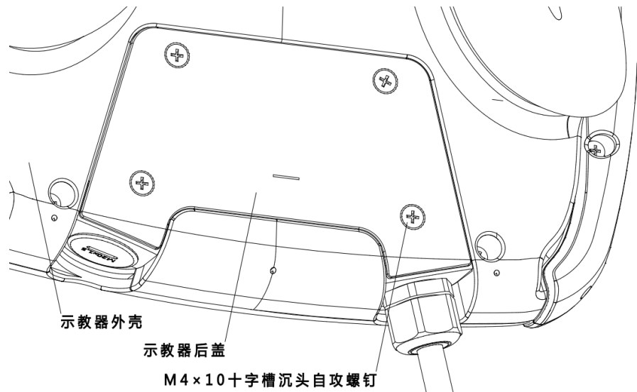
图 10-9 更换示教器外部线束示意图 1
