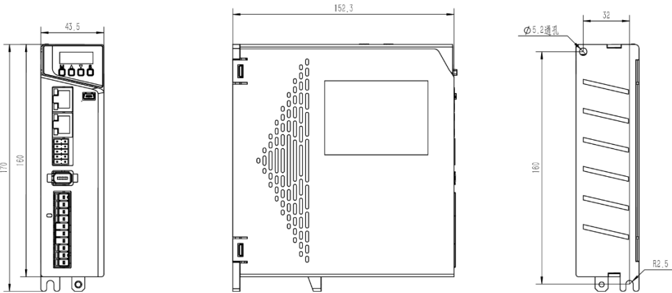
图 28-6 A2E-2R8AI-Q 驱动图纸
