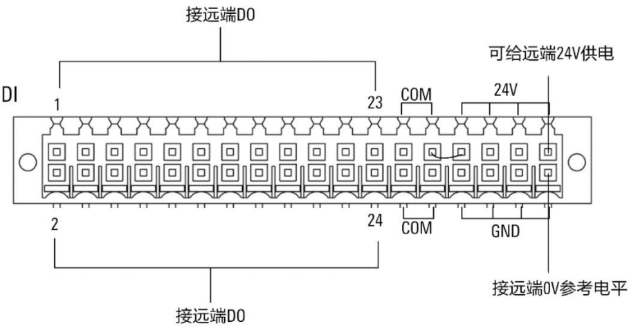
图 20-15 User DI 接口使用说明（NPN 输入）
