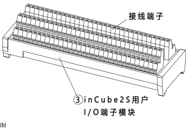
图 19-3 inCube2S 控制柜用户 DO 模块接线示意图
