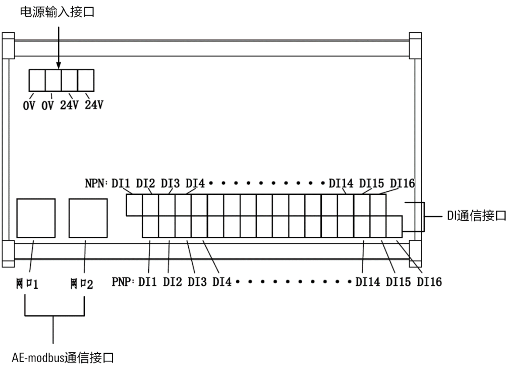
图 20-12 BDI 模块接口示意图
