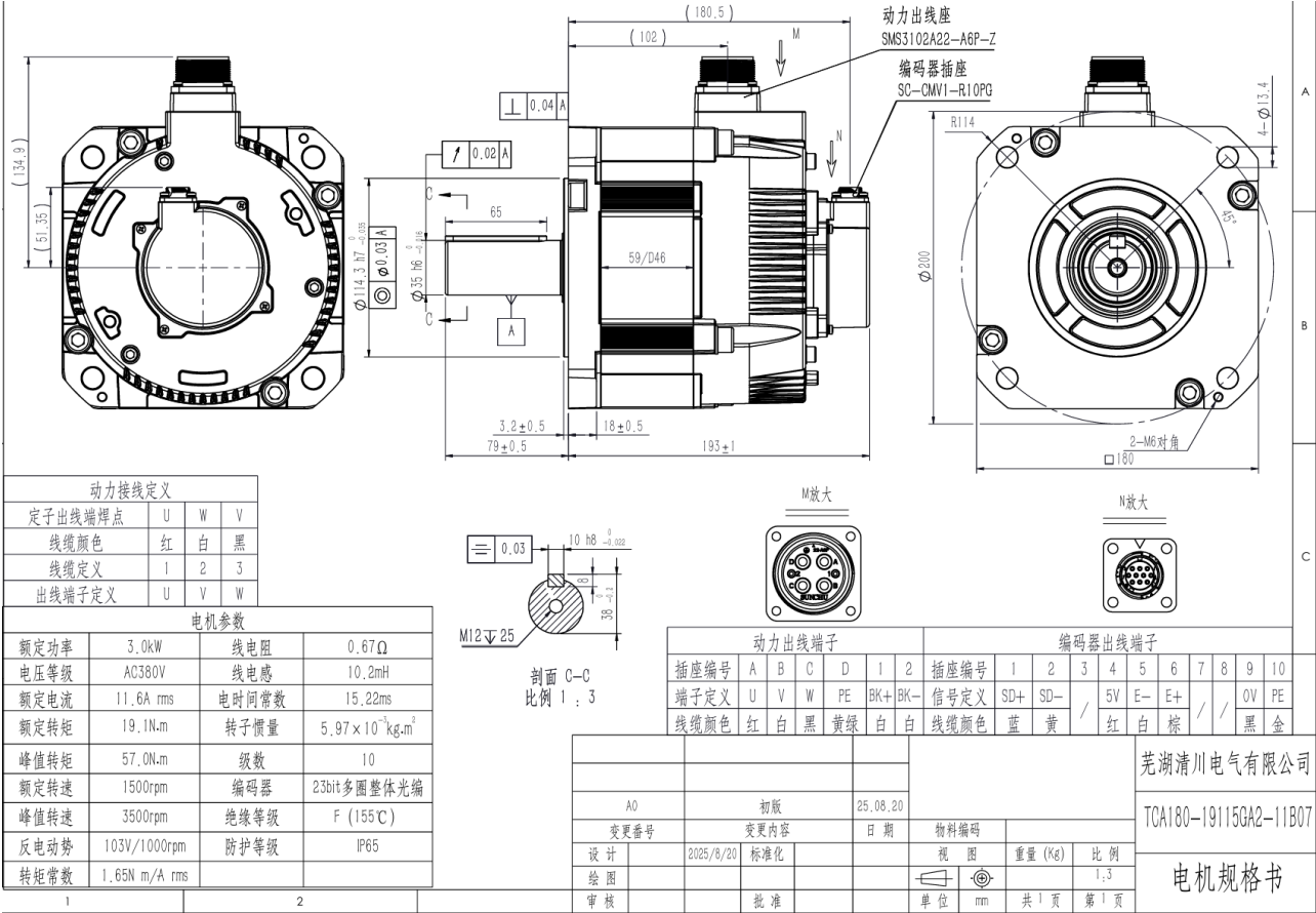
图 28-19 AE1M-1829TSA-Q 电机图纸
