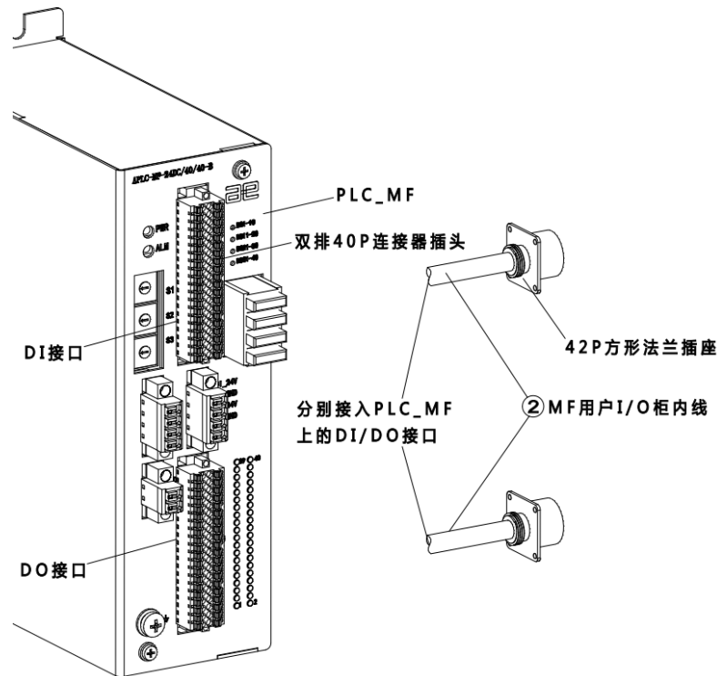
图 19-13 连接 PLC_MF 上的 DI/DO 接口
