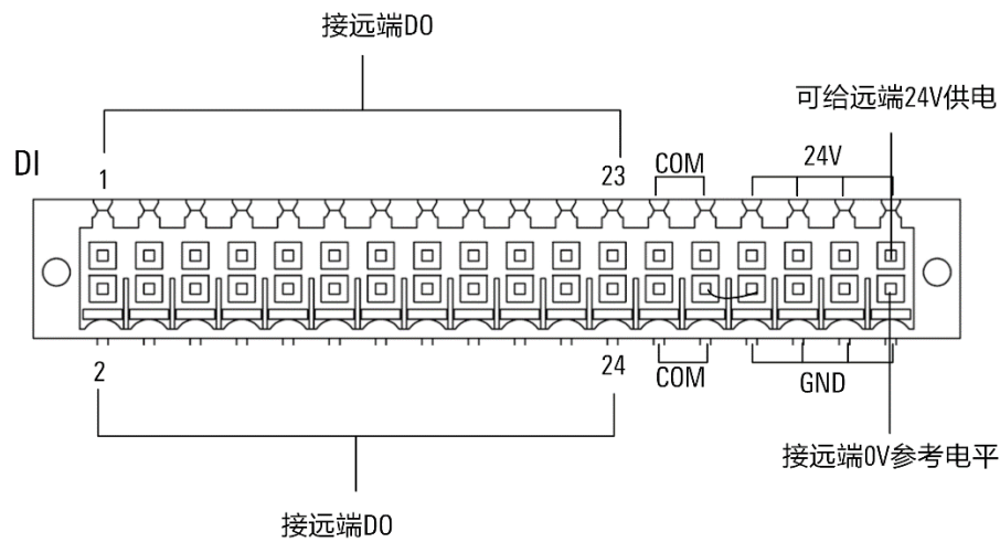
图 20-16 User DI 接口使用说明（PNP 输入）
