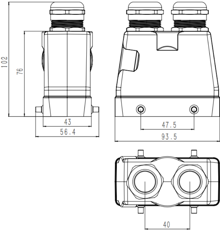
图 9-1 AIR8-710A/AIR10-1420A 机型本体端重载插头尺寸
