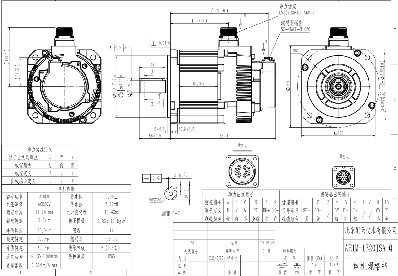
图 28-13 AE1M-1320JSA-Q 电机图纸
