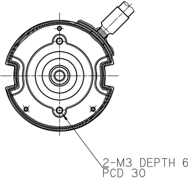
(a) 编码器仰视图
