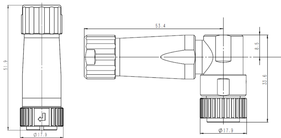
(c) 直管航插与弯管航插的外形尺寸
