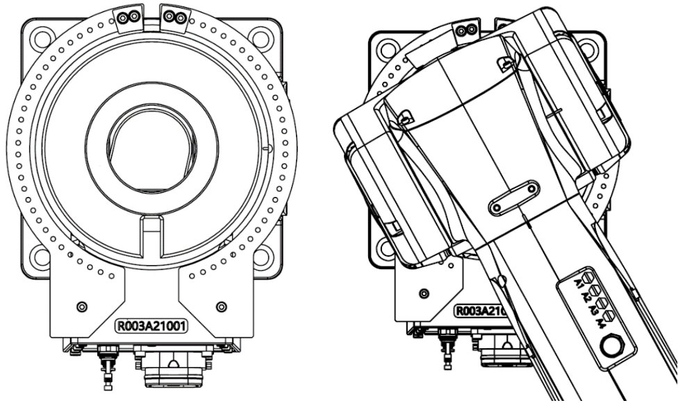
图 6-4 最大限位角度姿态示意图
