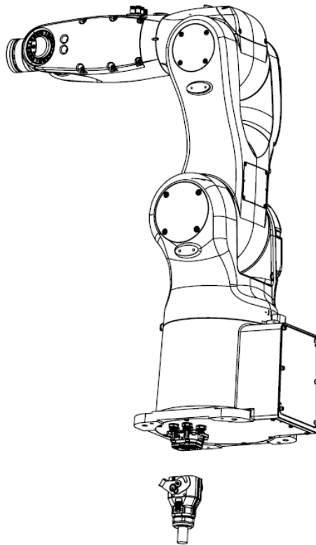
图 3-7 AIR8-710B 本体基座底部出线（选配）示意图
