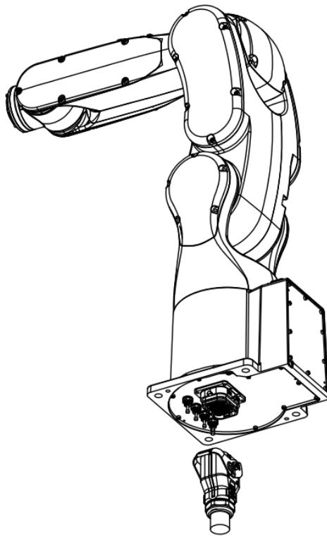
图 3-3 AIR4-560A 本体基座底部出线（选配）示意图
