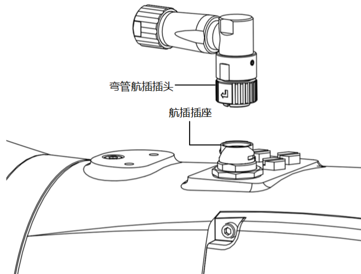
图 1-4 步骤 2 图示
