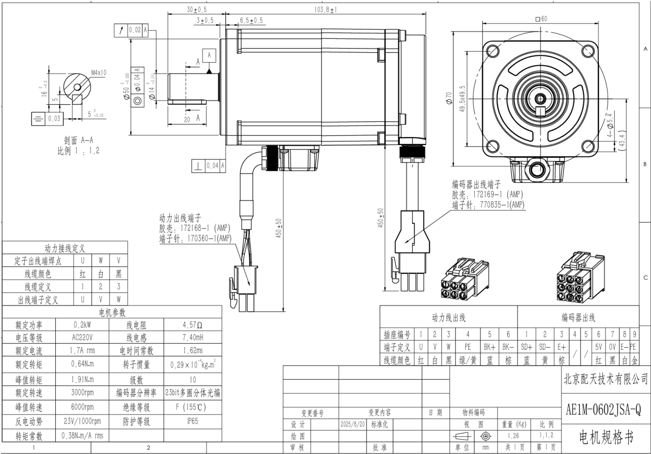
图 28-3 AE1M-0602JSA-Q 电机图纸
