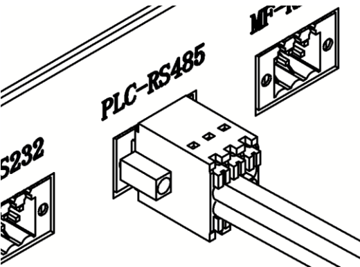
图 15-1 外扩 Modbus 接线
