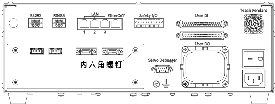
图 21-19 inCube2S-安装扣板钣金固定后示意图
