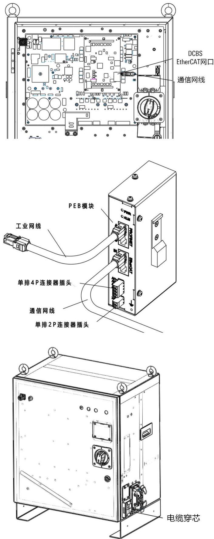
图 16-6 PEB 模块接线
