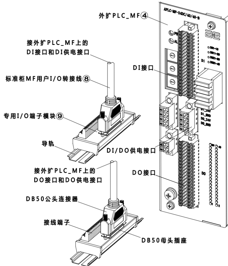
图 20-11 连接用户 I/O 端子示意图
