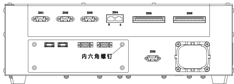
图 21-7 ARCCD20-安装扣板钣金固定后示意图
