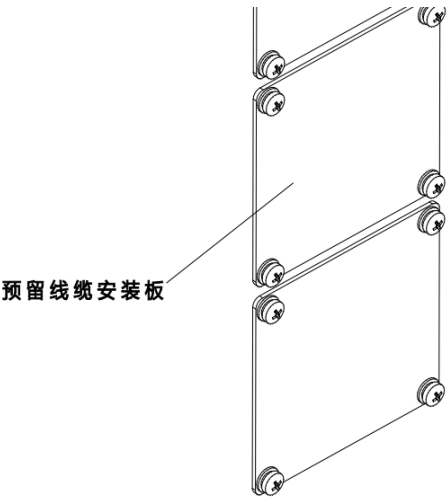
图 19-10 预留线缆安装板
