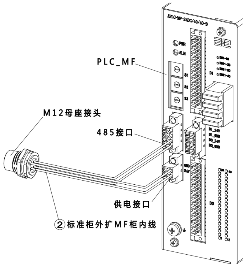
图 20-9 连接外扩 MF 示意图
