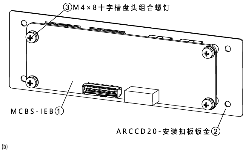
图 21-5 安装 MCBS-IEB
