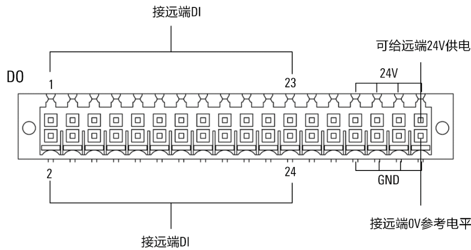
图 20-17 User D0 接口使用说明
