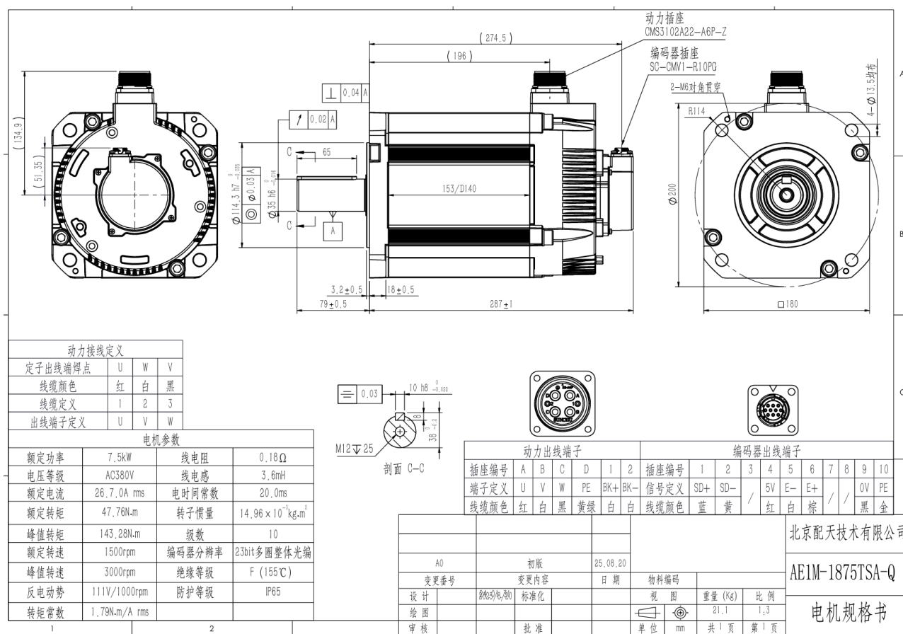
图 28-25 AE1M-1875TSA-Q 电机图纸
