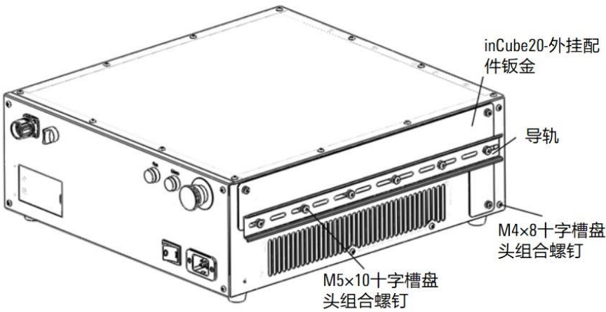
图 18-4 安装 inCube20-外挂钣金与导轨
