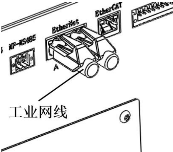
图 14-3 inCube20 /22 的 Ethernet 接线示意图
