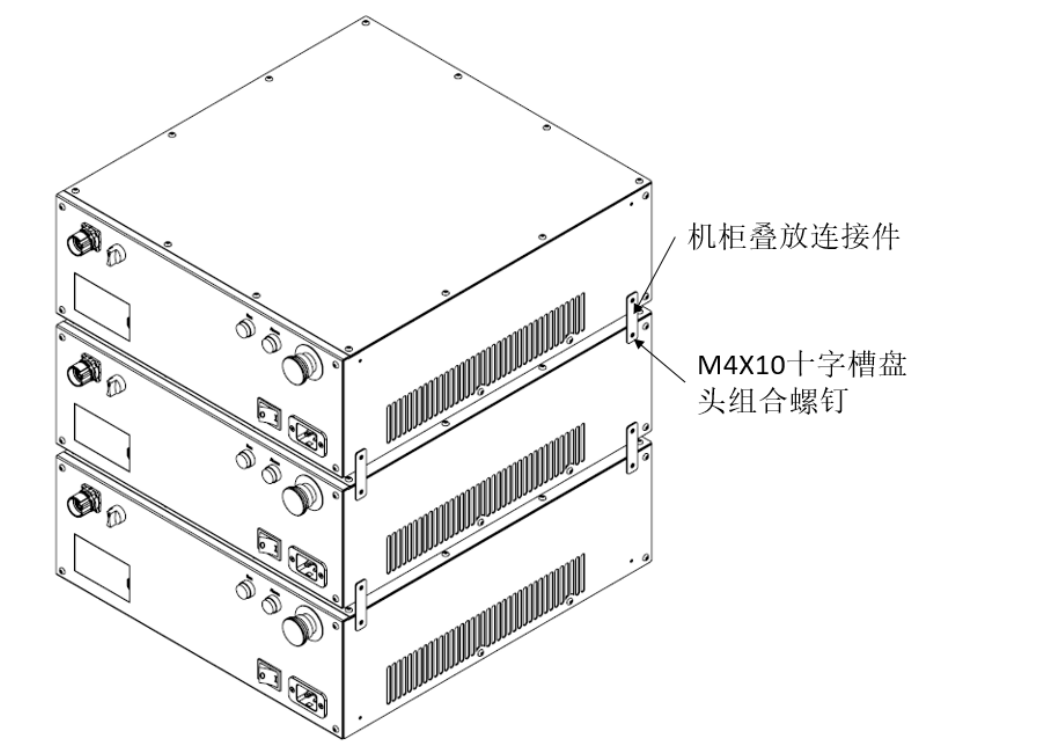
图 25-2 inCube20/22 控制柜叠放效果
