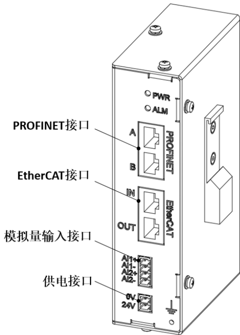
图 16-1 PEB 模块接口示意图
