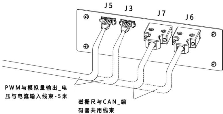
图 21-31 MCBS-IEB 正面示意图
