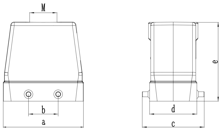
图 9-12 编码器线重载接头尺寸
