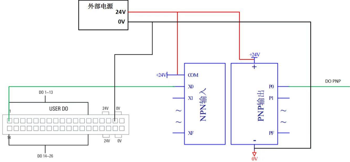
图 23-3 极性转换模块与控制柜连接示意图
