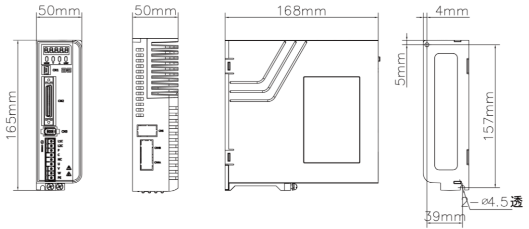
图 29-3 S2E 伺服驱动器外观
