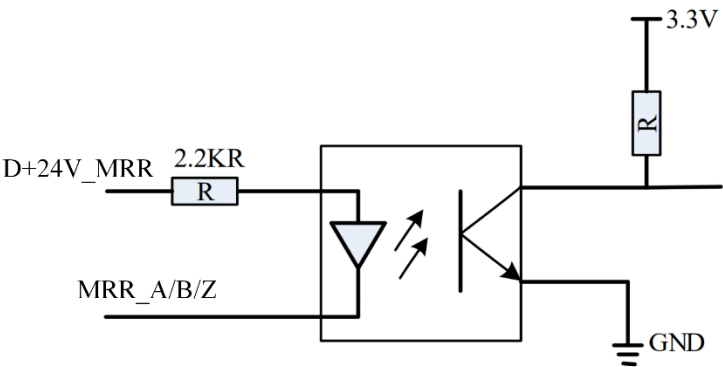
图 21-9 磁栅尺输入电路示意图
