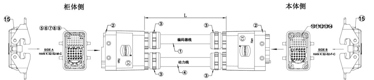
图 9-10 inCube30/inCube32 标准重载线（AIR12SC/AIR20SC 机型）示意图
