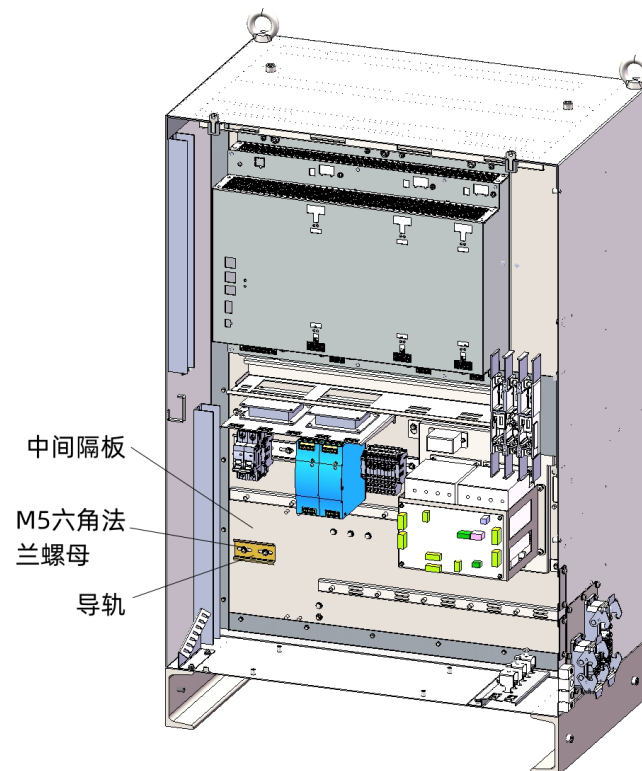
图 18-7 ARC5-280 控制柜安装导轨
