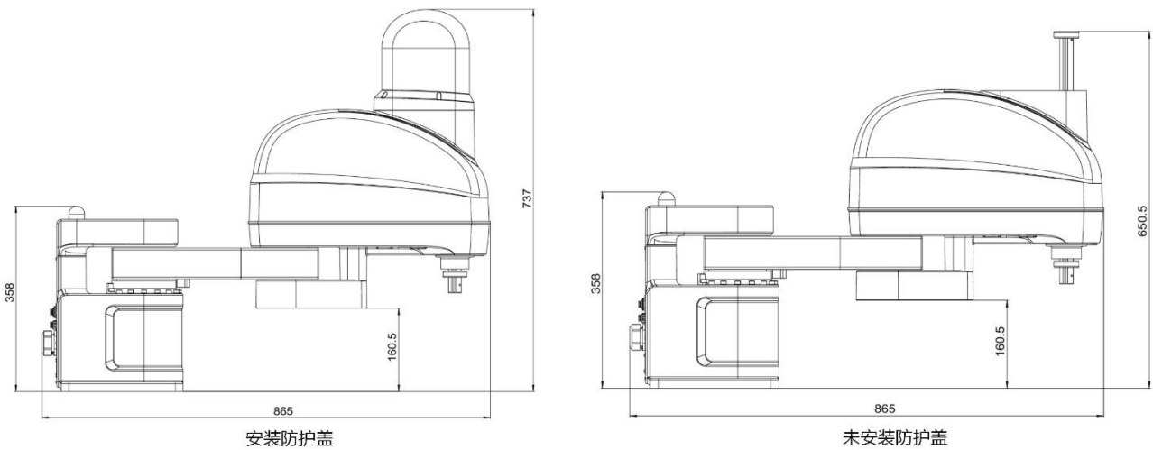
图 4-2 AIR12SC 的 200mm 行程的丝杆防护盖尺寸对比示意图
