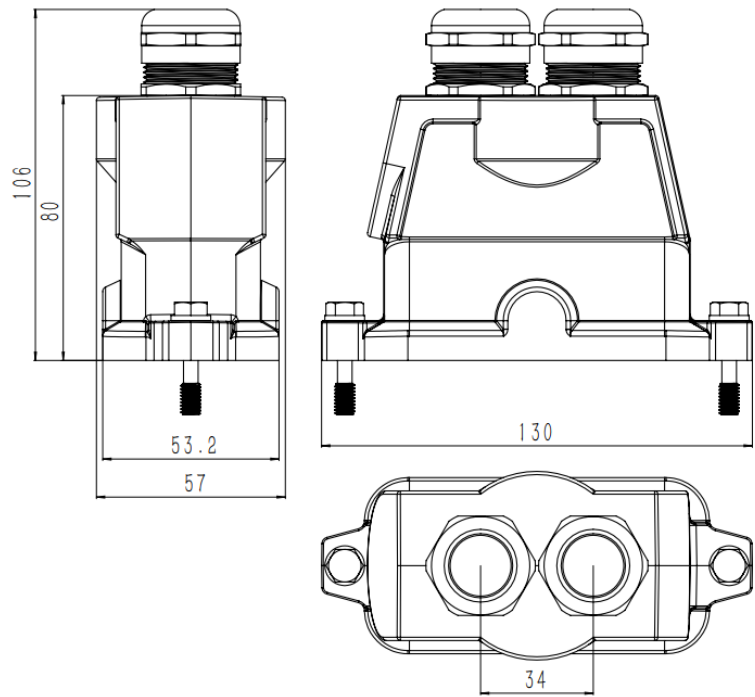
图 9-23 AIR6L-A 本体端重载尺寸图
