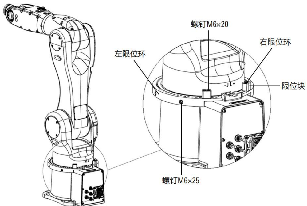
图 6-5 AIR7-920B 安装限位环总览图
