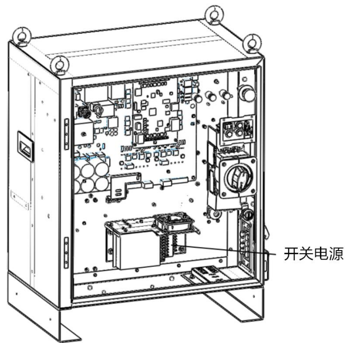
图 20-20 开关电源
