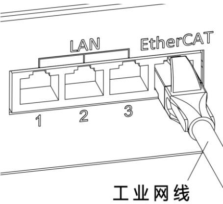
图 12-1 inCube2S 的 EtherCAT 接线
