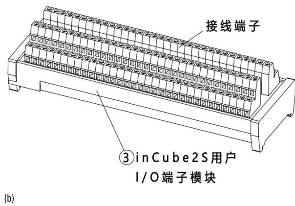
图 19-2 inCube2S 控制柜用户 DI 模块接线示意图
