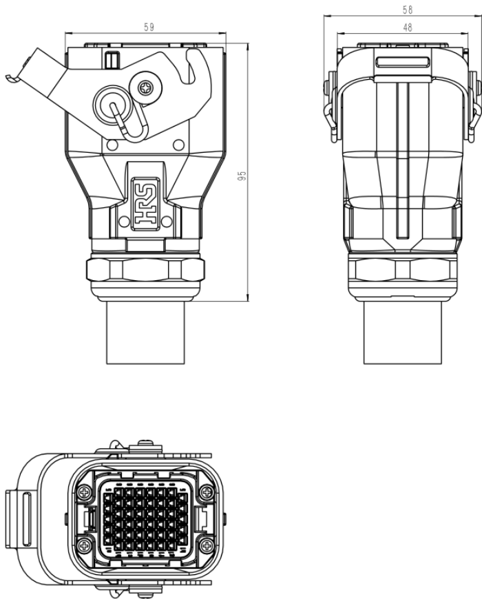
图 9-28 inCube20/2S 重载接头尺寸
