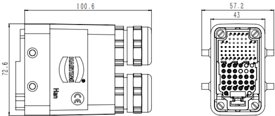
图 9-5 inCube30 重载插头尺寸图
