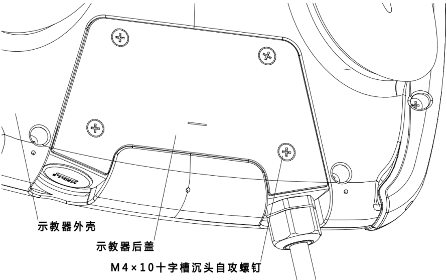
图 10-6 更换示教器外部线束示意图 1
