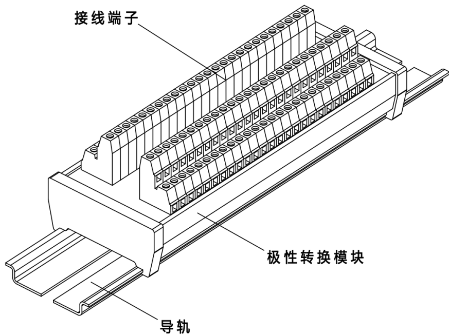
图 23-2 极性转换模块示意图
