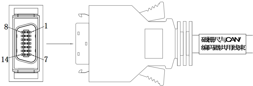
图 21-2 磁栅尺与 CAN_编码器共用线束及 SCSI 引脚示意图
