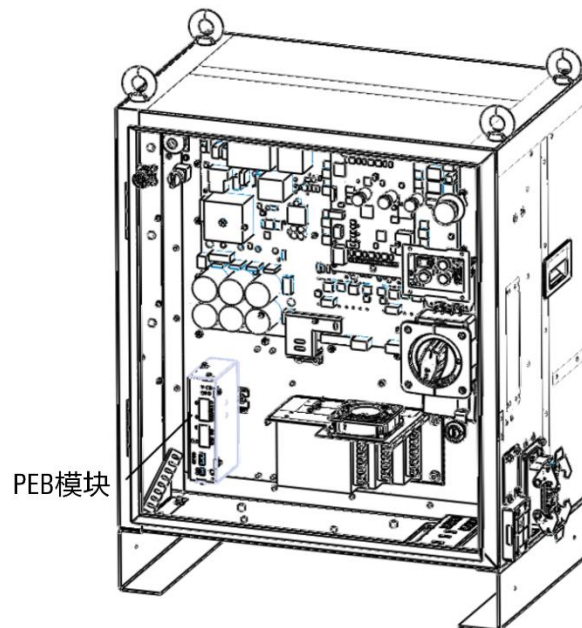
图 16-10 将 PEB 模块安装在导轨上
