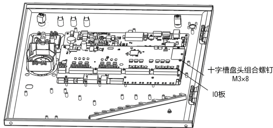
图 20-19 安装 48 路 I0 板
