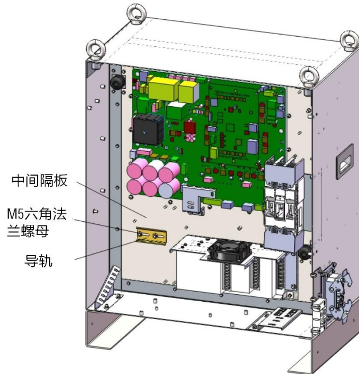
图 18-6 ARC5-12/25 安装导轨
