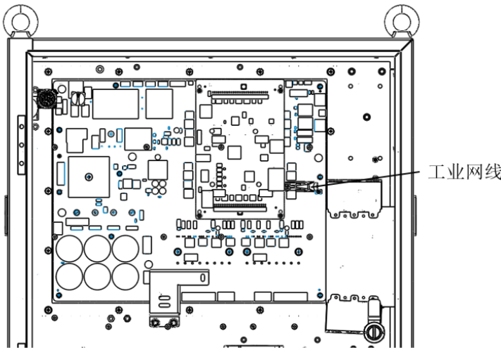
图 12-5 ARC5 的 EtherCAT 接线
