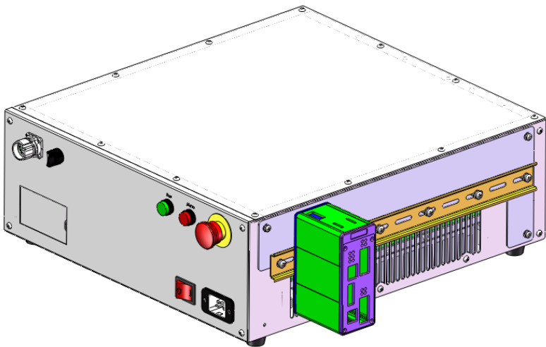
图 18-5 将 EtherNet/IP 模块安装在导轨上
