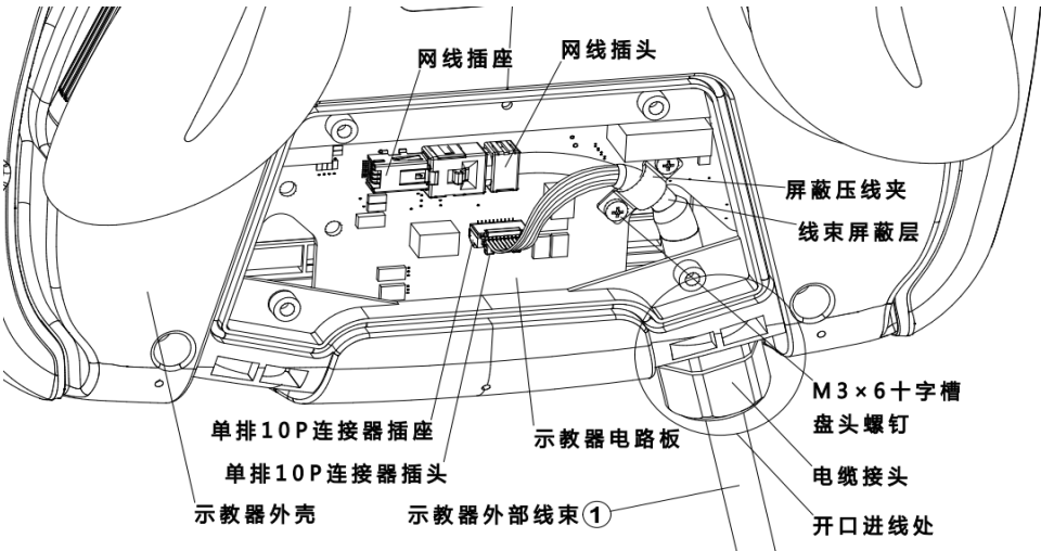
图 10-10 更换示教器外部线束示意图 2
