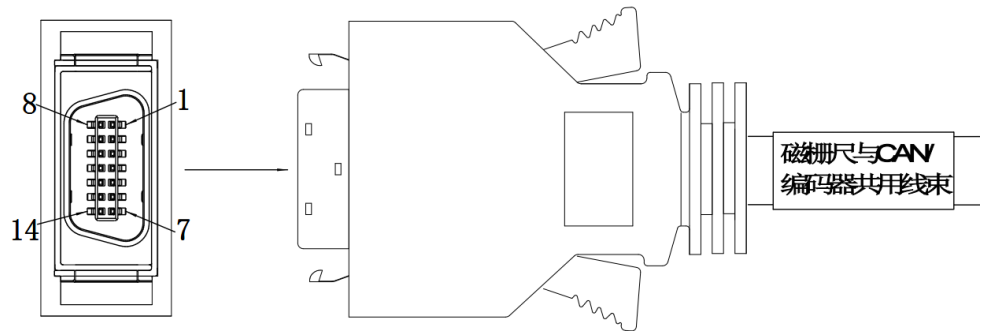
图 21-26 磁栅尺与 CAN_编码器共用线束及 SCSI 引脚示意图
