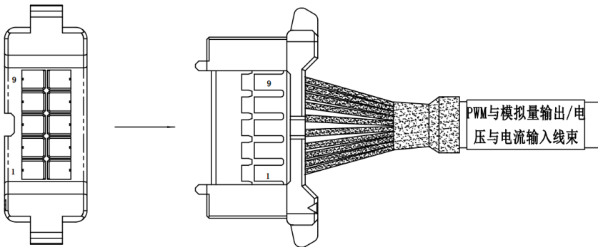
图 21-3 PWM 与模拟量输出_电压与电流输入线束（5m）示意图
