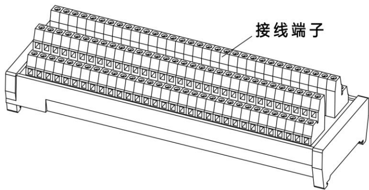
图 19-4 inCube20/22/ARC5 用户 I/O 连接端子台示意图
