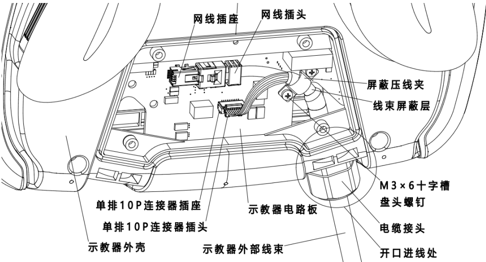
图 10-7 更换示教器外部线束示意图 2
