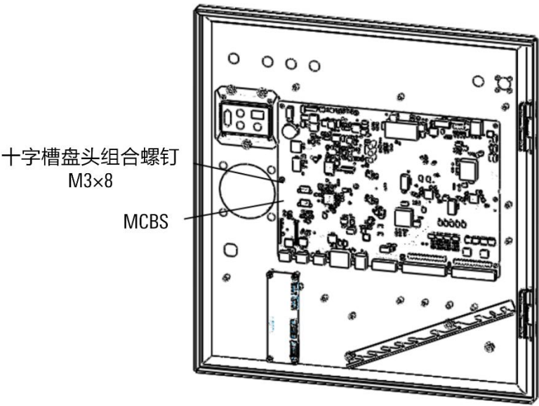
图 21-28 前门 MCBS 示意图
