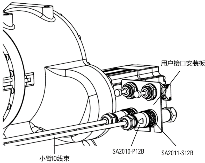
图 5-4 小臂上 I/O 线束连接示意图
