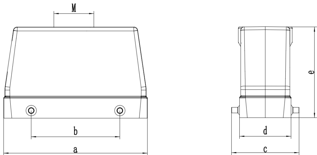
图 9-34 动力线重载接头尺寸
