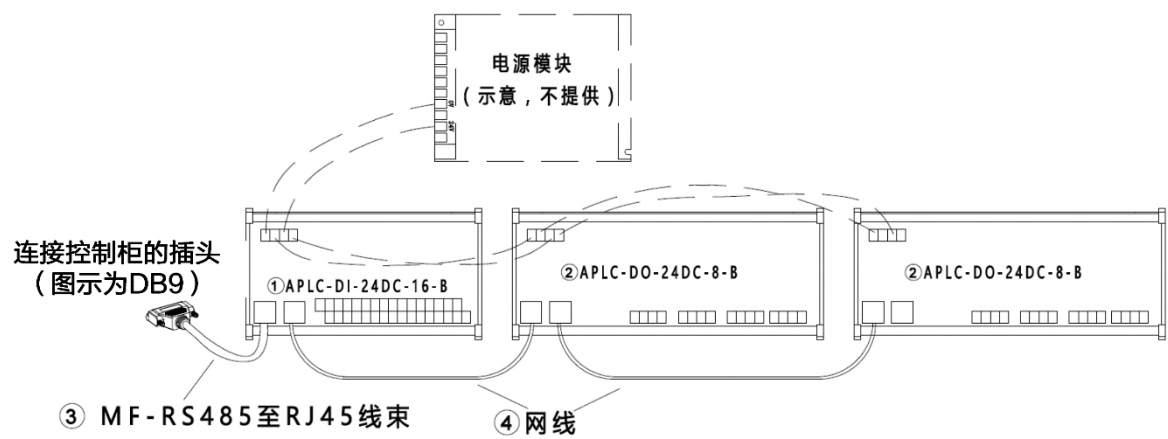
图 20-14 “16 路 DI+16 路 DO” 的连接示意图
