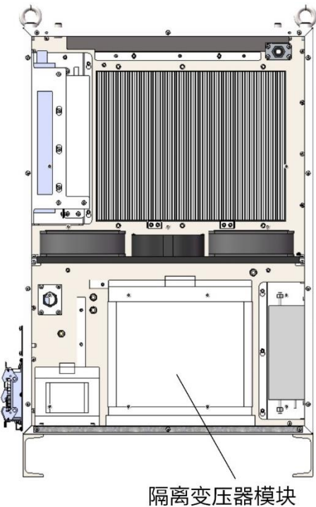
图 7-1 隔离变压器在 ARC5-280 柜内示意图
