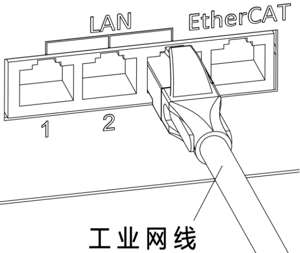
图 14-1 inCube2S 的 Ethernet 接线示意图
