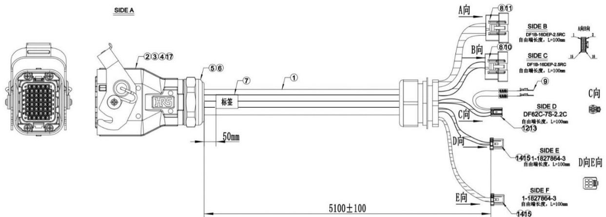
图 9-30 inCube2S-20 拖链重载线示意图
