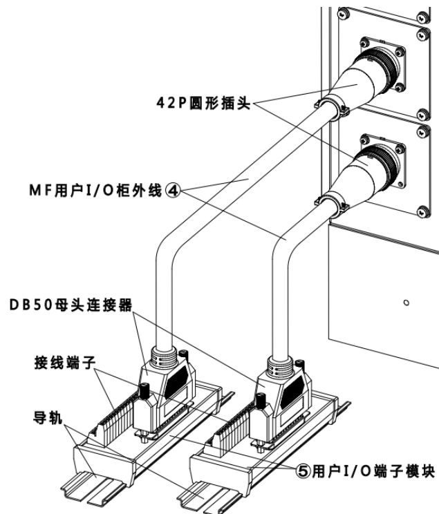
图 19-14 连接用户 I/O 端子模块
