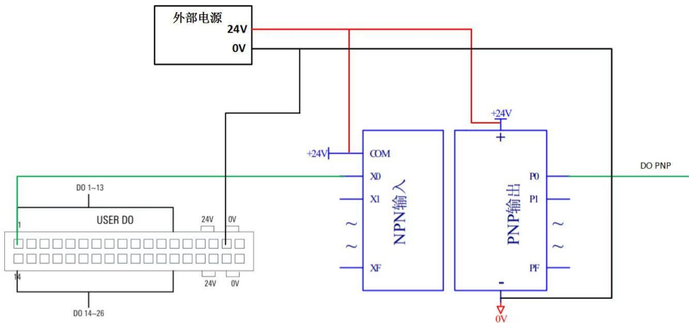
图 22-2 极性转换模块连接示意图
