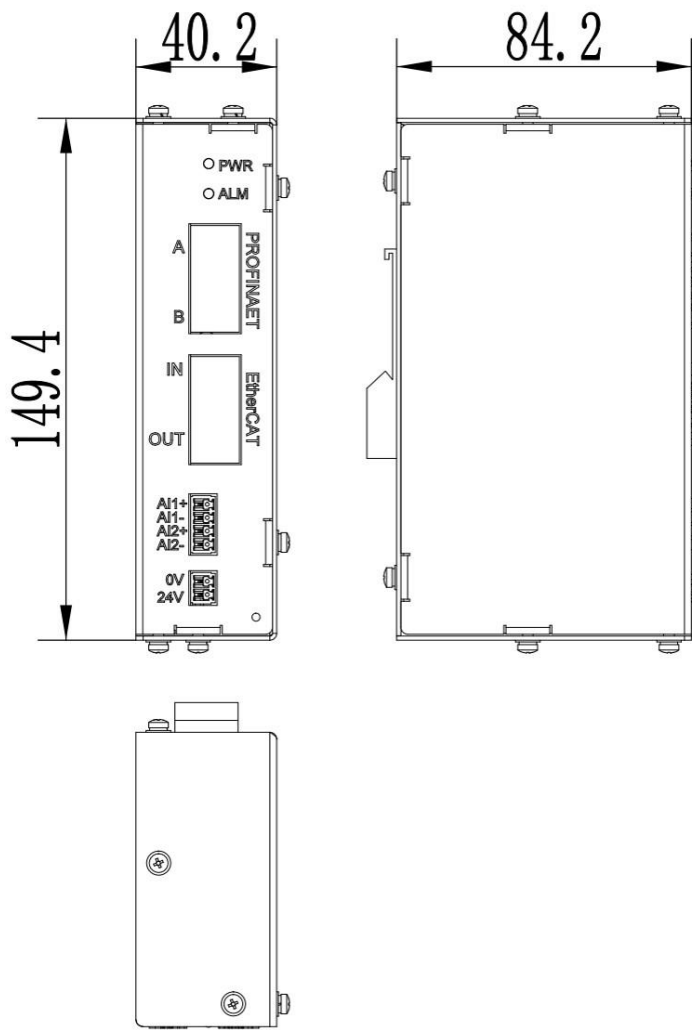
图 16-2 PEB 模块尺寸图
