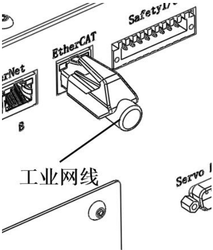
图 12-2 inCube /22 的 EtherCAT 接线
