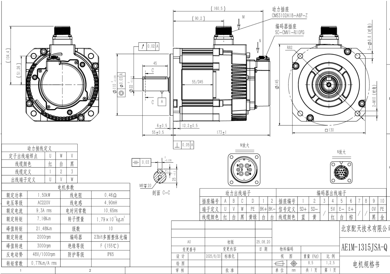
图 28-11 AE1M-1315JSA-Q 电机图纸
