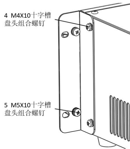
图 24-1 inCube20/22 系列控制柜 19 寸机柜安装支架示意图柜体叠放固定装置
