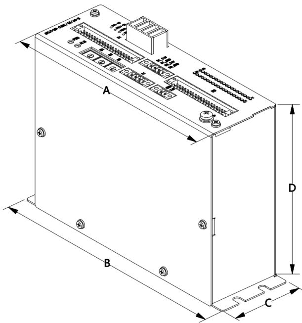
图 19-15 PLC_MF 的外形图
