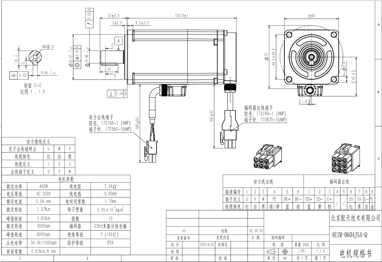
图 28-5 AE1M-0604JSA-Q 电机图纸
