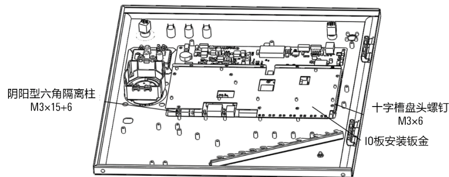
图 20-18 安装 I0 板安装板
