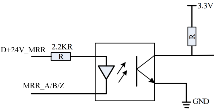
图 21-21 磁栅尺输入电路示意图
