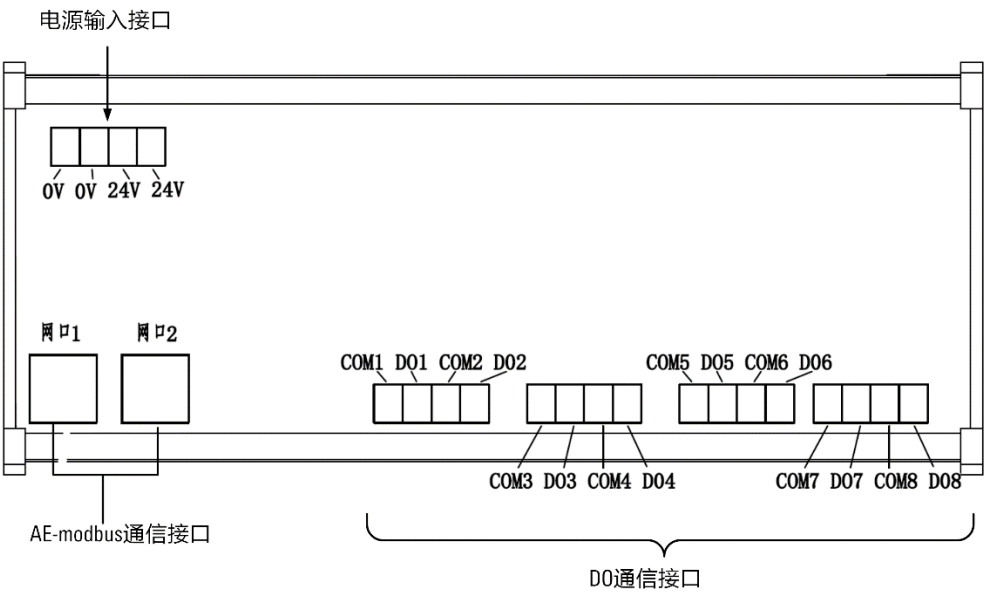
图 20-13 BD0 模块接口示意图
