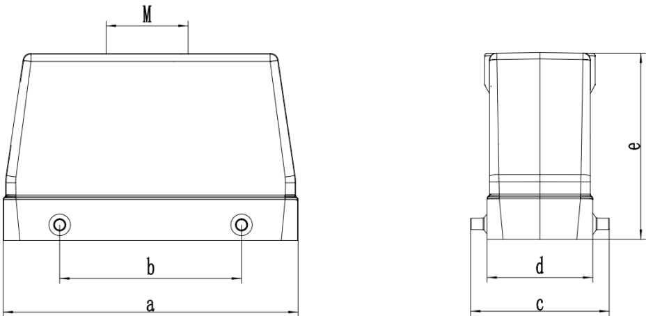
图 9-14 动力线重载接头尺寸
