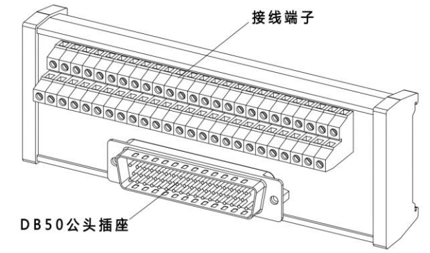
图 19-9 用户 I/O 端子模块
