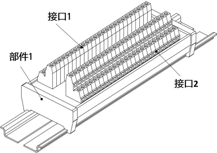
图 23-1 PNP/NPN 极性转换模块接口示意图
