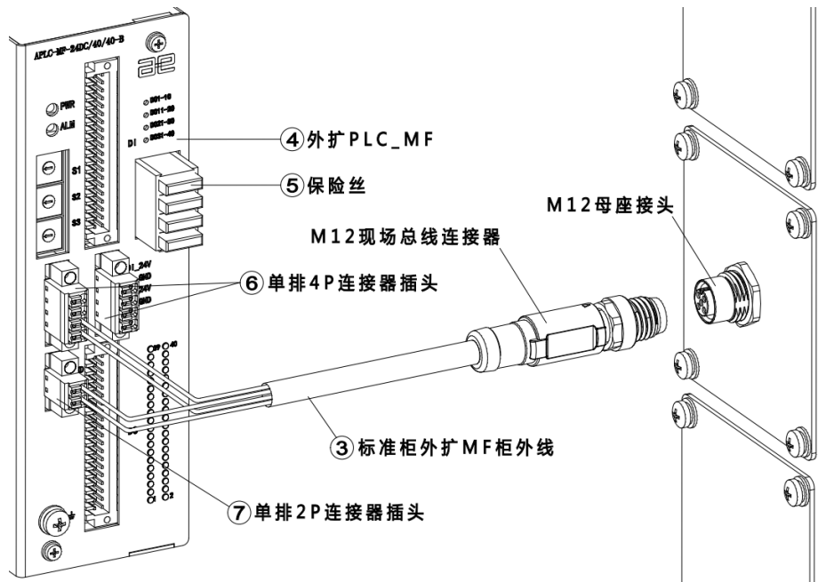
图 20-10 连接外扩 PLC_MF 示意图
