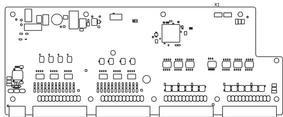
图 20-22 连接 BDIO-48IN-48OUTPCBA 示意图
