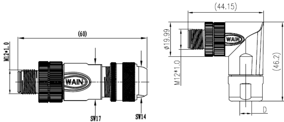
(c) 直管航插与弯管航插的外形尺寸
