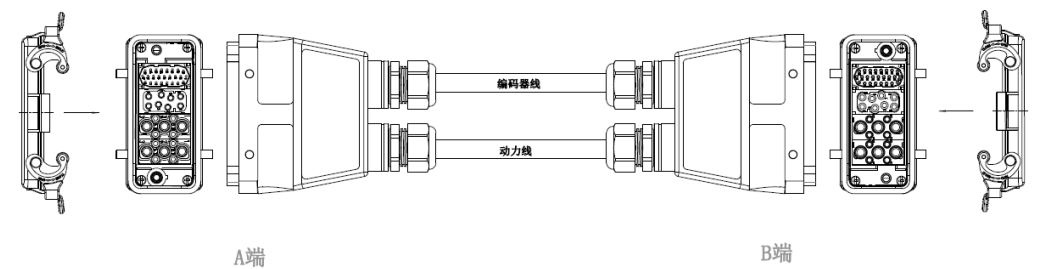
图 9-7 inCube22 标准重载线示意图
