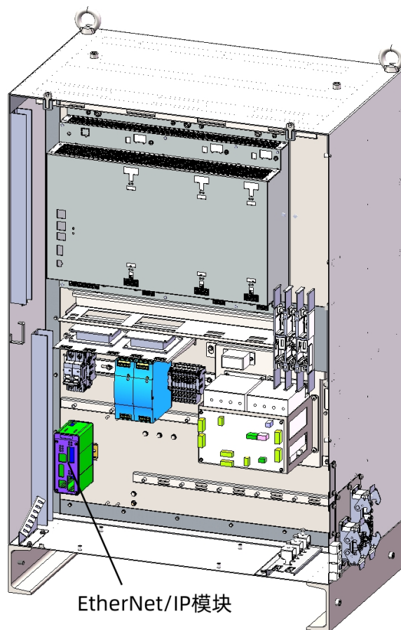
图 18-9 ARC5-280 控制柜安装 EtherNet/IP 模块
