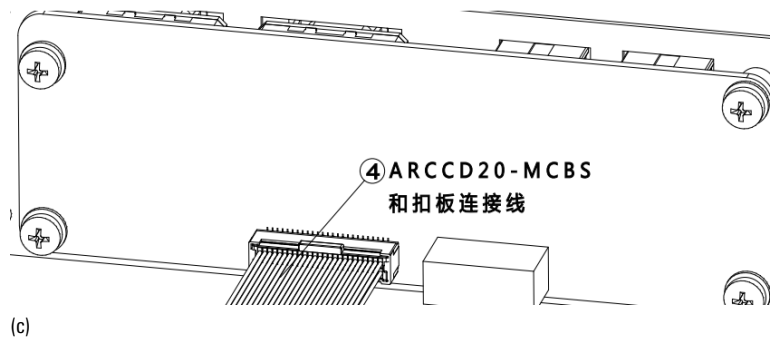
图 21-18 安装 ARCCD20-MCBS 和扣板连接线
