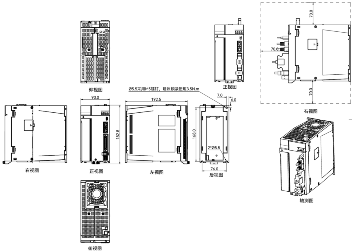
图 3-4 A2E(P)-120(170)TI-H 型号驱动器尺寸图
