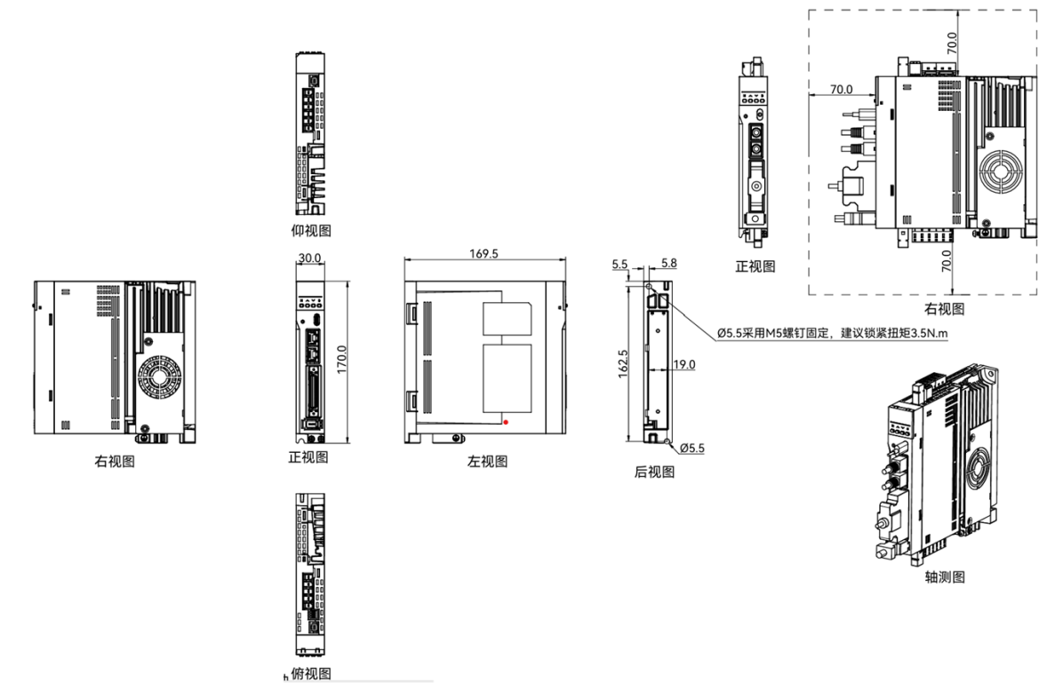
图 3-3 A2E(P)-5R4AI-H 型号驱动器尺寸图
