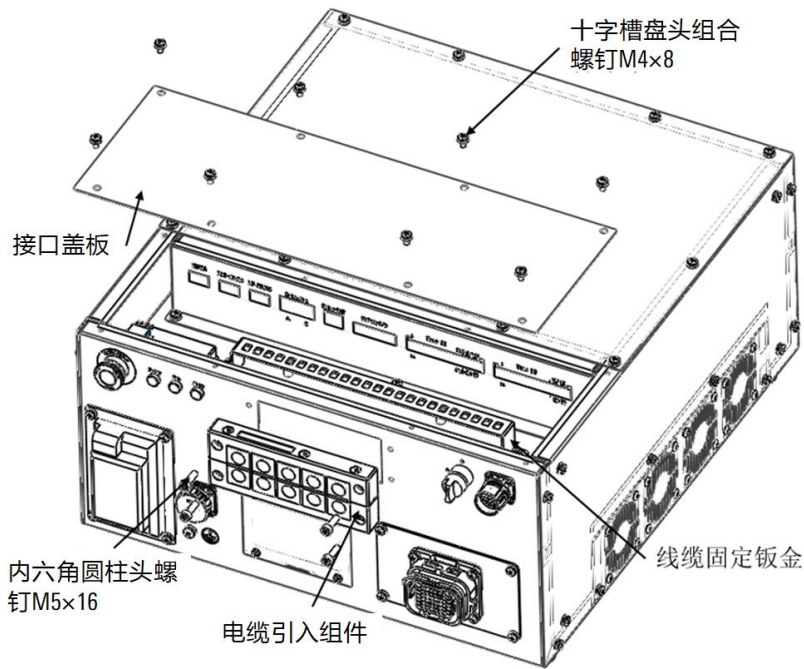
(a) Safety I/O 接口接线示意图
