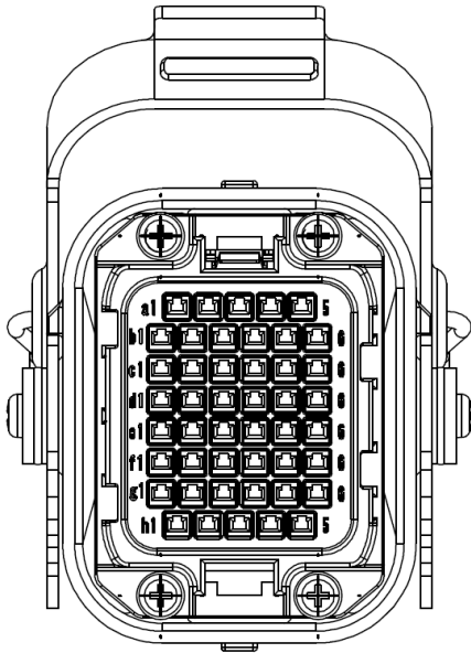
图 4-7 inCube20-HP 型控制柜重载接口定义
