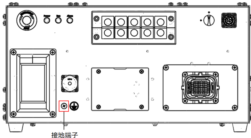
图 6-1 inCube20-HP 型控制柜地线接入点示意图
