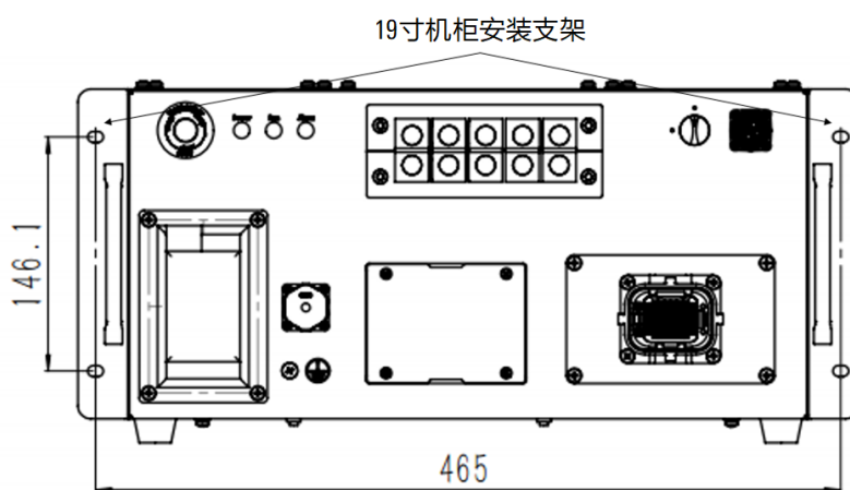
图 4-2 19 寸机柜安装图
