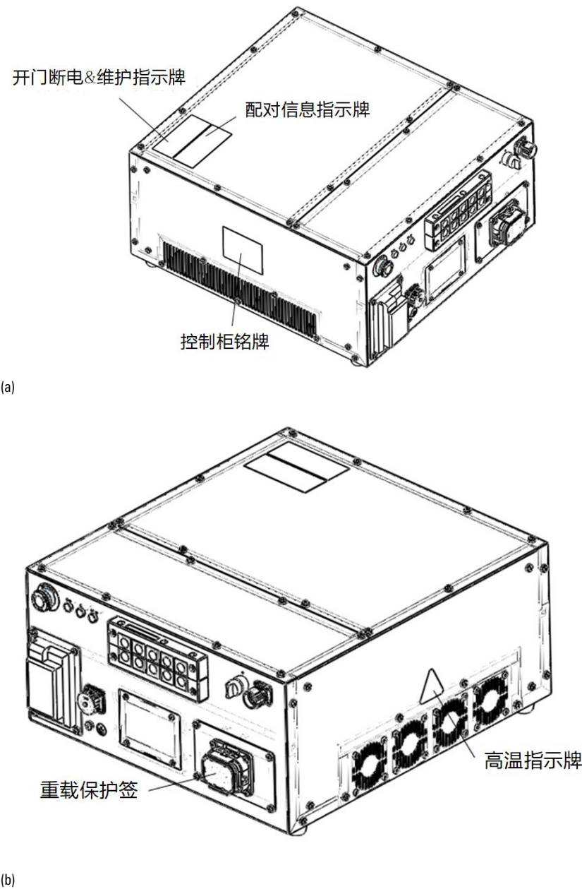
图 1-5 控制柜所含标签位置示意图
