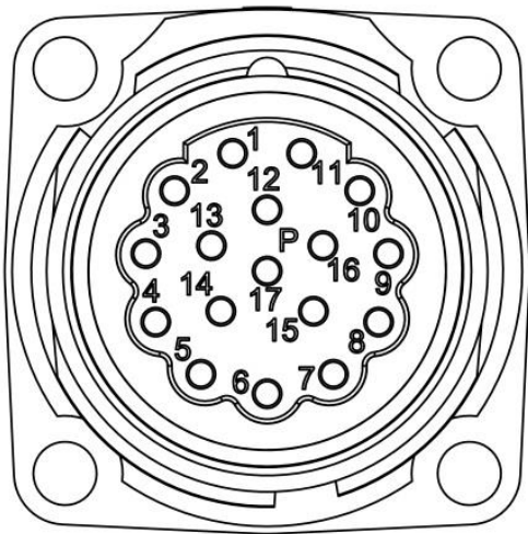
图 4-6 示教器接口
