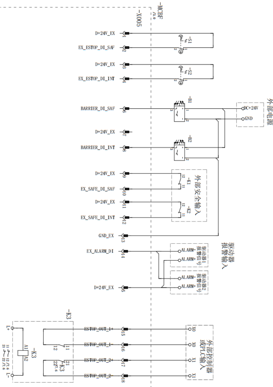
图 5-3 Safety IO 输出信号
