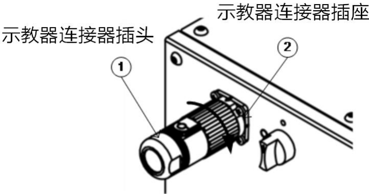
图 4-4 示教器连接
