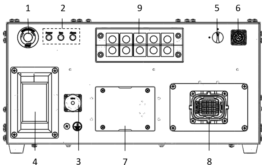
图 4-3 inCube20-HP 各接口所在位置示意图
