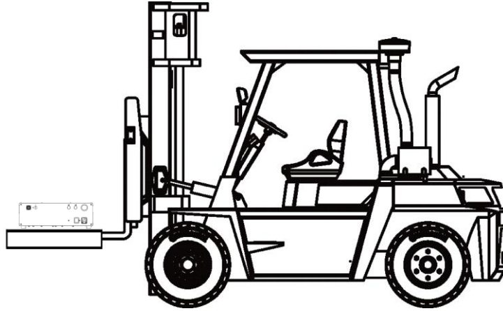
图 2-1 控制柜叉车搬运示意图
