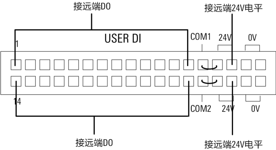
图 5-5 User DI 接口使用说明（NPN 输入）
