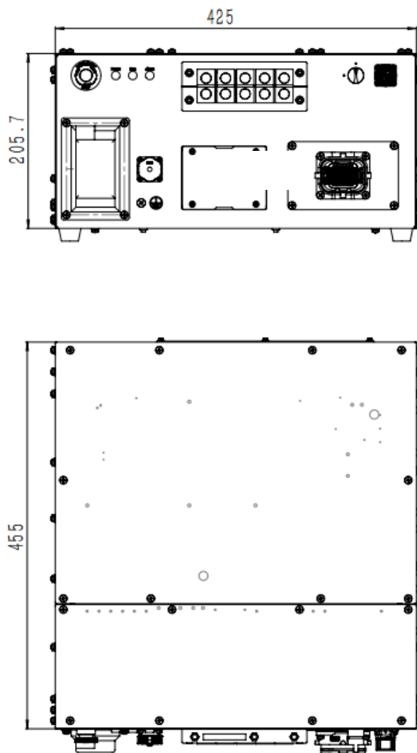
图 4-1 机柜外形尺寸图
