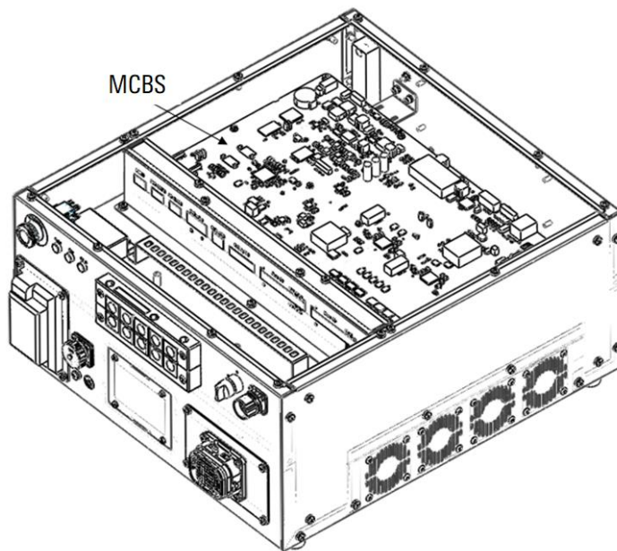
图 1-3 上腔内部器件示意图
