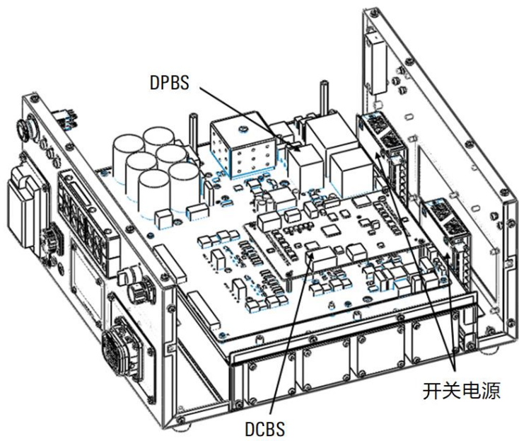
图 1-4 下腔内部器件示意图
