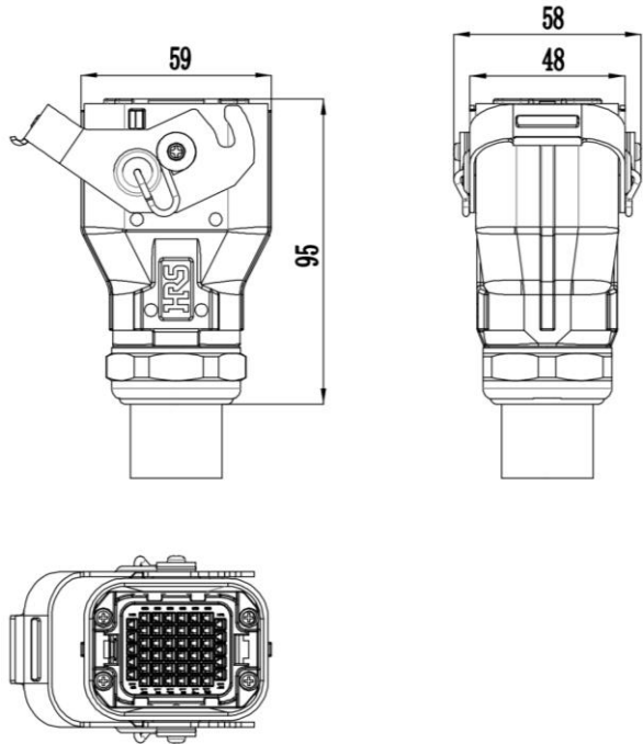
图 4-5 重载插头尺寸图
