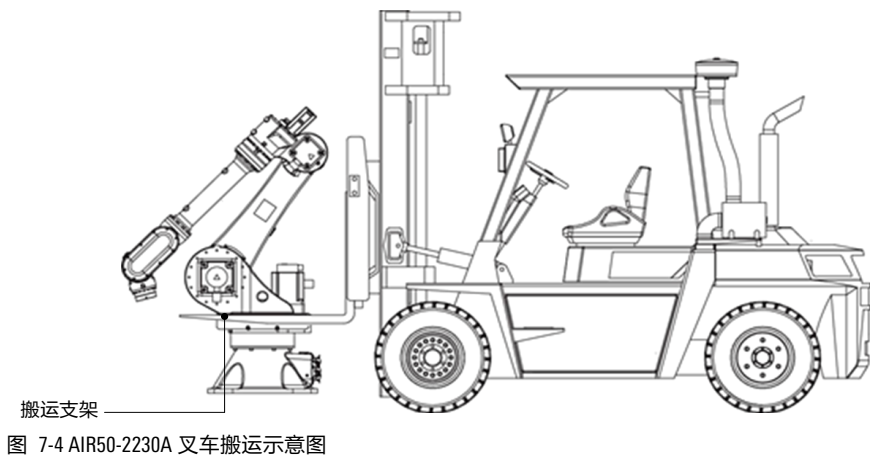
图 7-4 AIR50-2230A 叉车搬运示意图
