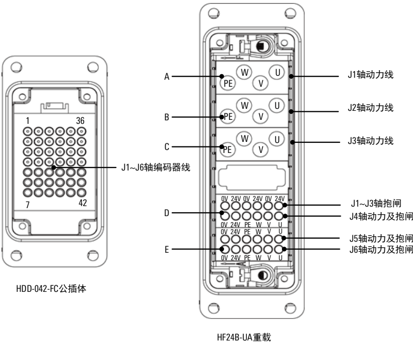
图 4-2 AIR50-2230A 操作机重载接口定义
