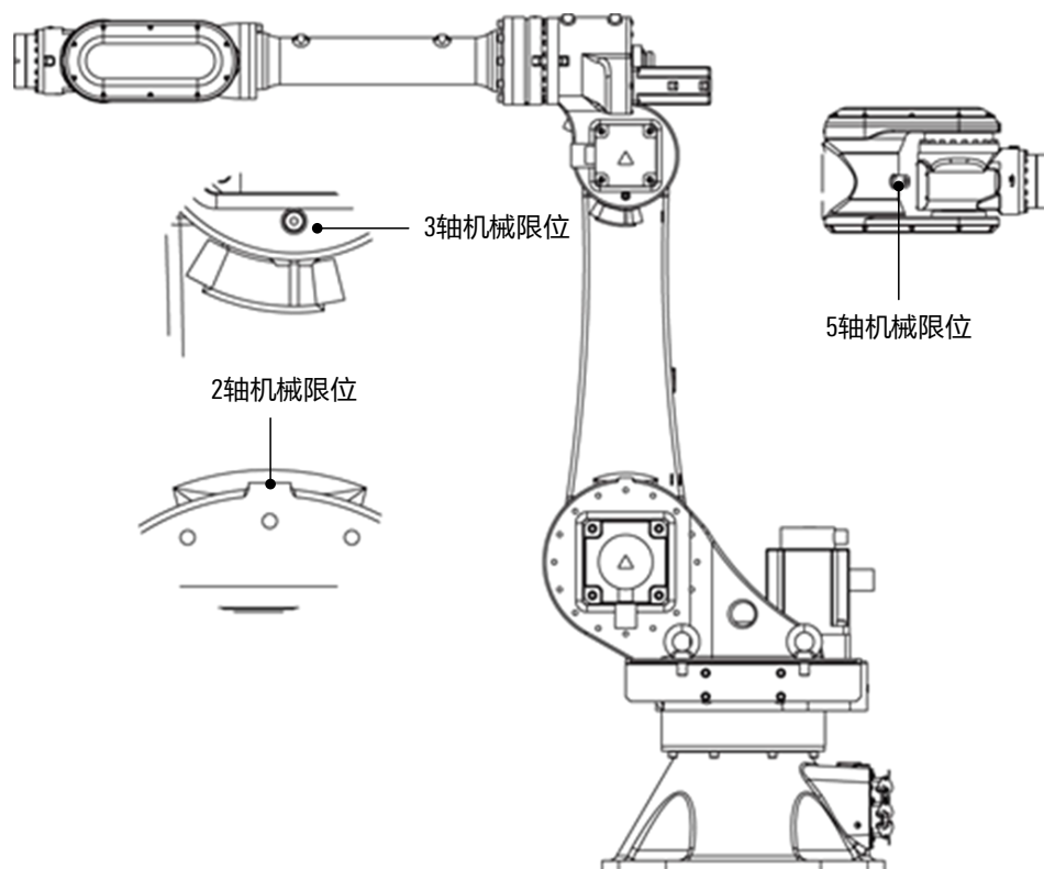
图 6-2 AIR50-2230A 操作机上机械式制动器
