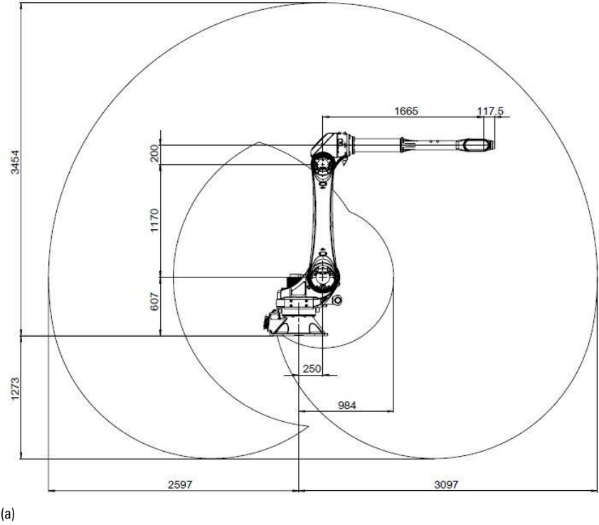
图 7-7 AIR35-2700 操作机工作范围
