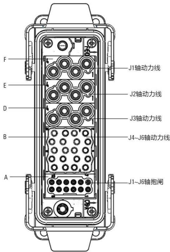
图 5-4 中负载操作机动力重载连接器
