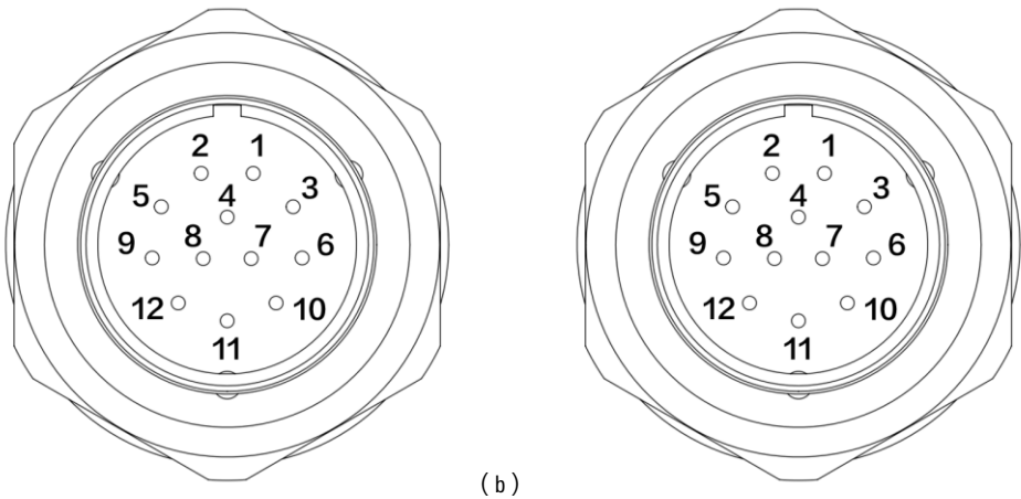
图 5-6 中负载操作机底座 I0 航插接口（左）及小臂 I0 航插接口（右）
