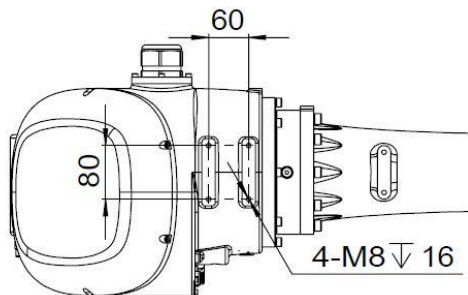
图 7-19 操作机肘部负载接口尺寸示意图
