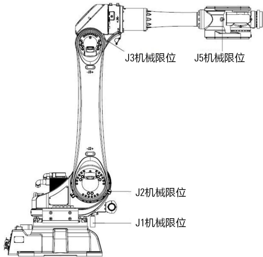
图 7-10 AIR50-2700/AIR80-2560 操作机上机械式制动器
