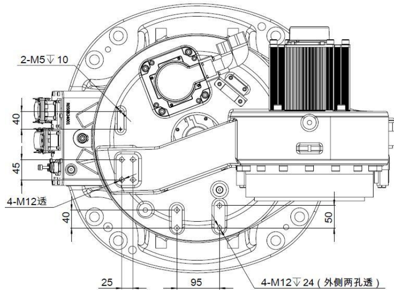
图 7-24 AIR50-2260/AIR80-2260/AIR35-2700/AIR20-3100 操作机肩部接口尺寸图
