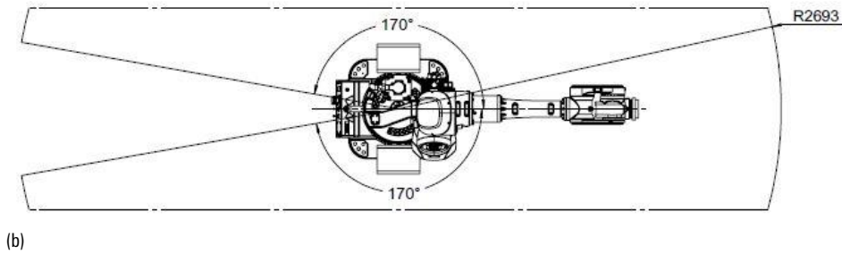
图 7-6 AIR50-2700 操作机工作范围
