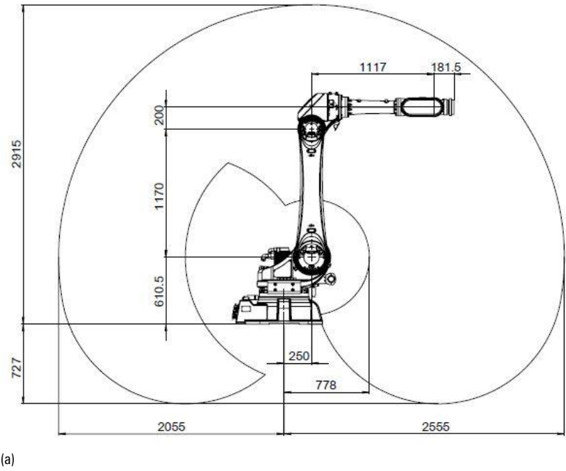
图 7-4 AIR50-2260/AIR80-2260 操作机工作范围
