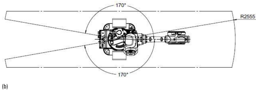
图 7-5 AIR80-2560 操作机工作范围
