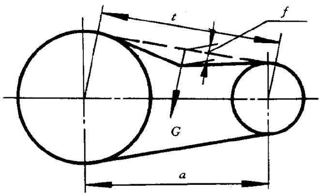
图 12-25 同步带安装挠度
