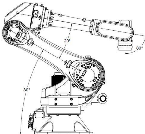
图 9-2 AIR50-2260/AIR80-2260 操作机搬运位姿图
