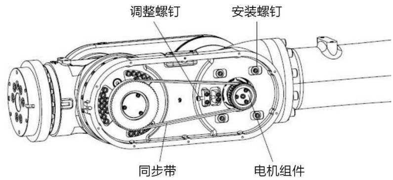
图 12-22 AIR80-2260/AIR80-2560 拆卸同步带
