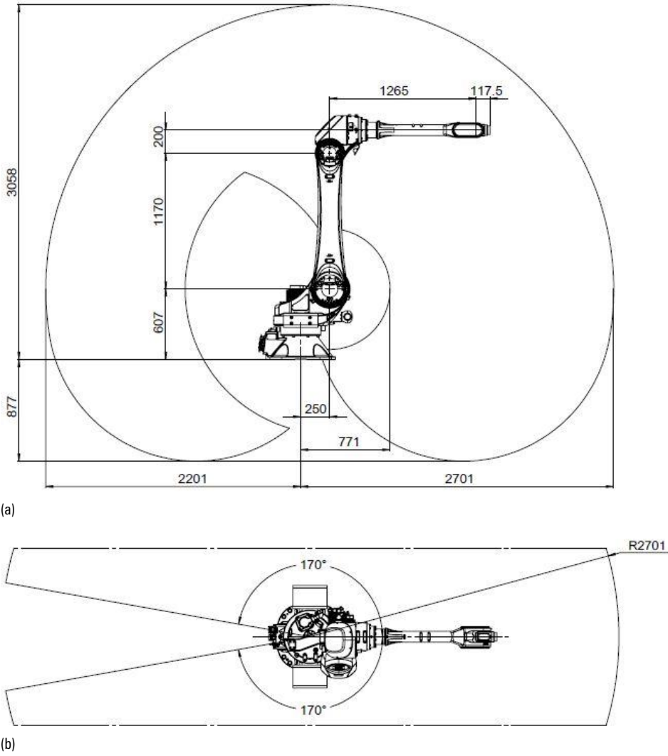
图 7-7 AIR35-2700 操作机工作范围
