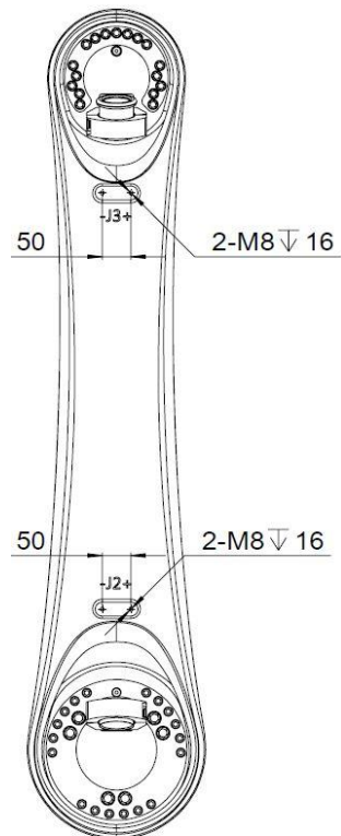
图 7-23 AIR80-2560/AIR50-2700/AIR35-2700/AIR20-3100 操作机大臂接口尺寸图
