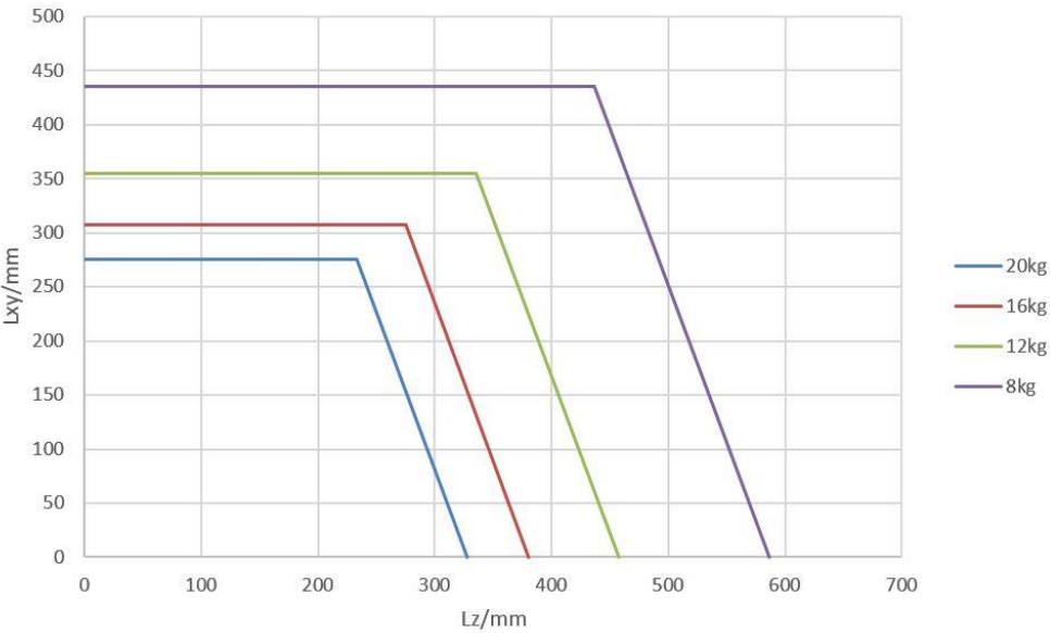
图 7-18 AIR20-3100 腕部负载质心位置示意图
