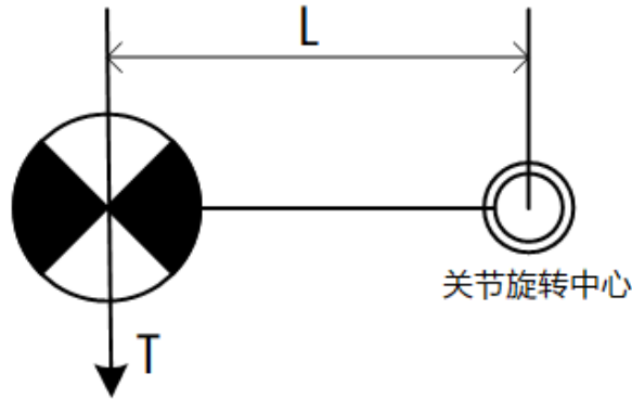
图 7-14 负载离心率示意图
