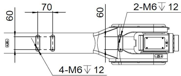
图 7-21 AIR35-2700/AIR20-3100 操作机小臂接口尺寸图
