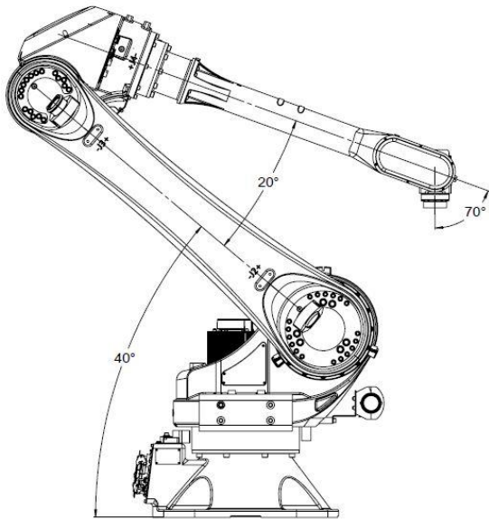
图 9-5 AIR35-2700 操作机搬运位姿图
