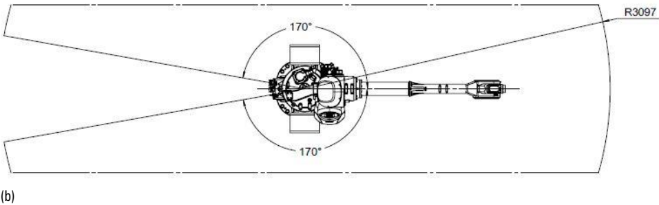
图 7-8 AIR20-3100 操作机工作范围
