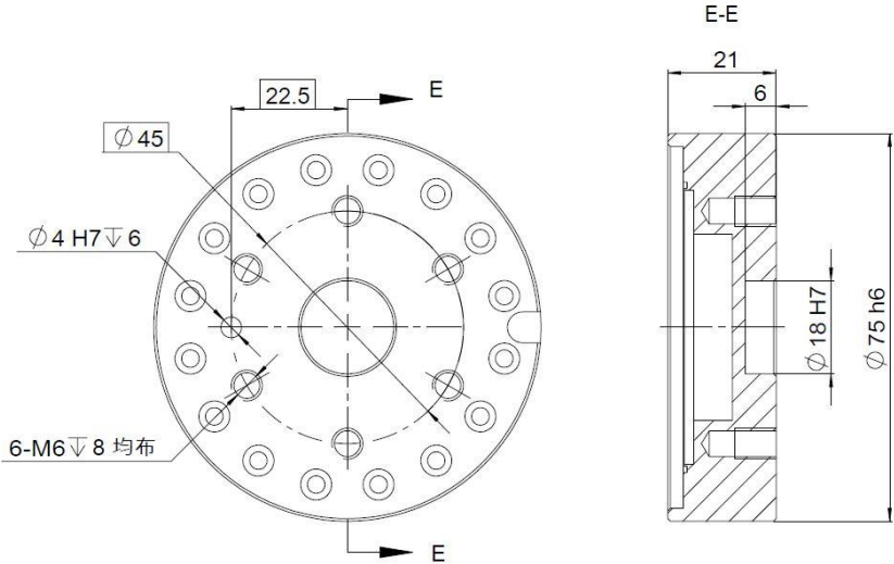
图 7-13 AIR35-2700/AIR20-3100 操作机腕部法兰尺寸示意图
