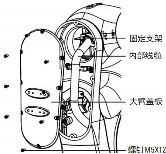
图 12-4 大臂内部线缆检修
