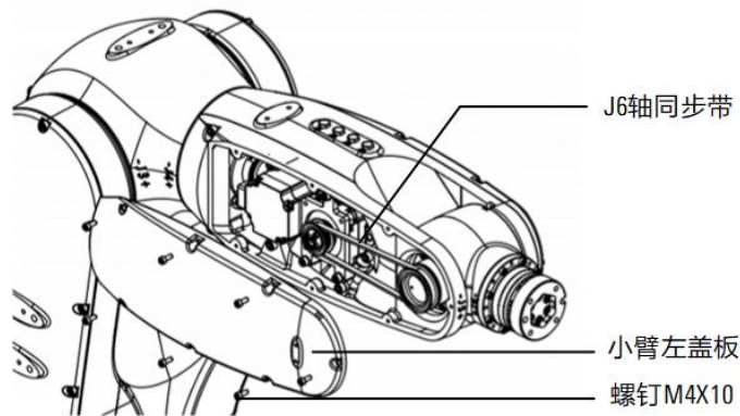
图 12-12 拆卸小臂左盖板
