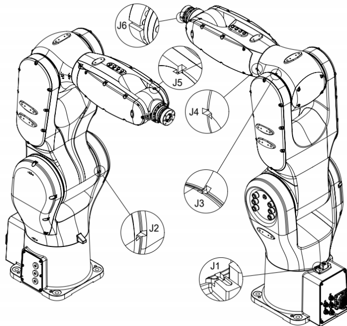
图 8-16 轴操作机各轴零点示意图
