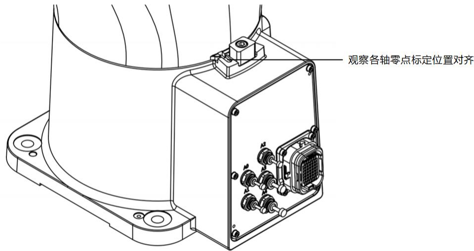
图 8-3 6 轴机器人肉眼观察零点标定方式
