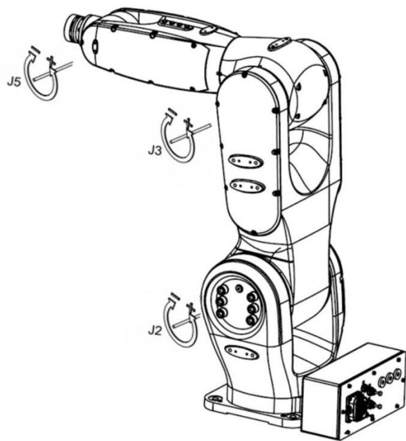
图 7-2 4 轴操作机各轴运动方向
