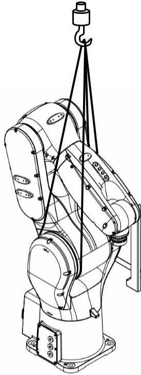
图 9-8 6 轴机器人吊环搬运示意图
