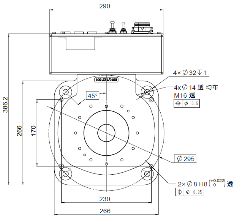
图 4-2 3/4 轴机器人操作机基座接口尺寸
