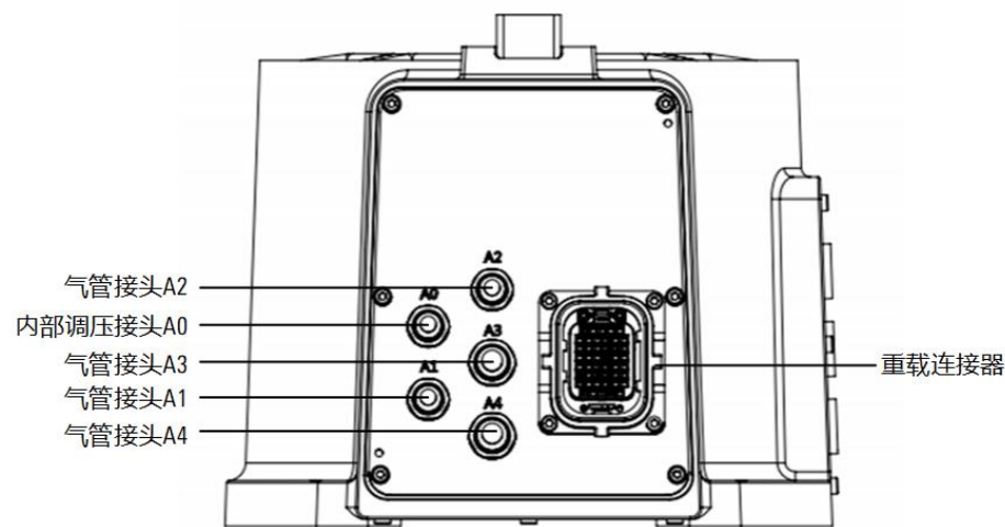
(a) 后视图
