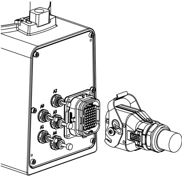
图 6-6 6 轴操作机侧重载线连接接口
