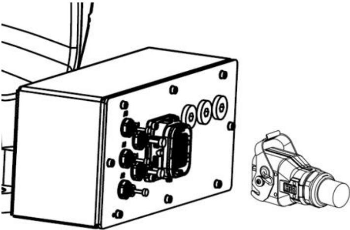
图 6-7 3/4 轴操作机侧重载线连接接口
