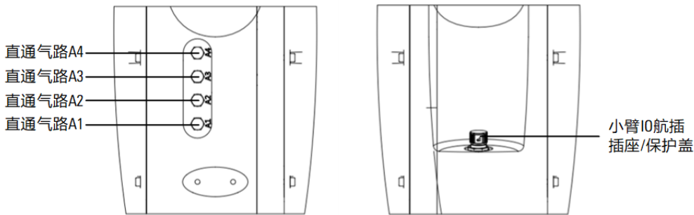
图 5-3 操作机小臂上接口
