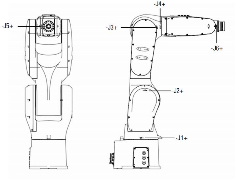
图 2-3 6 轴操作机上各轴方向标识
