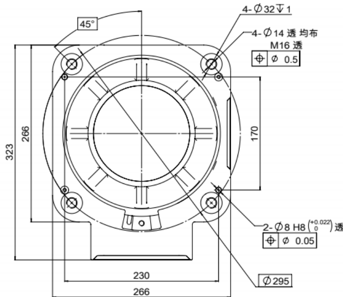
图 4-16 轴机器人操作机基座接口尺寸
