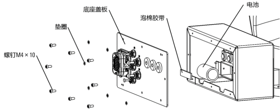
图 12-6 更换电池示意图
