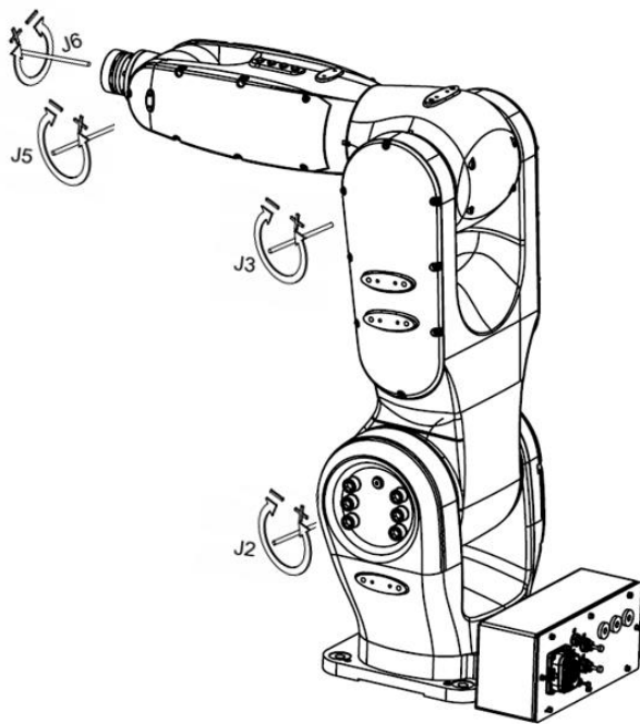
图 7-3 4 轴操作机各轴运动方向
