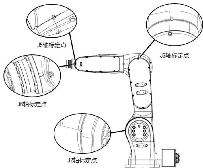
图 8-2 3/4 轴操作机各轴零点示意图
