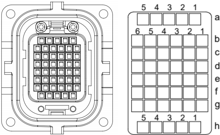
图 5-4 操作机重载接口
