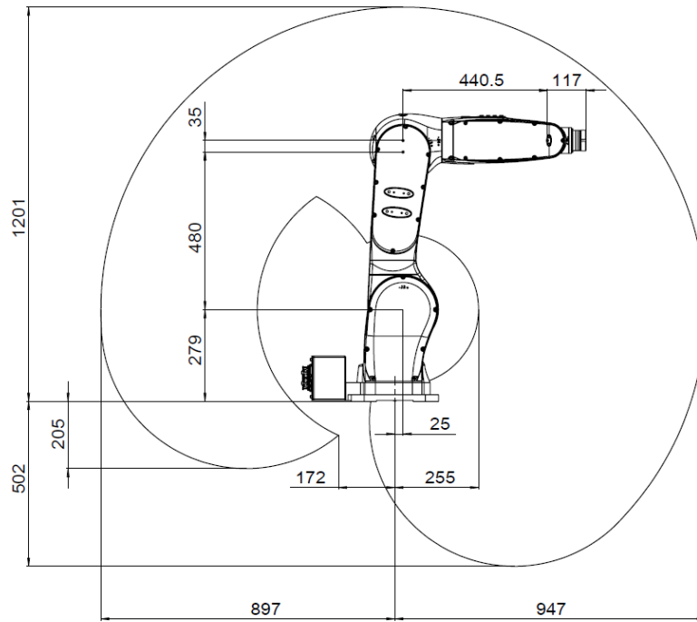
图 7-5 3/4 轴操作机工作范围
