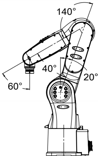
图 9-2 6 轴操作机搬运位姿图
