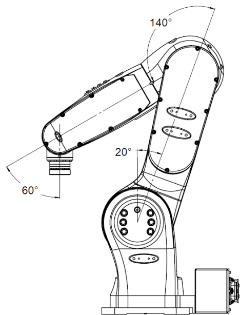
图 9-3 3/4 操作机搬运位姿图
