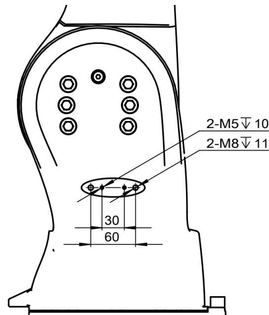
图 7-14 操作机肩部接口尺寸图
