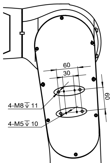
图 7-13 操作机大臂接口尺寸图
