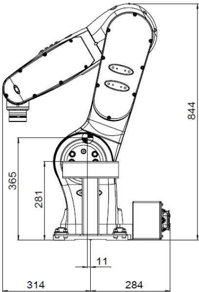
(a) 右视图
