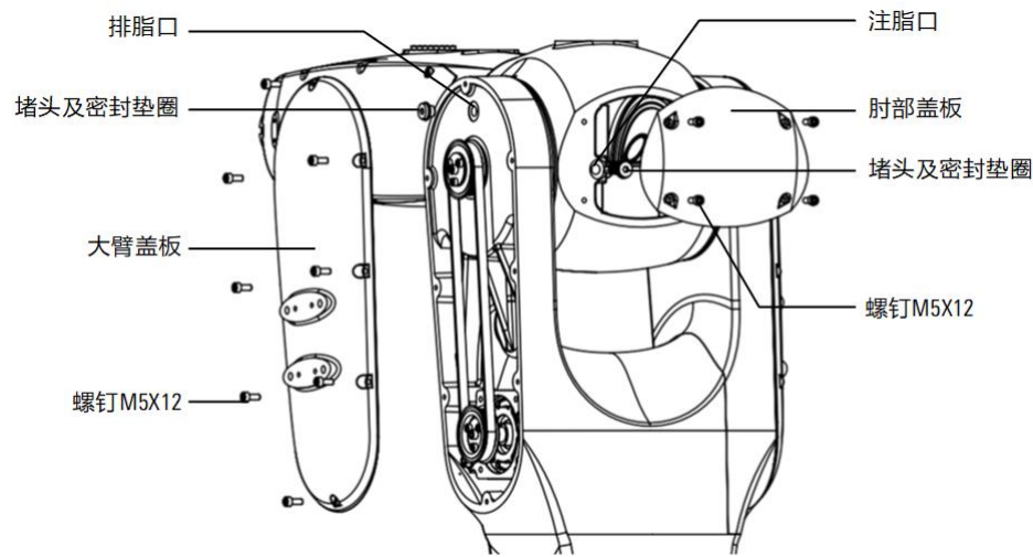
图 12-8 更换 J3 轴减速器润滑脂
