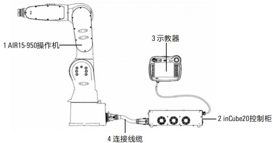
图 1-1 AIR15-950（6 轴）工业机器人系统的构成
