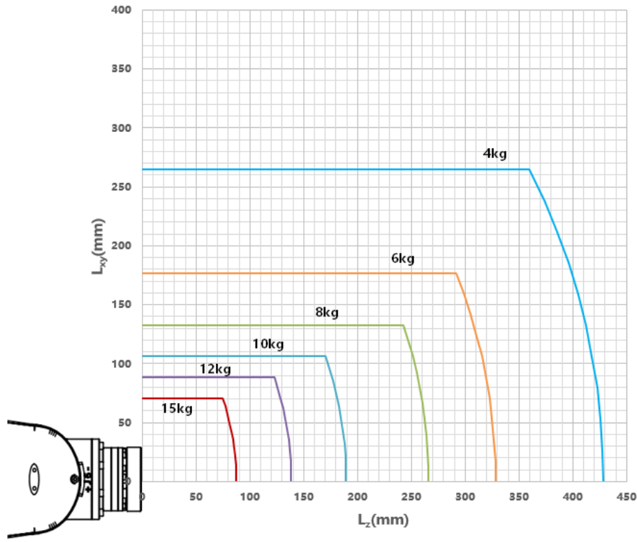
(b) 负载质心位置允许范围示意图
