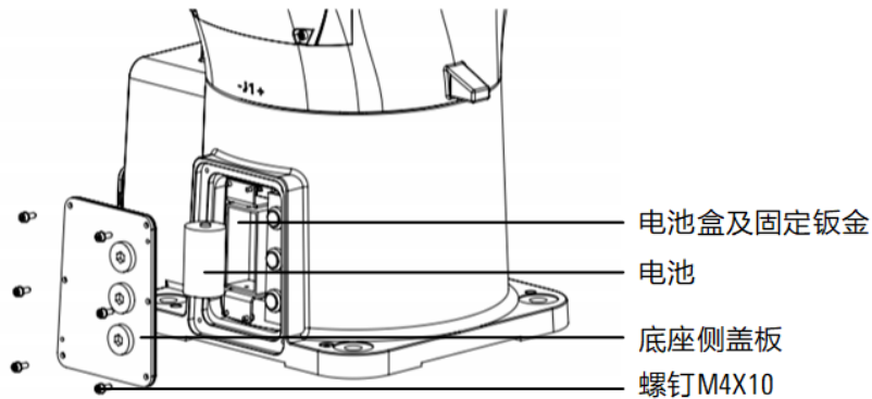
图 12-5 更换电池示意图
