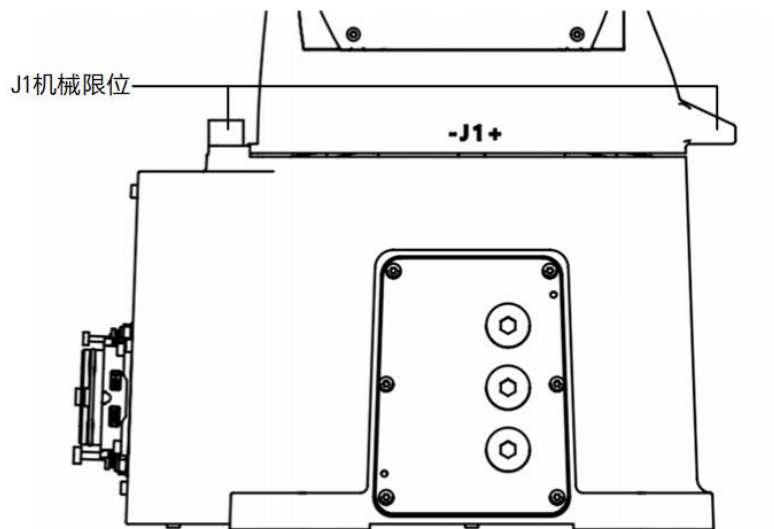
图 7-6 操作机上机械式制动器
