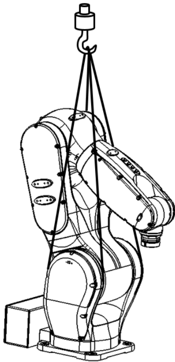
图 9-9 3/4 轴机器人吊环搬运示意图
