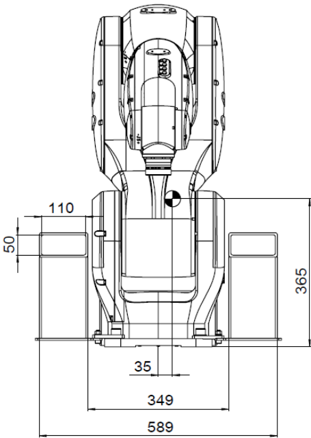
(b) 后视图
