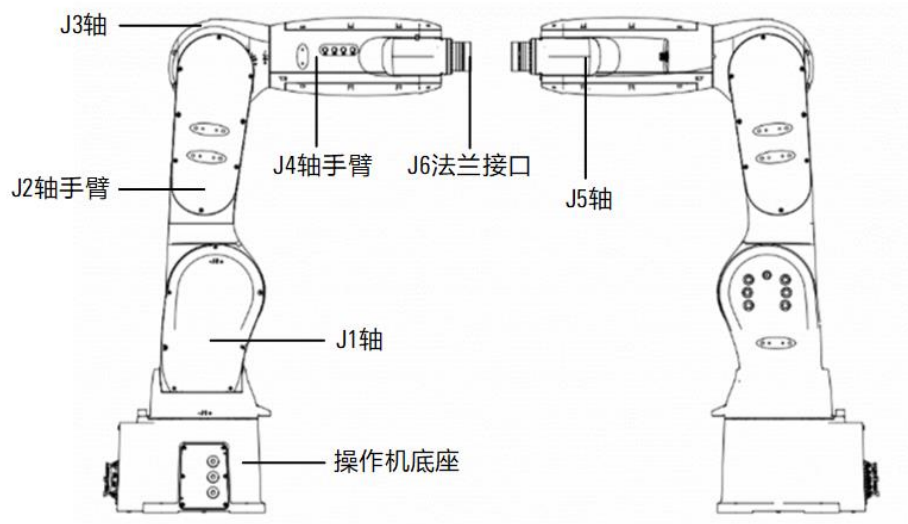
图 1-3 6 轴机器人本体及其各个部分
