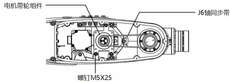
图 12-13 拆卸 J6 轴同步带
