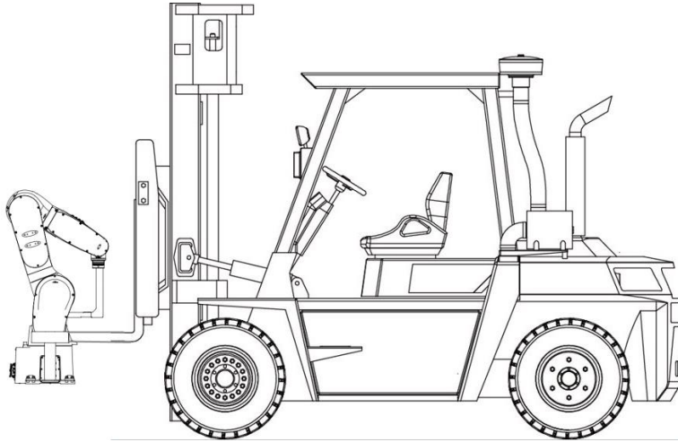
图 9-6 6 轴机器人叉车搬运示意图
