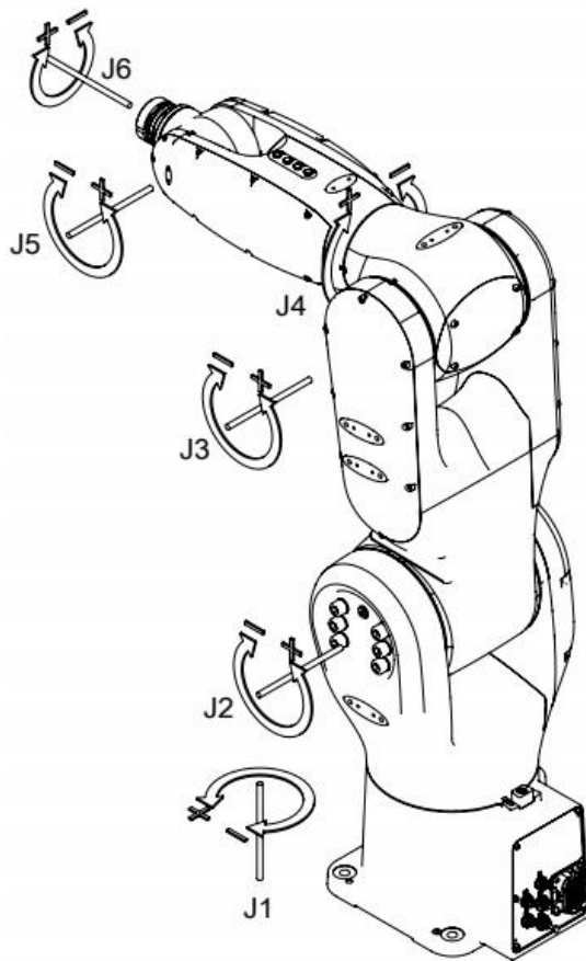
图 7-16 轴操作机各轴运动方向
