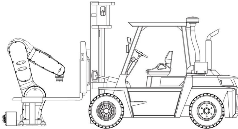
图 9-7 3/4 轴机器人叉车搬运示意图
