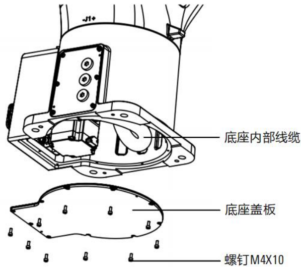
图 12-16 轴底座内部线缆检修
