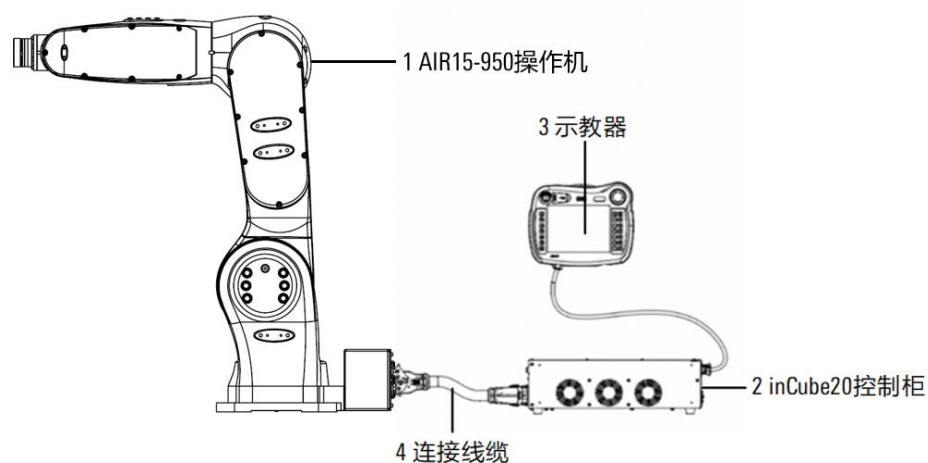
图 1-2 AIR15-950（3/4 轴）工业机器人系统的构成
