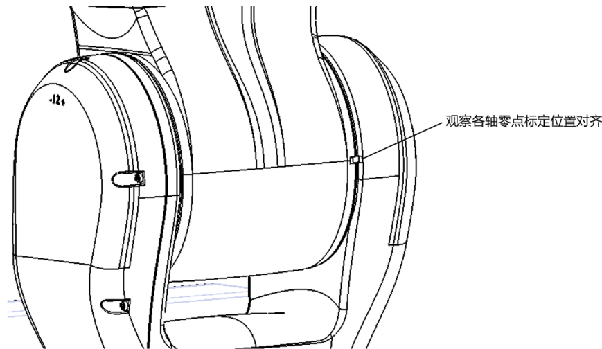
图 8-4 3/4 轴肉眼观察零点标定方式
