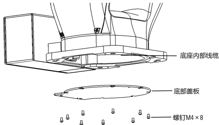
图 12-2 3/4 轴底座内部线缆检修
