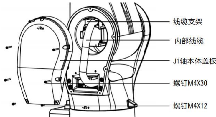
图 12-3 肩部内部线缆检修
