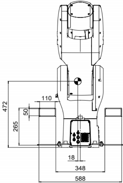
(b) 后视图
