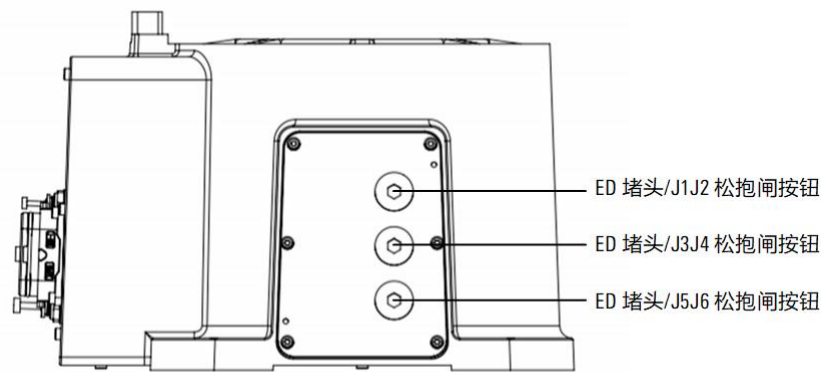
(b) 左视图
