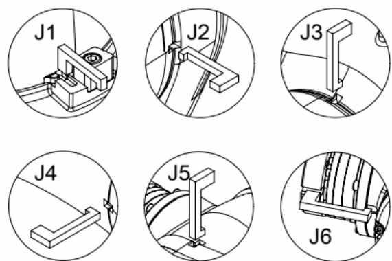
图 8-5 零点标定块标定方式
