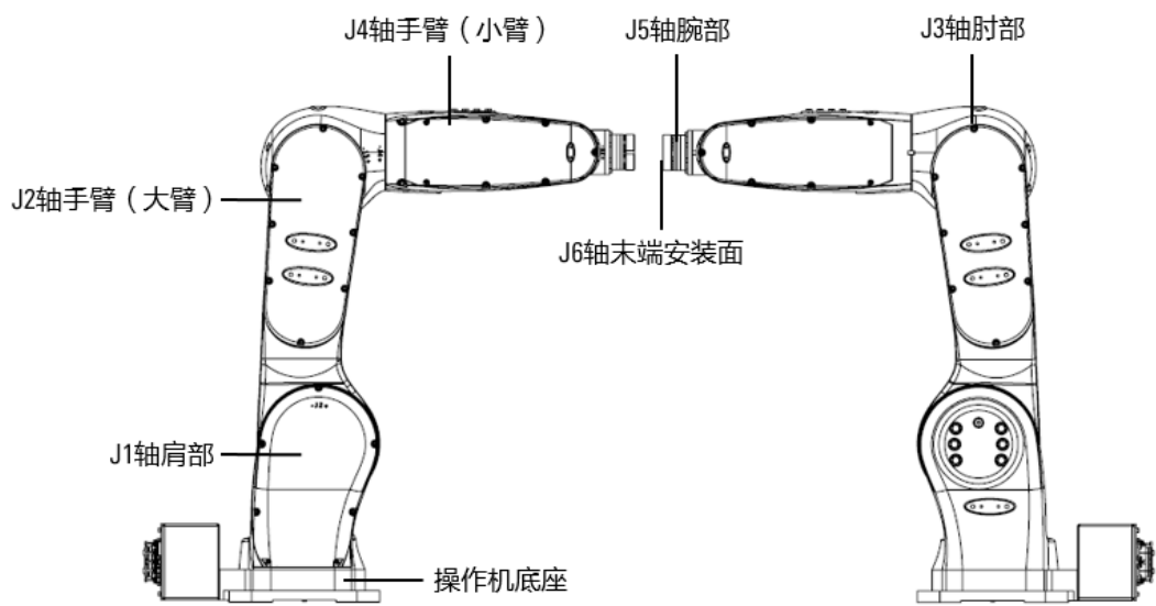
图 1-4 3/4 轴机器人本体及其各个部分
