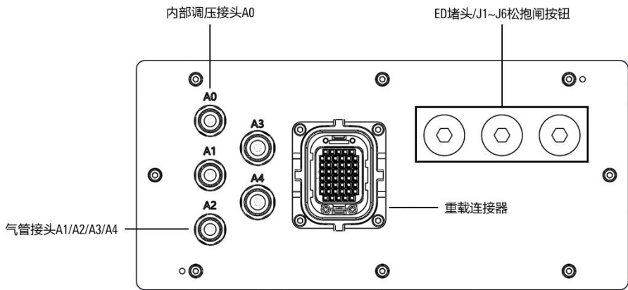
图 5-2 3/4 轴操作机本体底座电气接口
