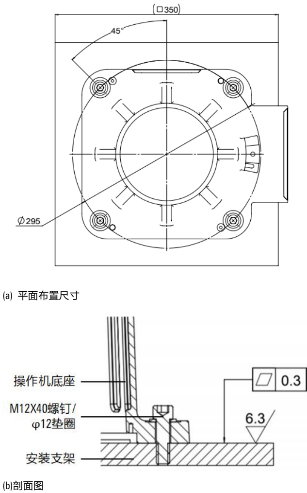
图 4-4 支架固定示意图
