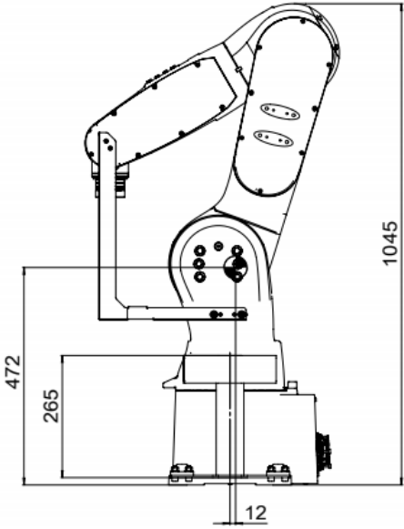
(a) 右视图
