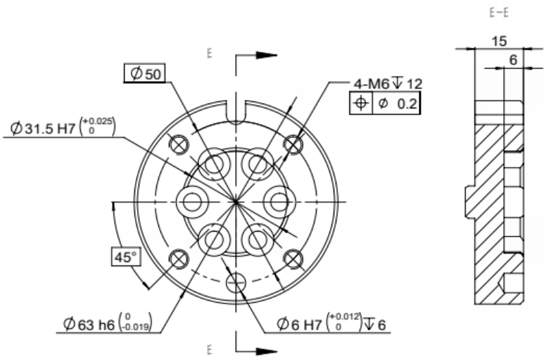
图 7-7 操作机腕部法兰尺寸示意图
