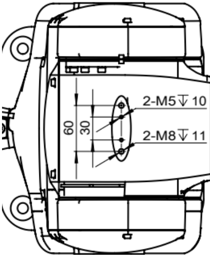
图 7-12 操作机肘部接口尺寸图
