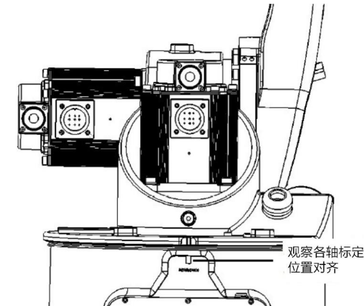
图 8-2 肉眼观察零点标定方式
