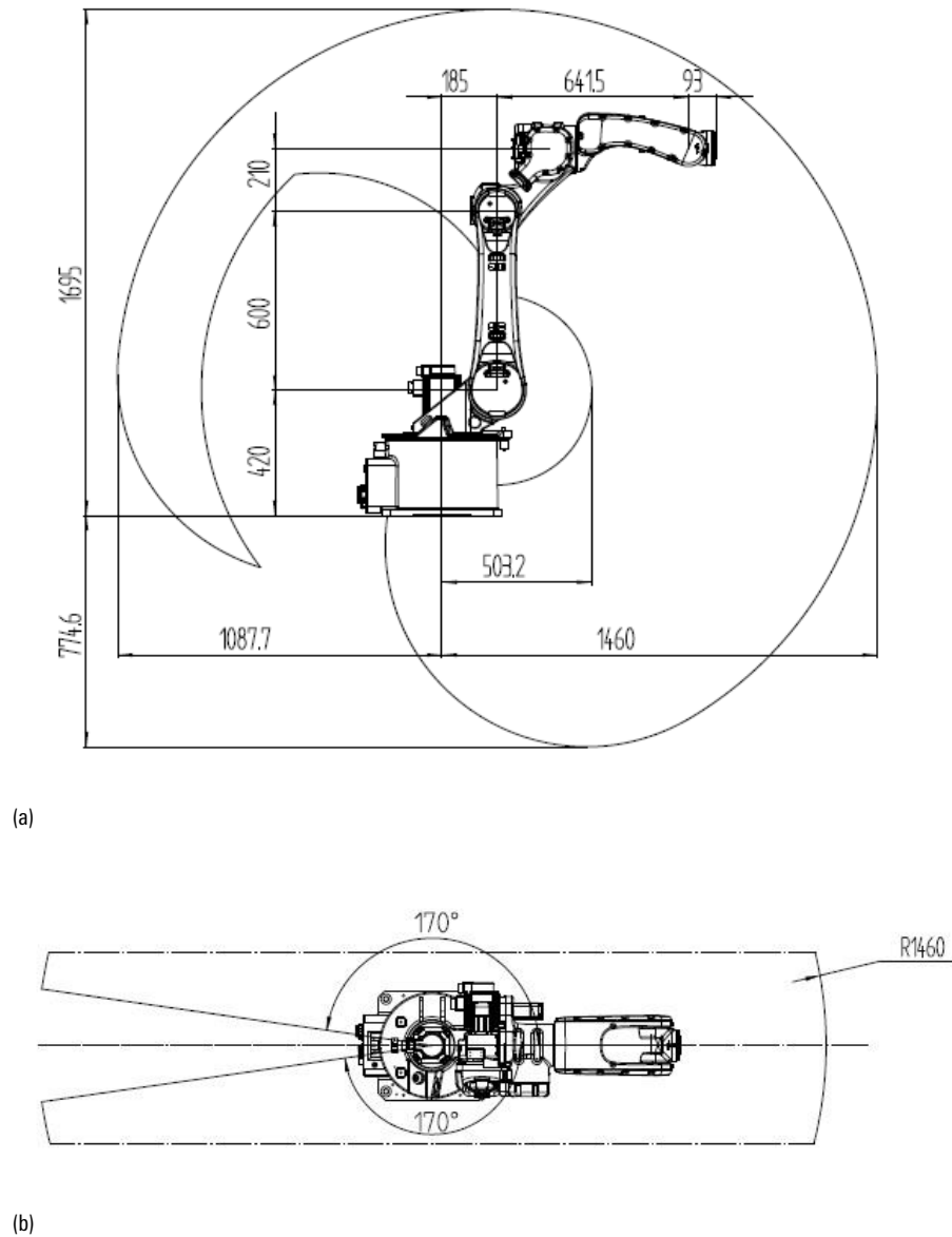
图 7-1 AIR6-1460B-HW 操作机工作范围
