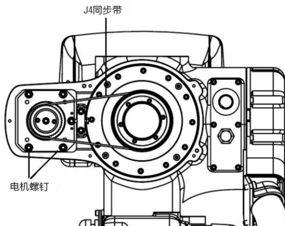
图 11-7 更换 J4 轴同步带示意图
