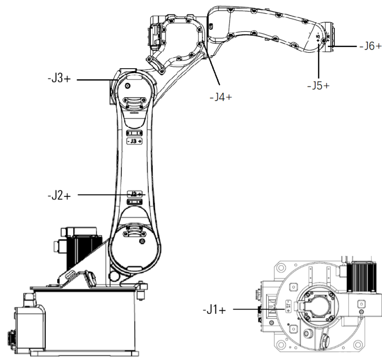
图 2-5 AIR6-1460B-HW 操作机上各轴方向标识
