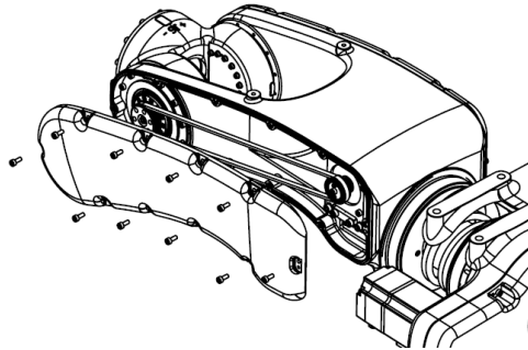
图 11-6 拆除 J6 盖板示意图
