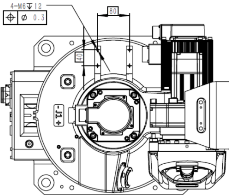
图 7-9 AIR6-1460B-HW 操作机肘部负载接口尺寸示意图
