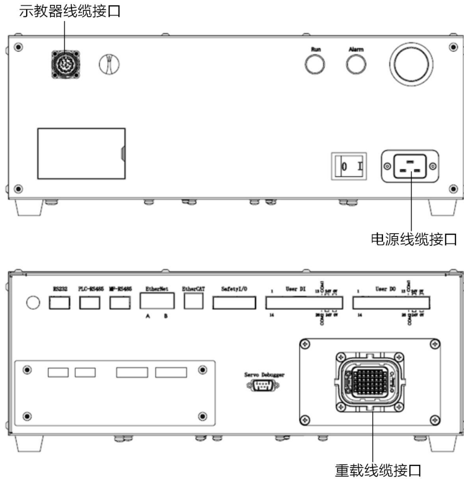
图 6-4 AIR6-1460B-HW 控制柜线缆连接器定义
