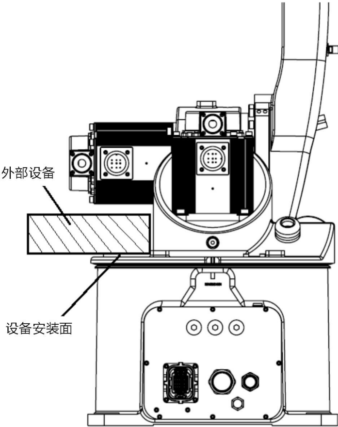
图 7-8 AIR6-1460B-HW 操作机肩部负载安装尺寸示意图
