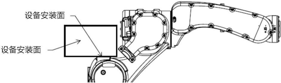
图 7-6 AIR6-1460B-HW 操作机肘部负载安装尺寸示意图
