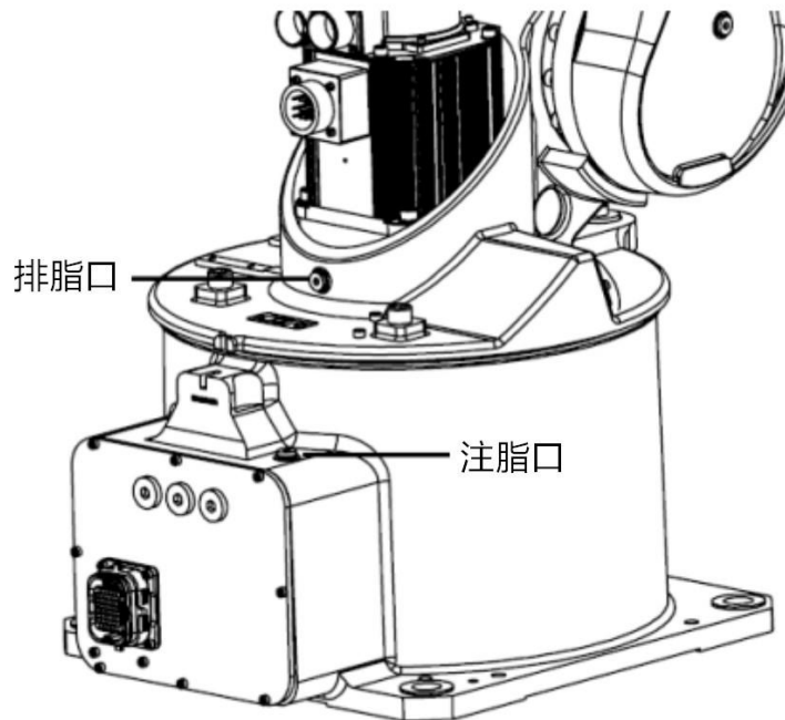
图 11-7 更换 J1 轴减速器润滑脂
