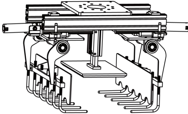
图 6-1 工业机器人用抓手
