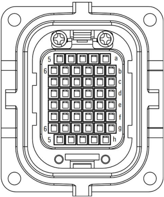
图 5-2 AIR6-1460B-HW 型操作机重载接口示意图
