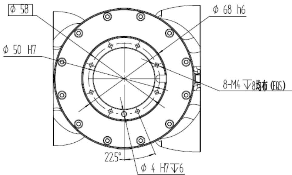
图 7-3 AIR6-1460B-HW 操作机腕部法兰尺寸示意图
