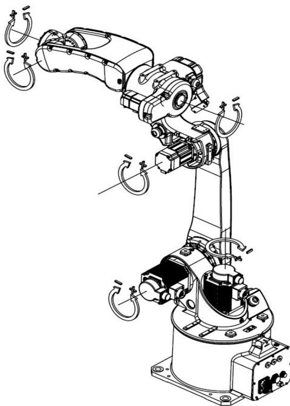
图 8-4 操作机各轴的运动方向
