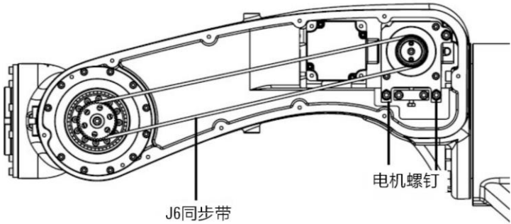
图 11-9 更换 J6 轴同步带示意图
