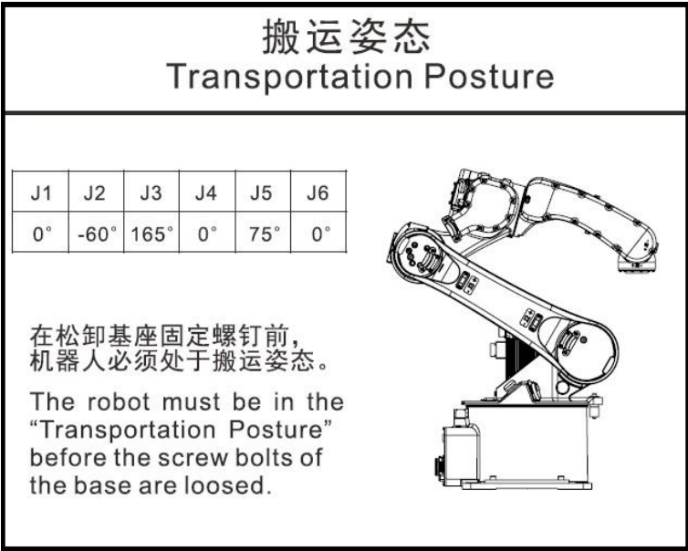
图 2-4 AIR6-1460B-HW 本体各轴搬运姿态标签
