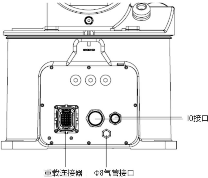
图 5-1 AIR6-1460B-HW 操作机底座上重载连接器接口示意图
