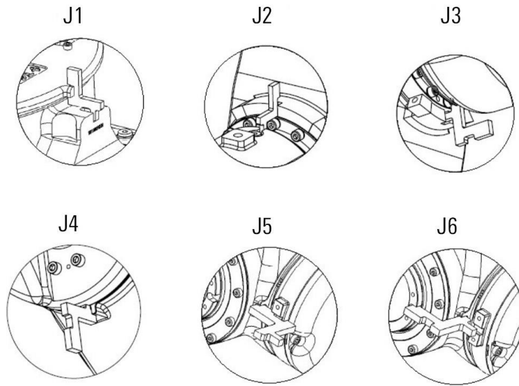
图 8-3 各轴标定块示意图
