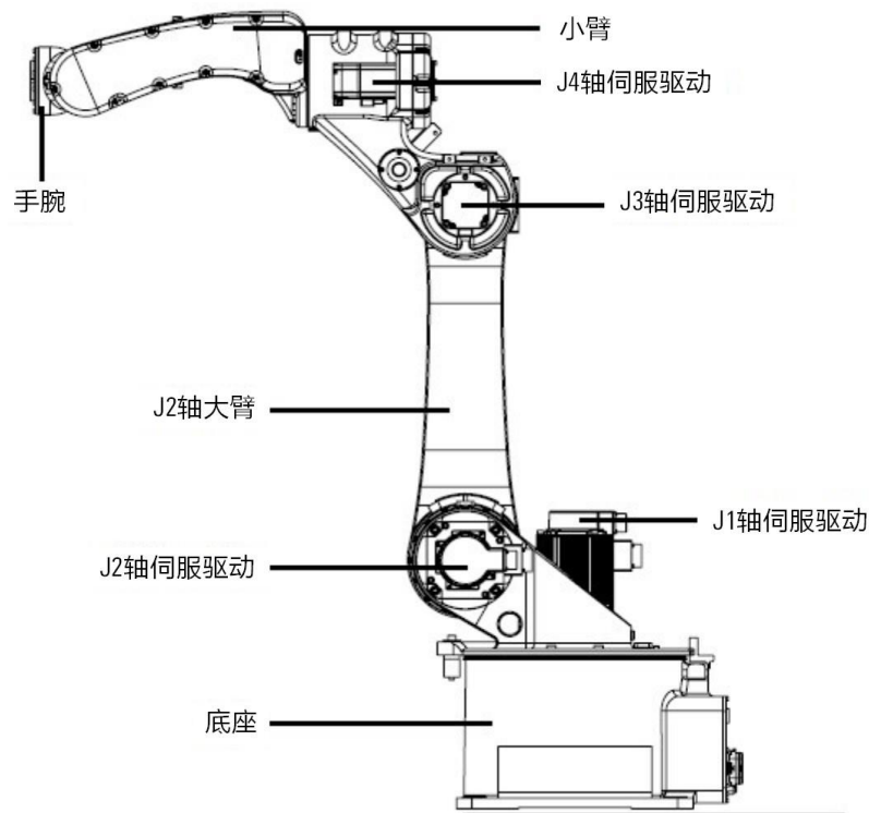
图 1-2 AIR6-1460B-HW 机器人本体及其各个部分
