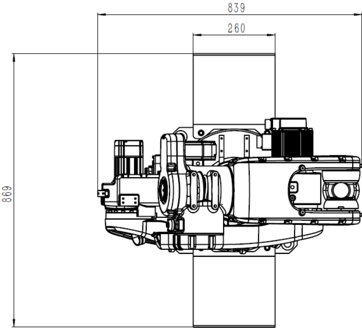
(c) 图 2-8 AIR6-1460B-HW 搬运时操作机各部分尺寸
