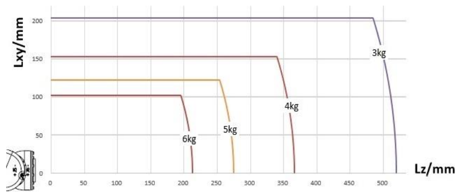
(b) 图 7-5 AIR6-1460B-HW 操作机腕部负载质心位置示意图
