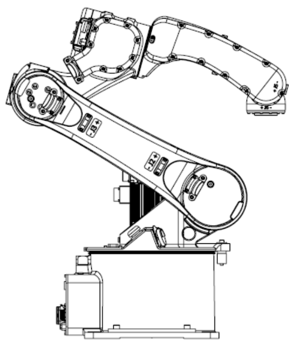
图 2-7 AIR6-1460B-HW 操作机搬运位姿图
