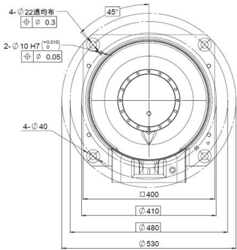
图 4-1 AIR6-1460B-HW 操作机底座接口尺寸
