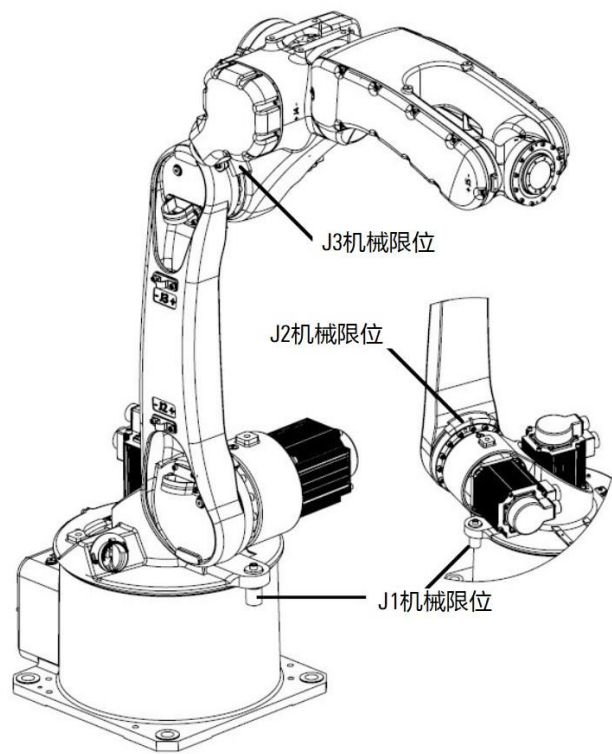
图 7-2 AIR6-1460B-HW 操作机上机械式制动器
