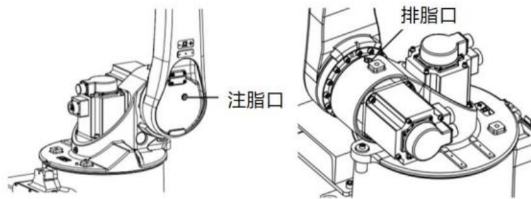
图 11-8 更换 J1 轴减速器润滑脂
