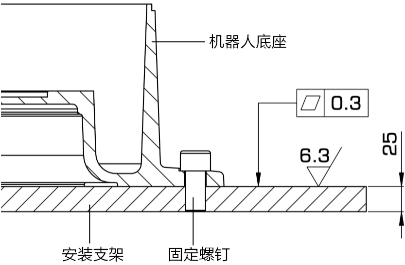
(b) 图 4-3 操作机支架固定示意图
