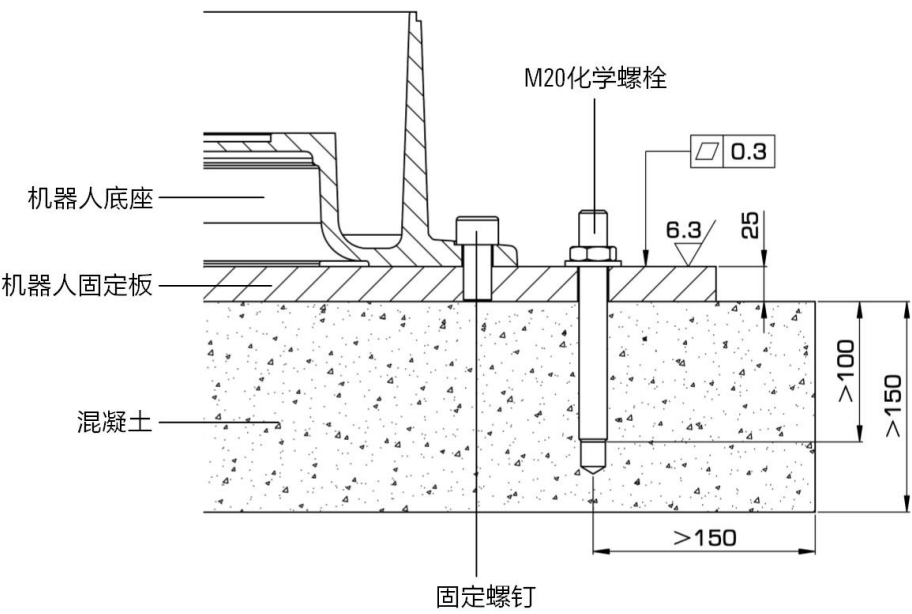
(b) 图 4-2 操作机地面固定示意图
