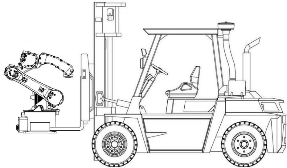
图 2-9 AIR6-1460B-HW 叉车搬运示意图
