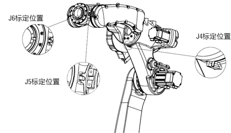
(b) 图 8-1 AIR6-1460B-HW 各轴零点示意图
