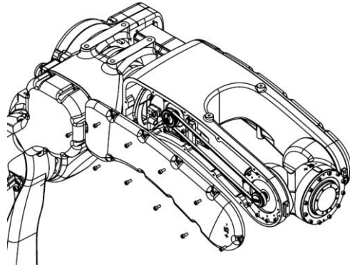
图 11-5 拆除 J5 盖板示意图
