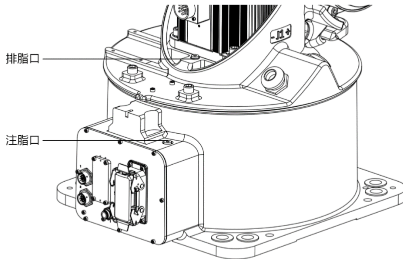
图 12-6 AIR25-1700C 更换 J1 轴减速器润滑脂
