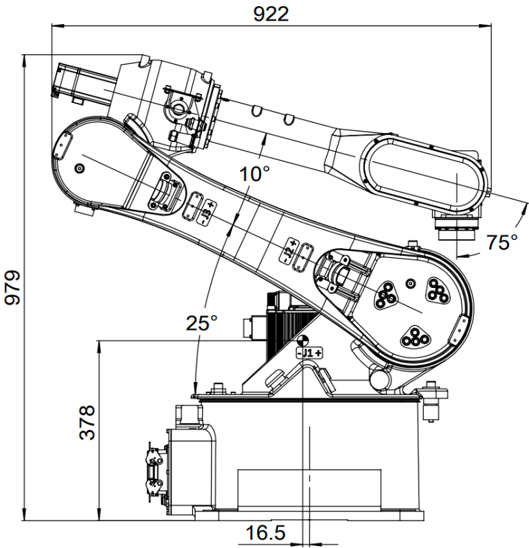
图 9-3 AIR25-1700C 系列 操作机搬运位姿图
