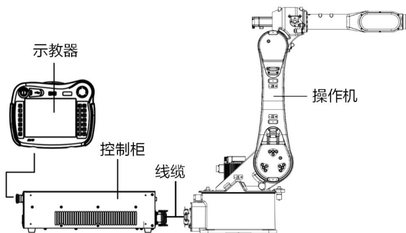
图 1-1 AIR25-1700C 机器人系统的构成
