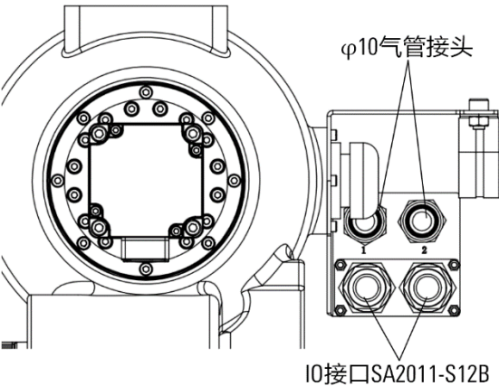
图 5-1 操作机小臂接口示意图
