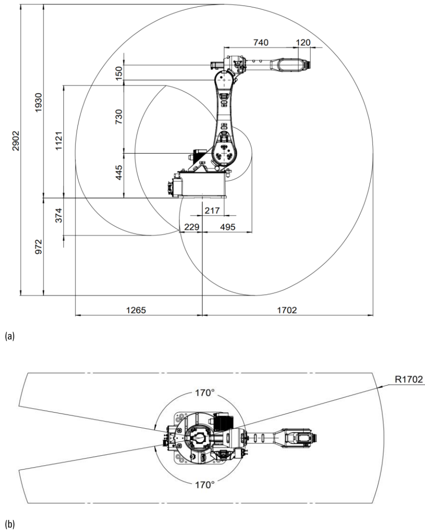
图 7-1 AIR25-1700C 系列操作机工作范围
