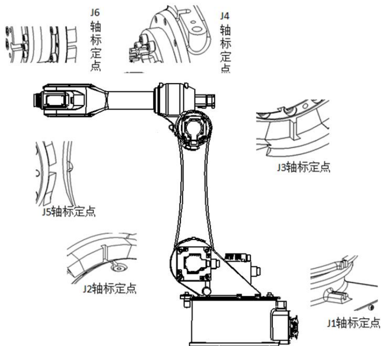
图 8-1 AIR25-1700C 系列各轴零点示意图
