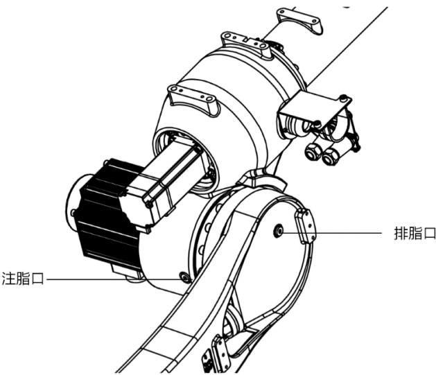
图 12-8 AIR25-1700C 更换 J3 轴减速器润滑脂
