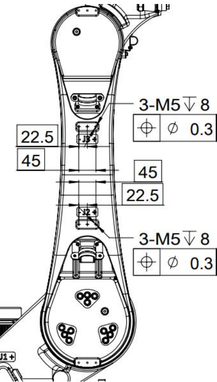
图 7-9 大臂接口尺寸图
