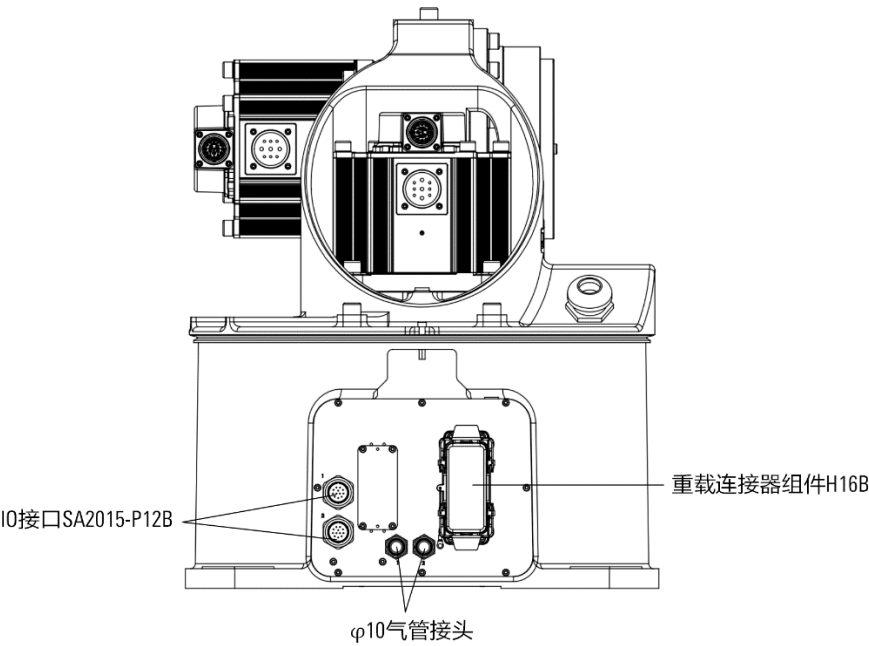
图 5-2 操作机底座接口示意图
