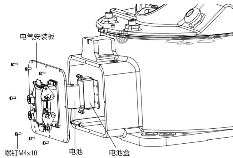
图 12-5 AIR25-1700C 拆卸操作机电器安装面板
