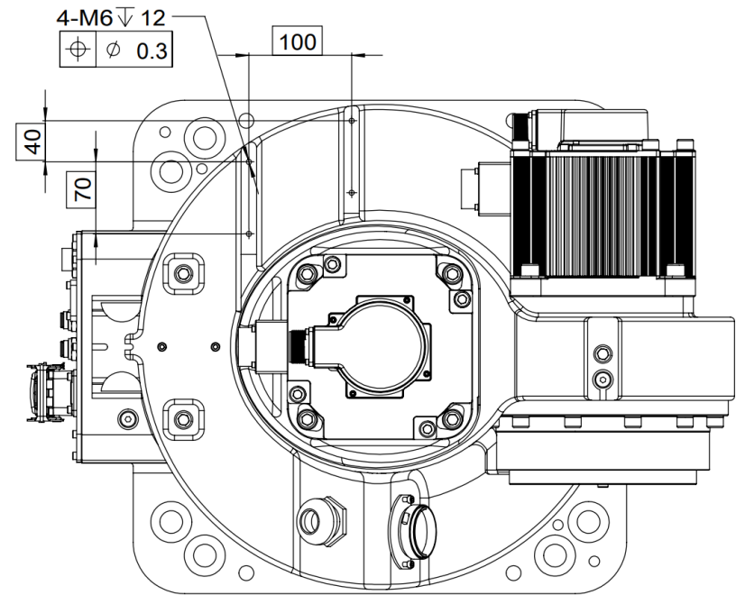
图 7-8 肩部接口尺寸图
