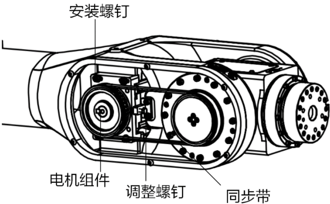
图 12-10 拆卸同步带
