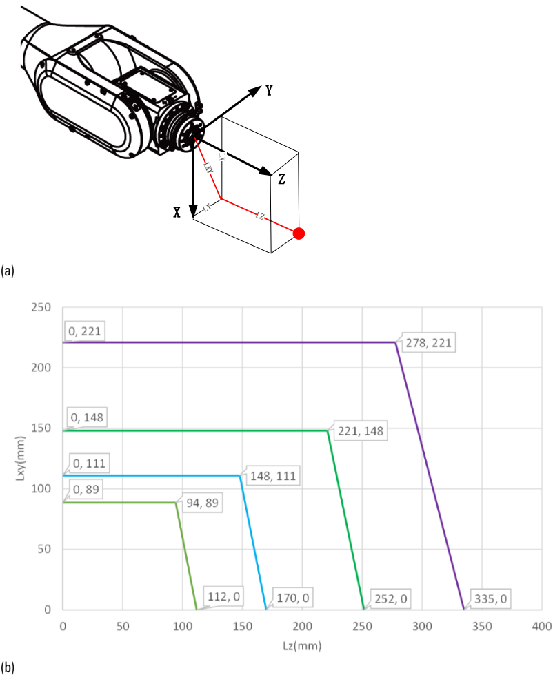
图 7-5 AIR25-1700C 系列腕部负载质心位置示意图
