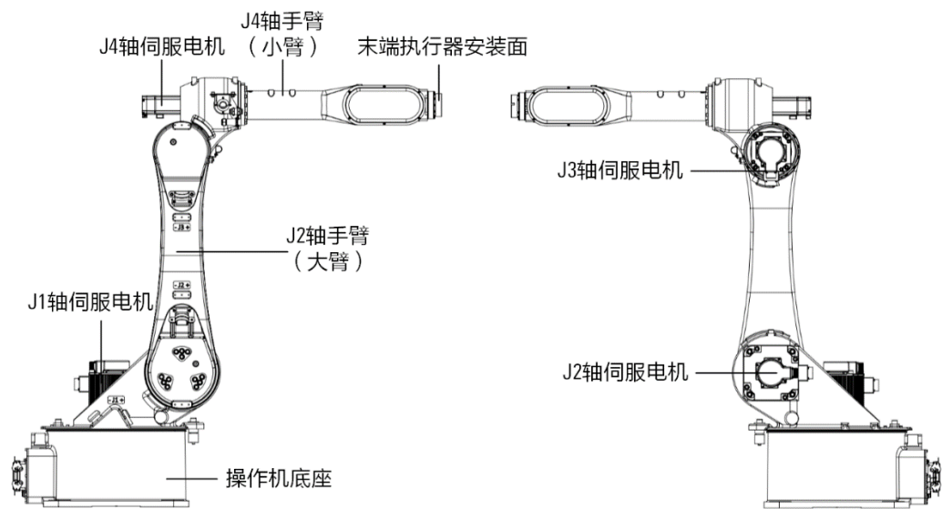
图 1-2 AIR25-1700C 系列机器人本体及其各个部分
