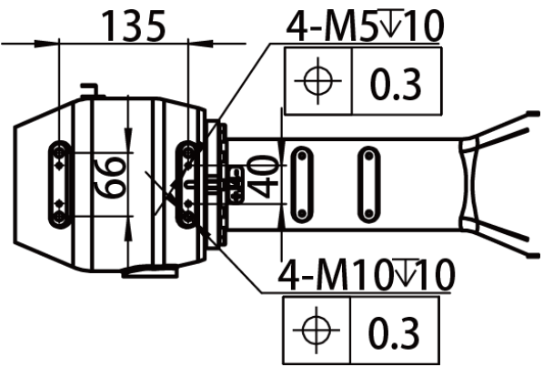
图 7-6 肘部负载接口尺寸示意图
