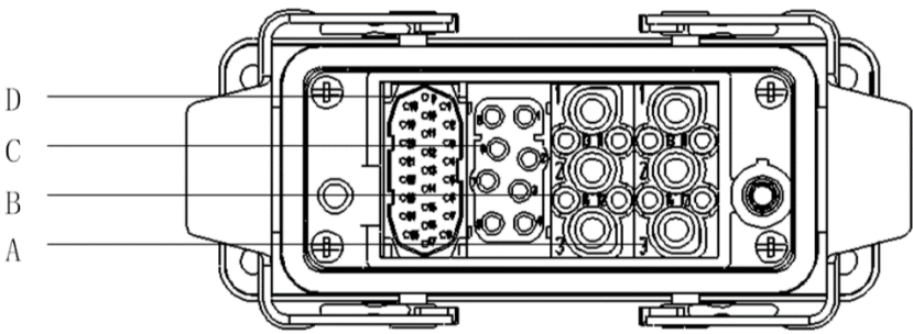
图 5-3 AIR25-1700C 操作机本体上重载连接器
