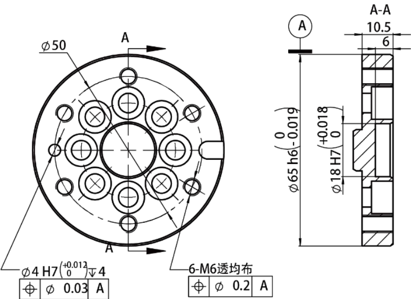
图 7-3 腕部法兰尺寸示意图
