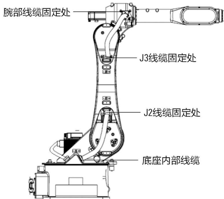
图 12-1 操作机线缆布局图
