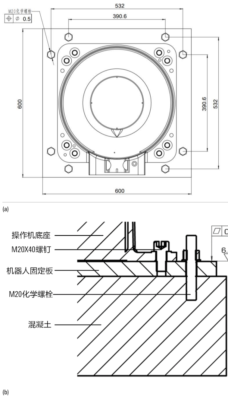
图 4-3 操作机吊装示意图
