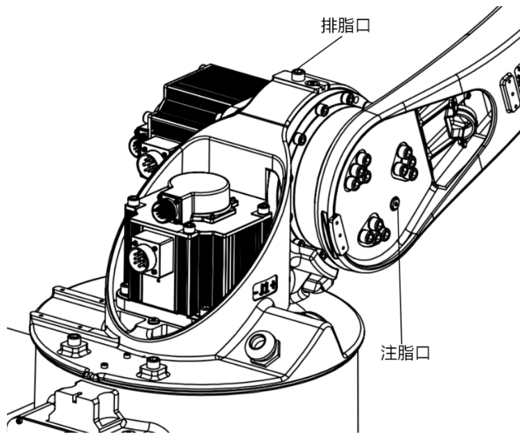
图 12-7 AIR25-1700C 更换 J2 轴减速器润滑脂
