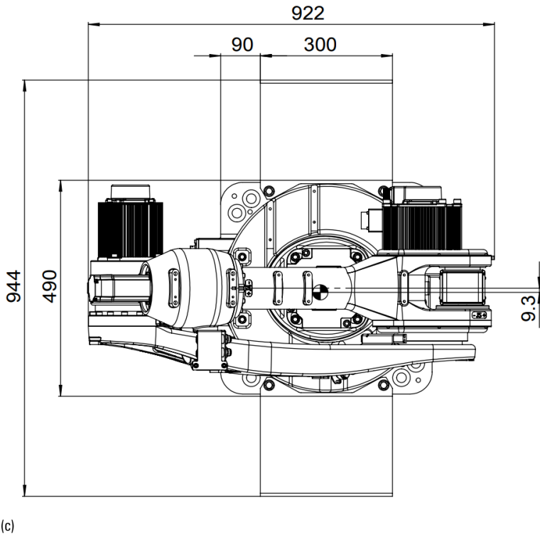
图 9-2 AIR25-1700C 系列搬运时操作机尺寸
