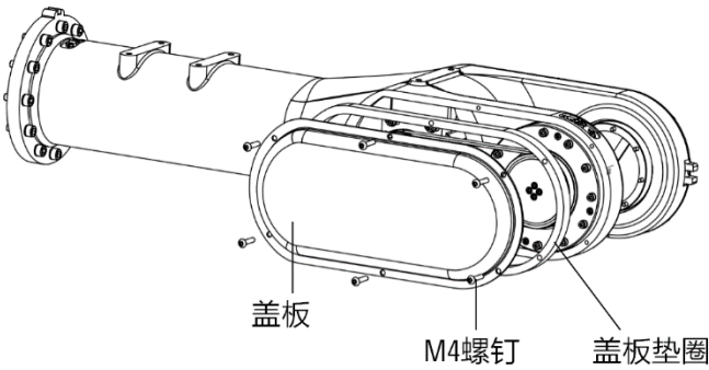
图 12-9 拆卸盖板
