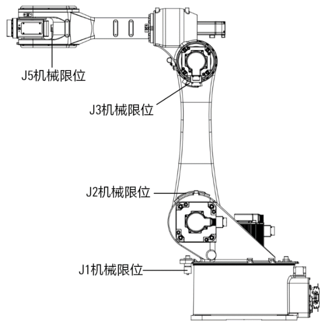
图 7-2 操作机上机械式制动器
