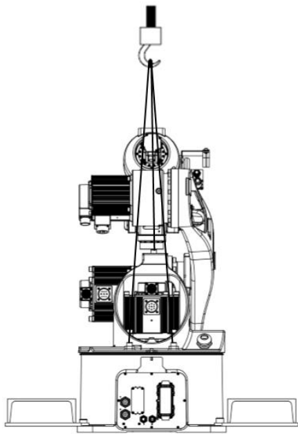
图 9-5 AIR25-1700C 系列吊环搬运示意图
