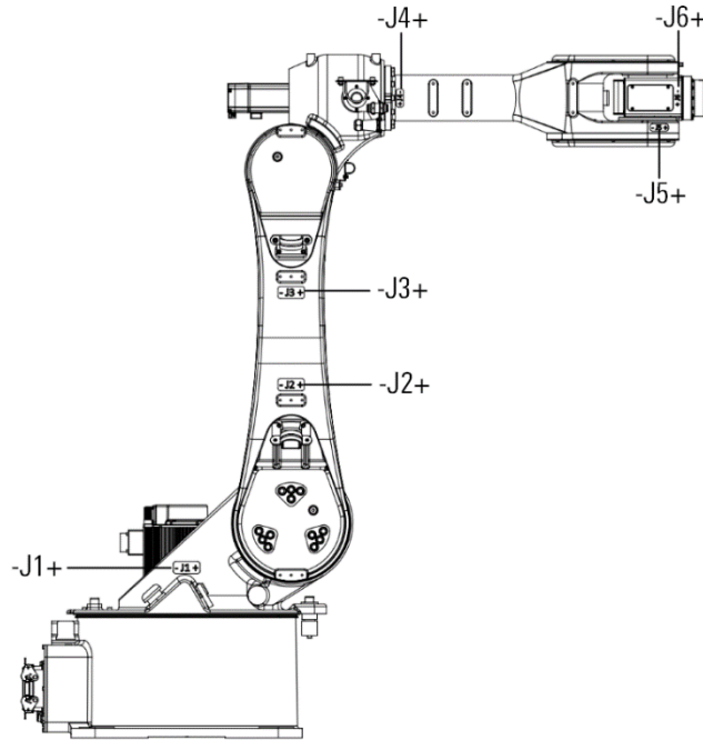
图 2-3 AIR25-1700C 操作机上各轴方向标识
