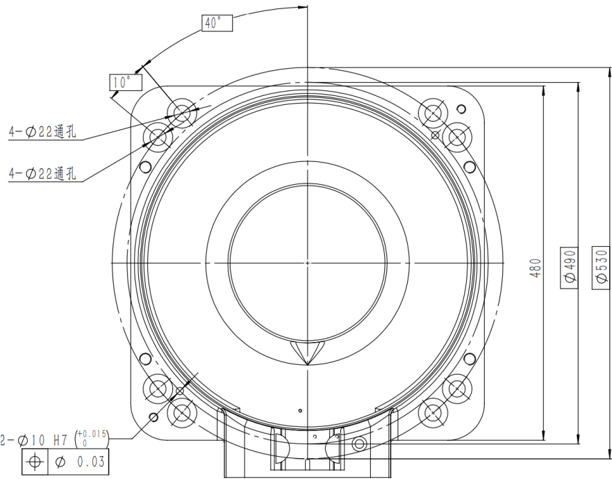
图 4-1 操作机基座接口尺寸
