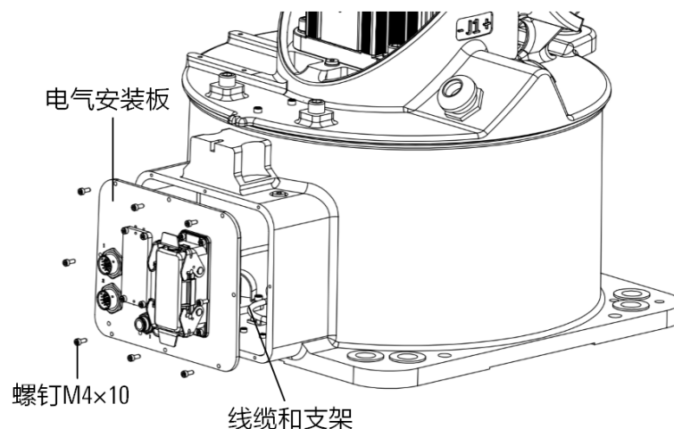
图 12-2 AIR25-1700C 底座内部线缆
