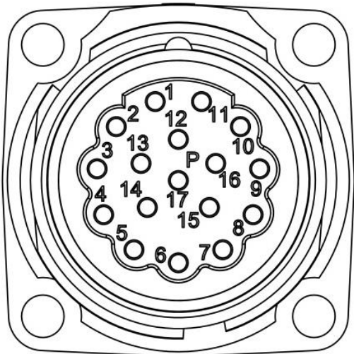
图 5-4 示教器接口
