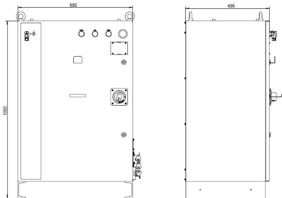
图 3-1 控制柜外观
