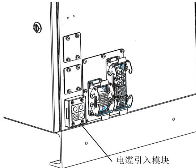
图 6-1 电缆引入模块示意图
