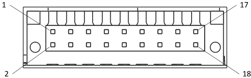
图 6-4 Safety IO 接口引脚标识图
