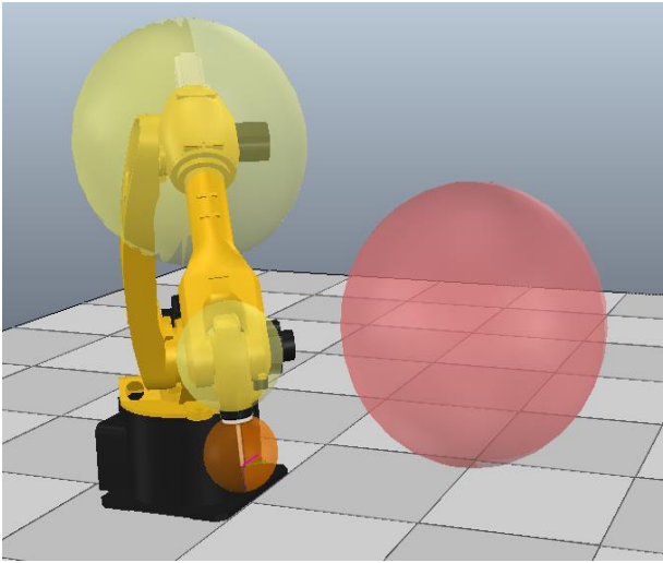
图 6-79 机器人的“轴包络”和“工具包络”边界在禁止区域外
