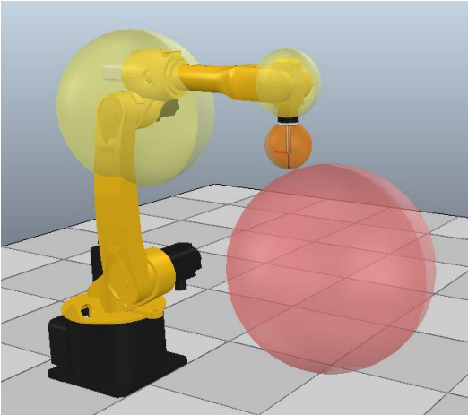
图 6-76 禁止区域使用实例所用模型示意图
