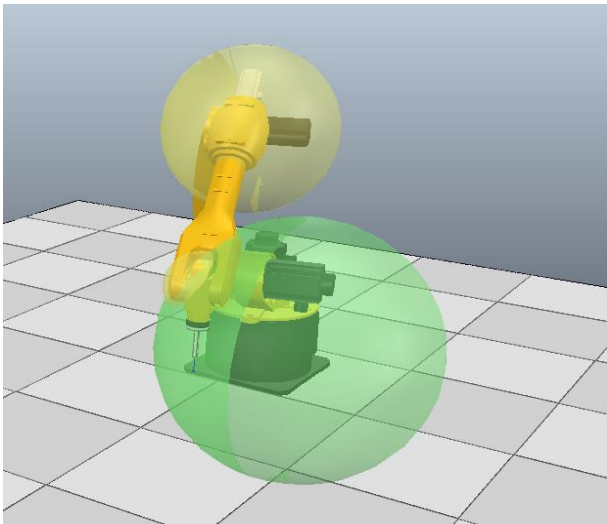
图 6-72 机器人的 5 轴“轴包络”离开工作区域
