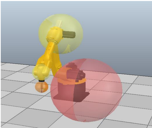
图 6-80 机器人的 5 轴“轴包络”进入停止缓冲区
