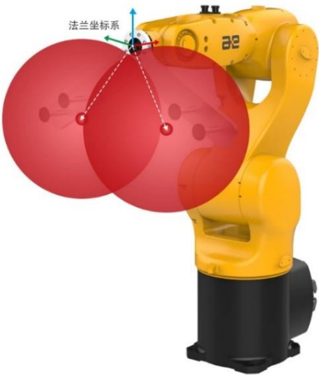
图 6-46 法兰坐标系为参考坐标系时包络球心位置示意
