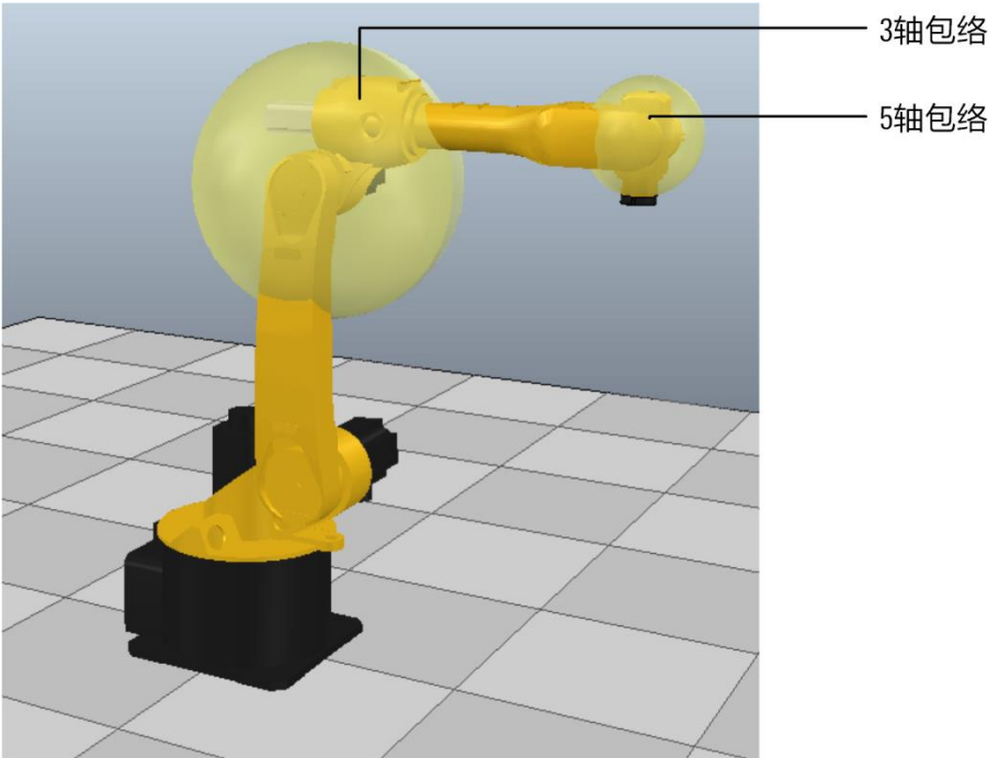
图 6-49 机器人 3 轴及 5 轴包络示意图
