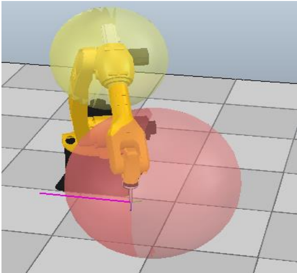
图 6-81 机器人位于停止缓冲区或禁止区域时
