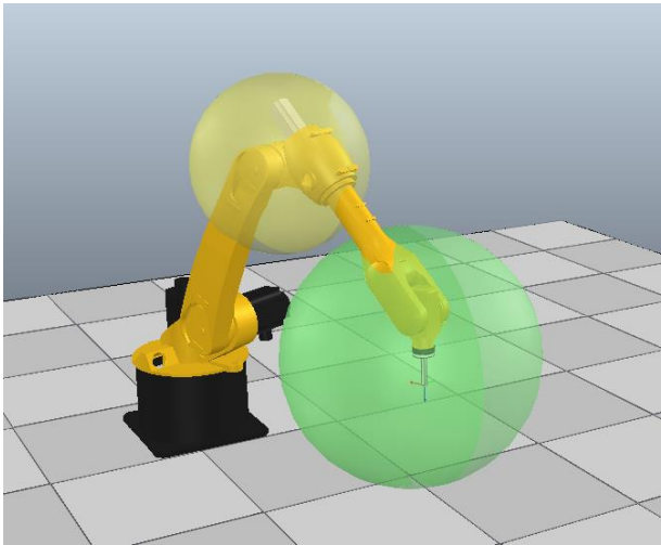
图 6-71 机器人的 5 轴“轴包络”和“工具包络”在工作区域中
