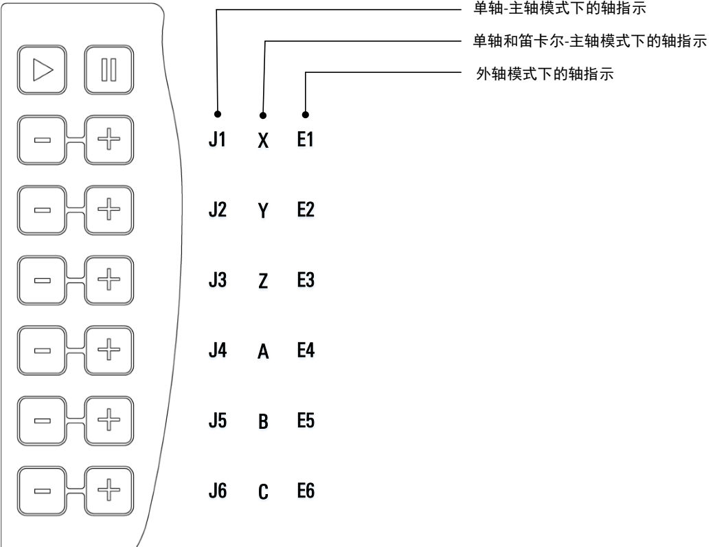
图 2-11 示教器控制键
