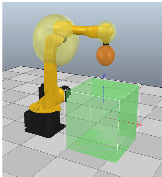
图 6-55 长方体工作区域的工况示意图
