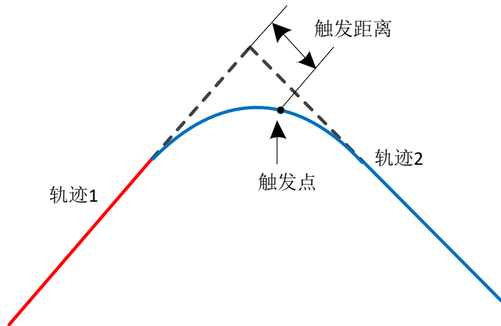
图 7-1 轨迹触发
