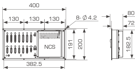
安装尺寸图
