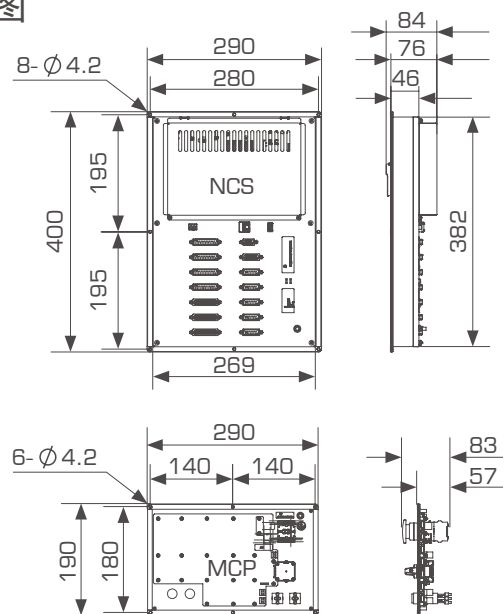
AE8100-AMV/CM 安装尺寸图
