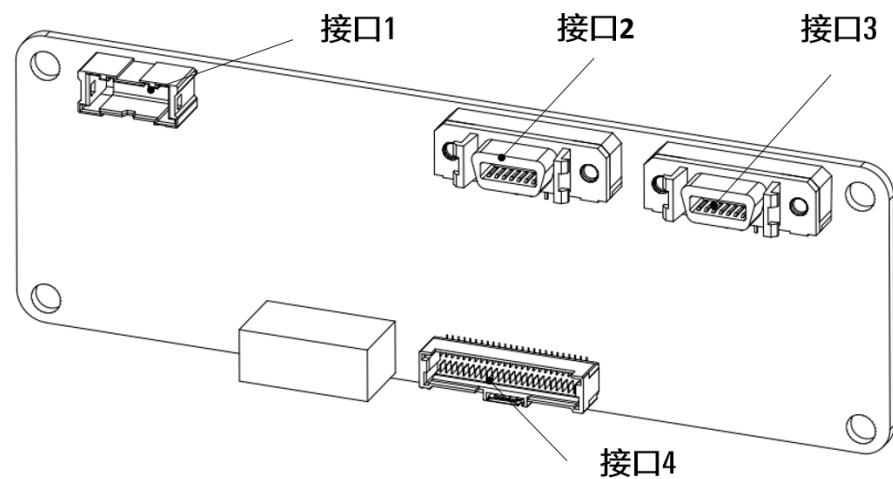
图 21-36 MCB-IEB 接口示意图
