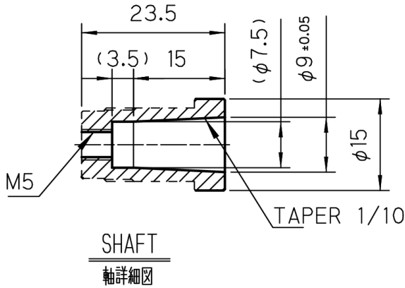
(b) 编码器对外连接孔剖面图
