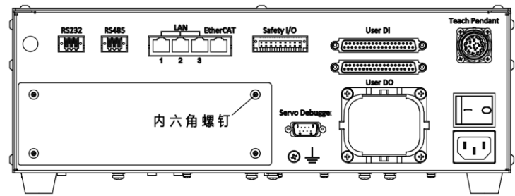
图 21-16 控制柜后面板示意图
