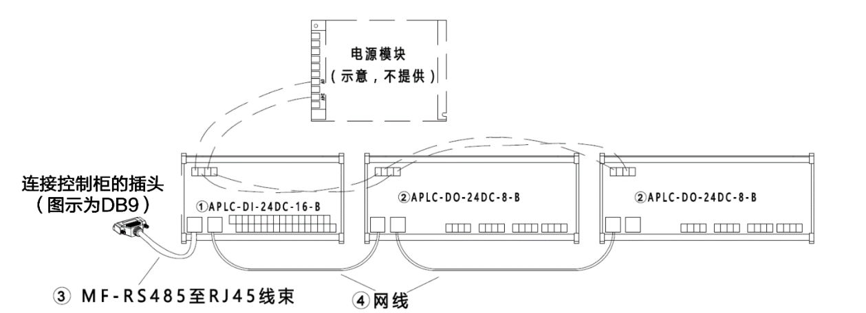
图 20-14 “16 路 DI+16 路 DO” 的连接示意图
