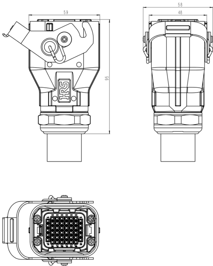
图 9-27 inCube20/2S 重载接头尺寸
