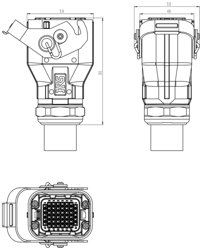
图 9-23 inCube20/2S 重载接头尺寸
