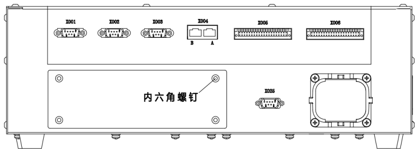
图 21-4 控制柜后面板示意图
