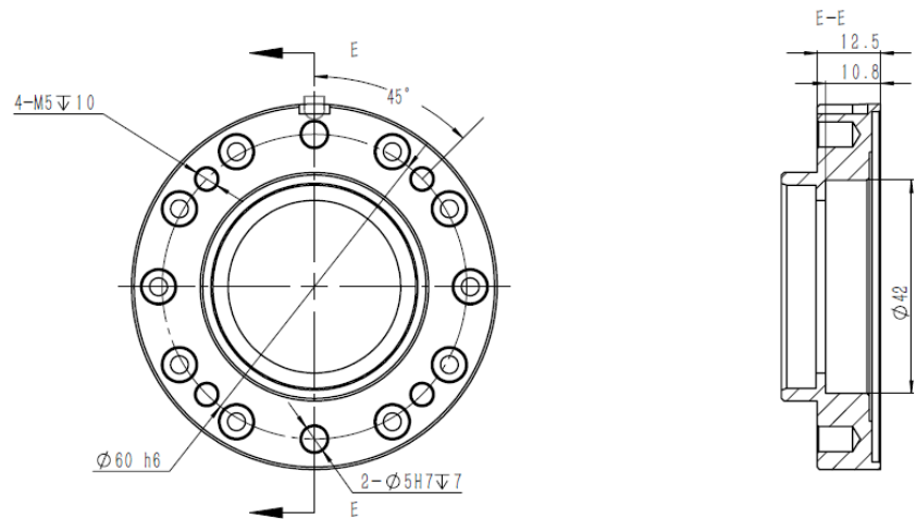
图 7-5 AIR10-1210C(-HW) 操作机腕部法兰尺寸示意图
