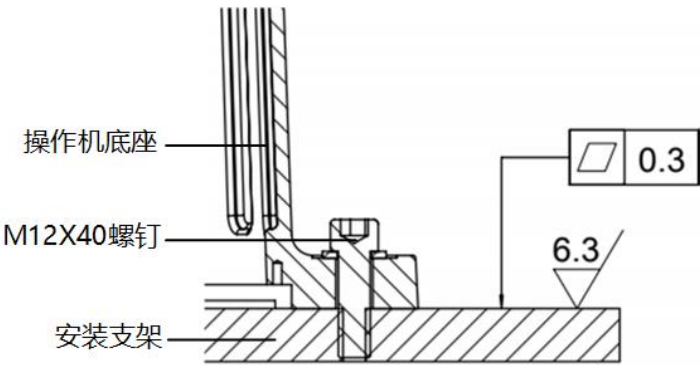
(b)剖面图
