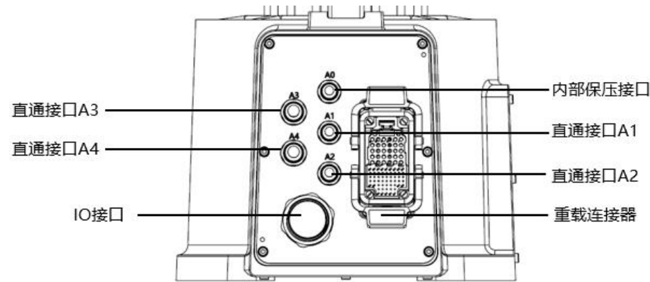
图 5-1 操作机本体底座电气接口
