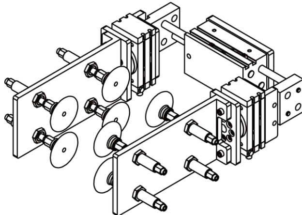
图 6-2 工业机器人用吸盘
