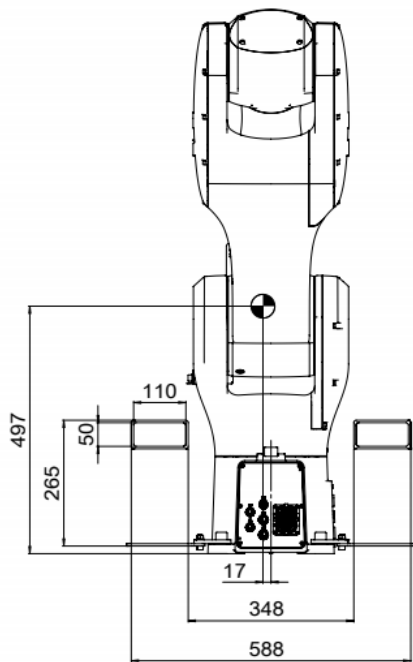
(b) 后视图
