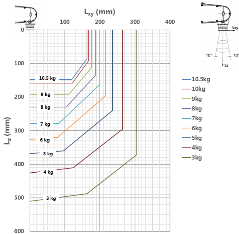
图 7-8 AIR10-1210C(-HW)操作机腕部向下时的负载质心位置示意图
