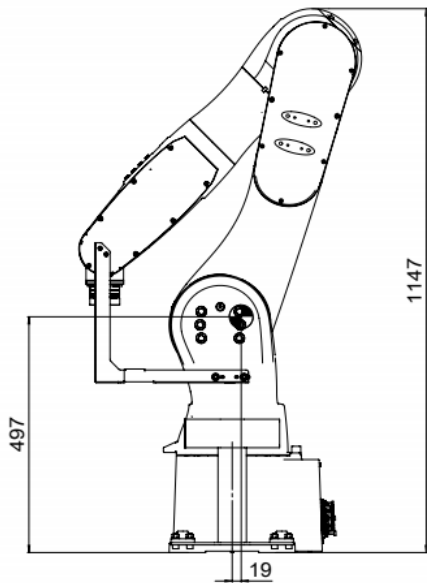
(a) 右视图
