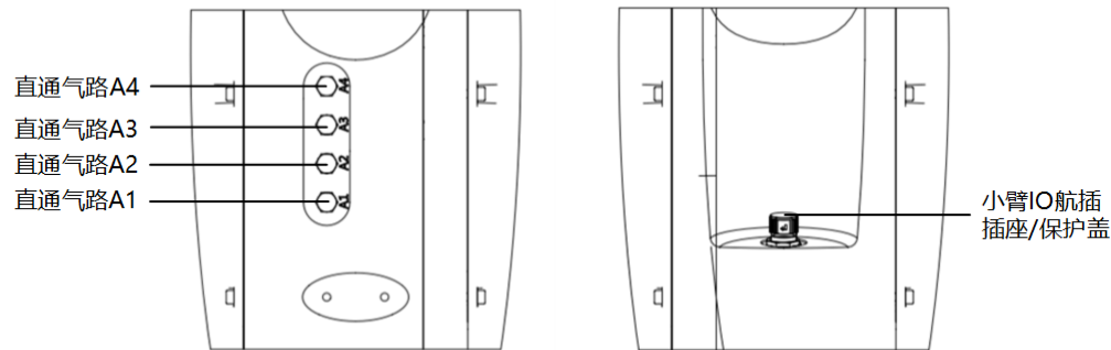
图 5-2 AIR10-1210C 操作机小臂上接口
