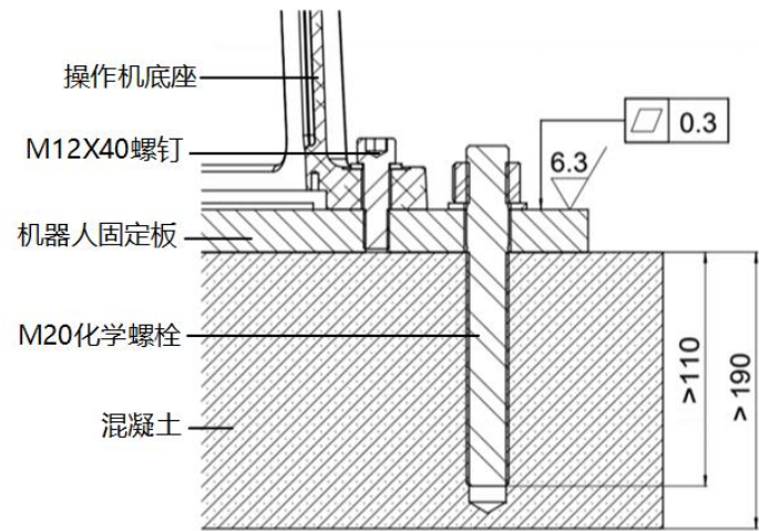
(b) 剖面图
