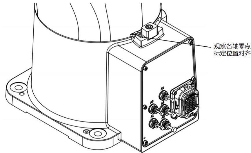
图 8-2 肉眼观察零点标定方式
