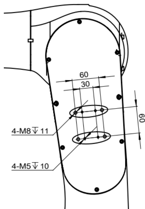
图 7-12 操作机大臂接口尺寸图
