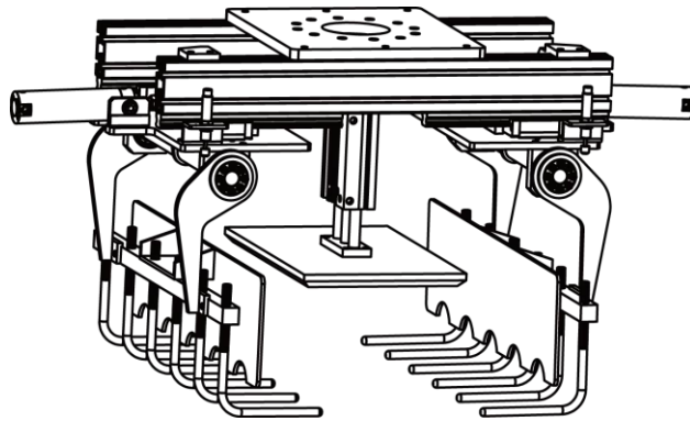
图 6-1 工业机器人用抓手
