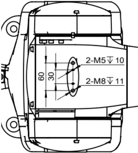
图 7-11 操作机肘部接口尺寸图
